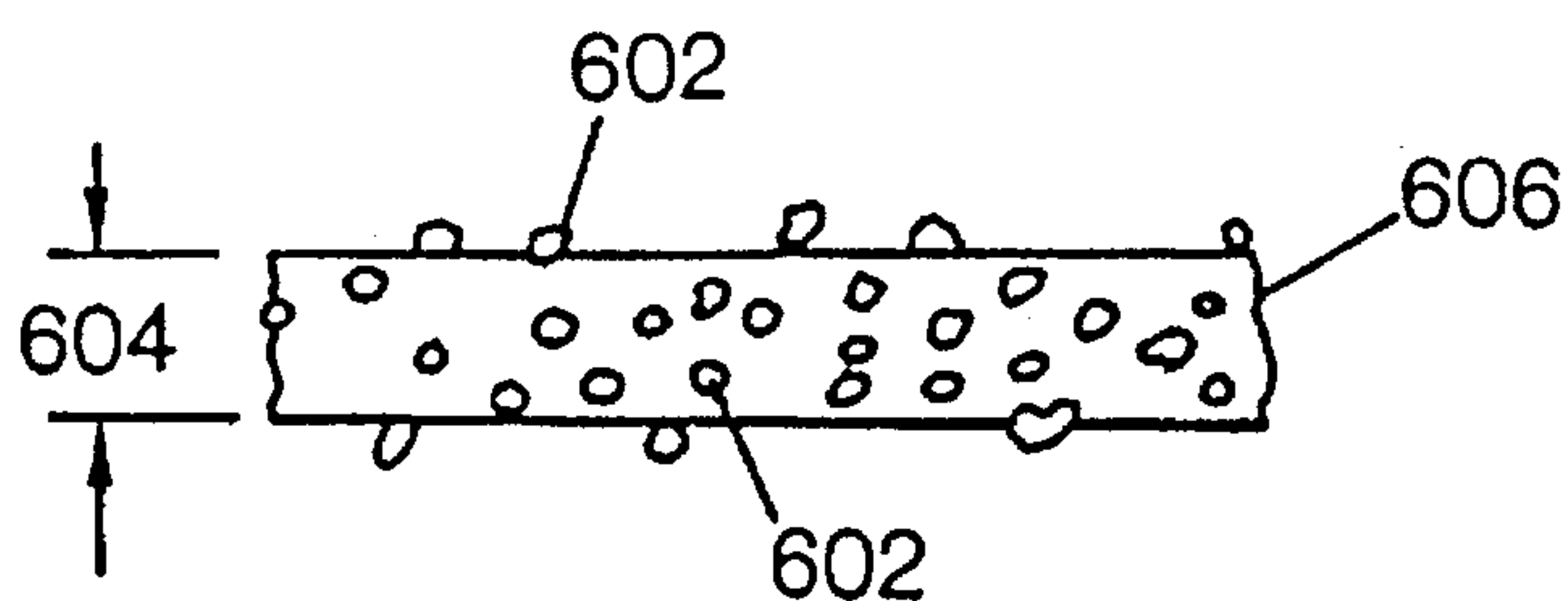
FIG. 12
