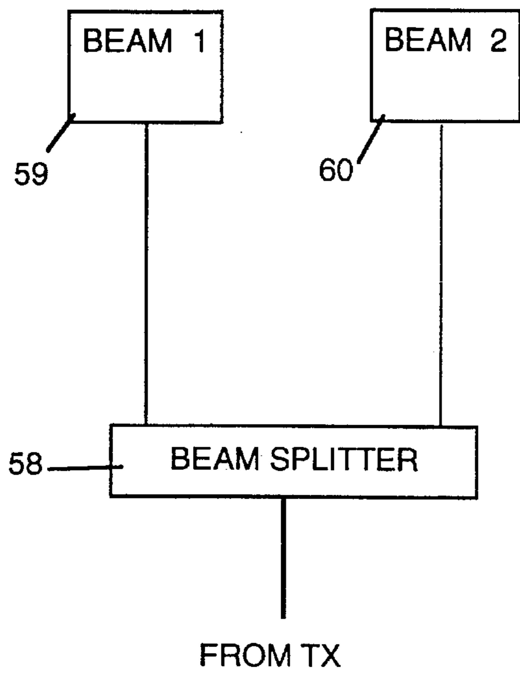
Fig. 14 (a) INPHASE
