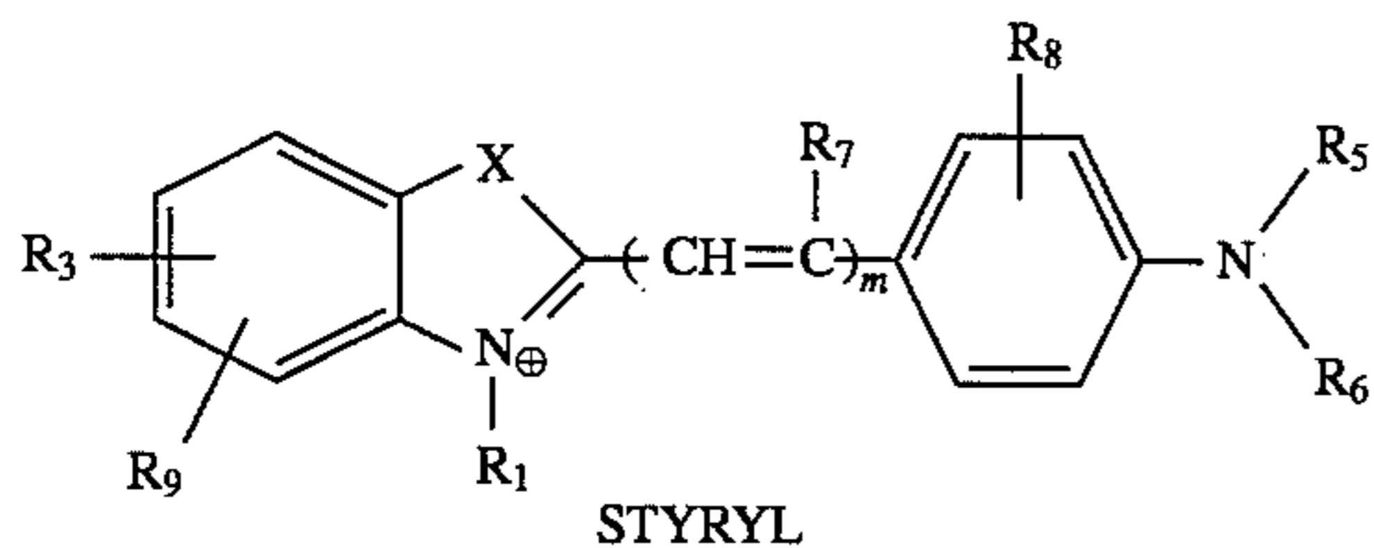
STYRYL
