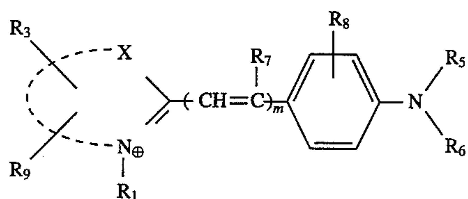
STYRYL
