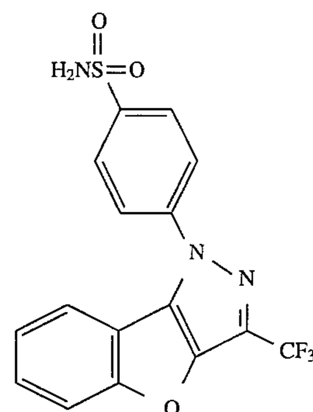
4-[3-(Trifluoromethyl)-1H-benzofuro[3,2-c]pyrazol-1-yl]benzenesulfonamide
