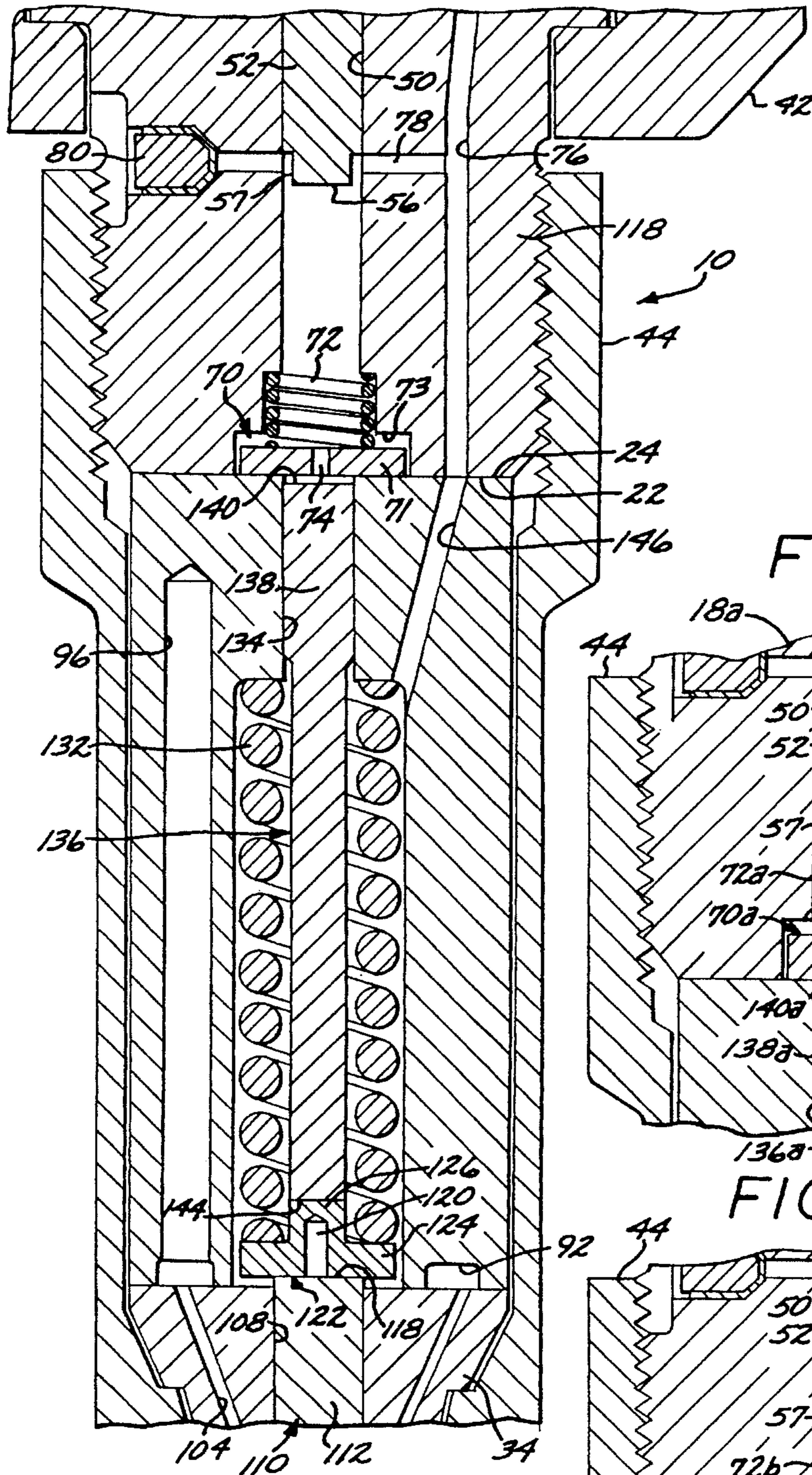
FIG. 8
