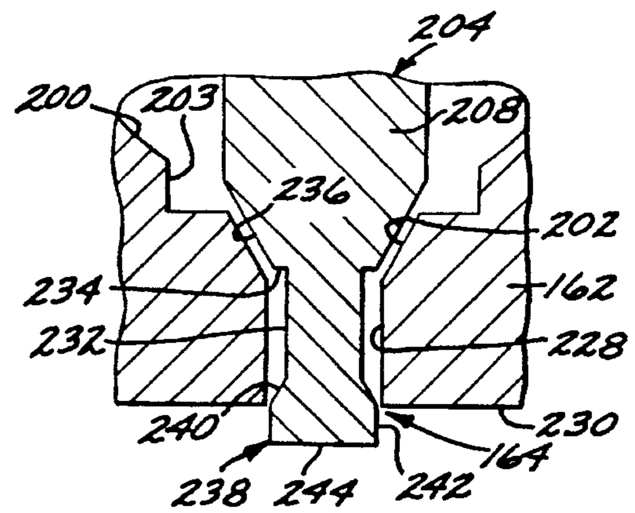
FIG. 16
