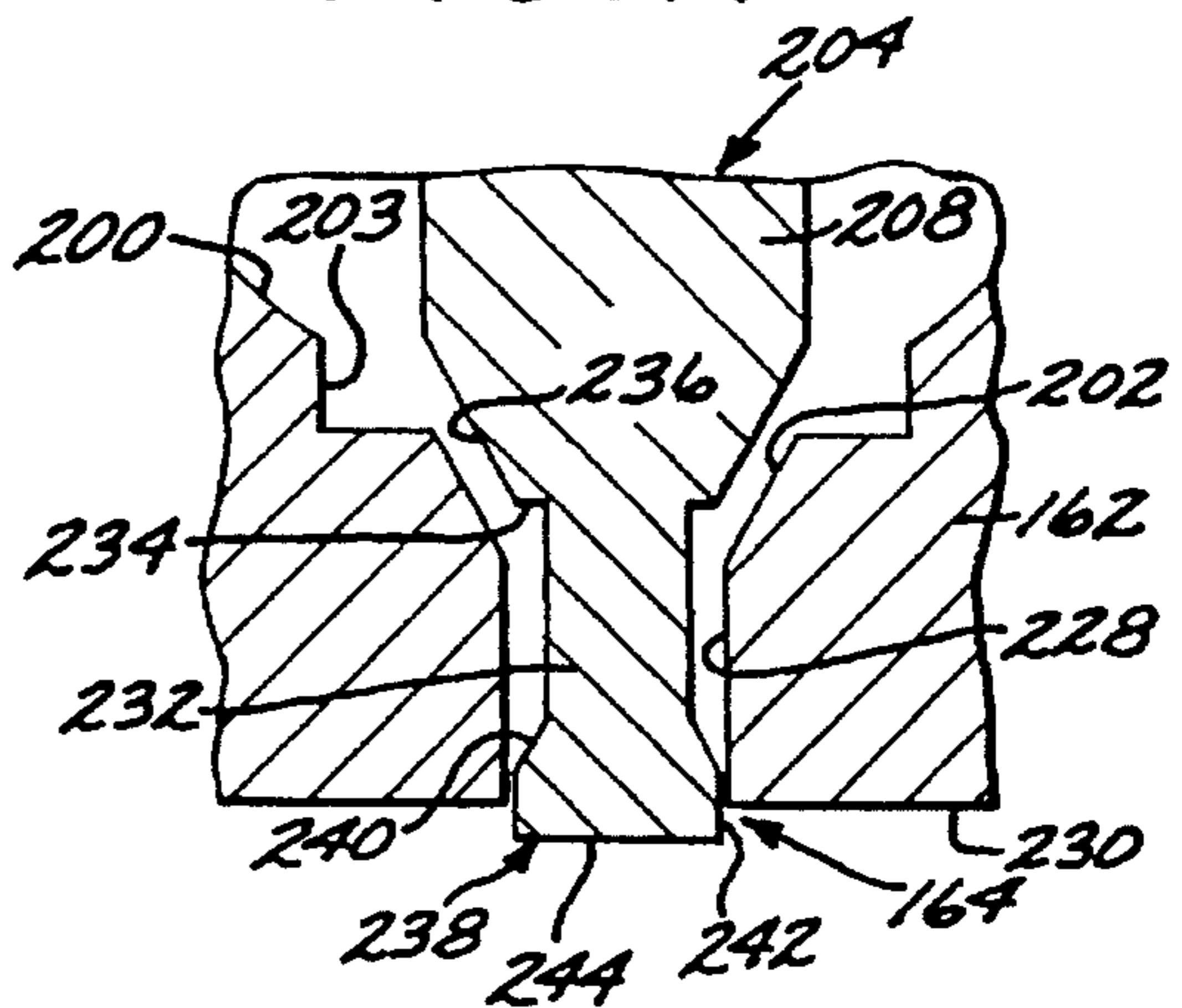
FIG. 17
