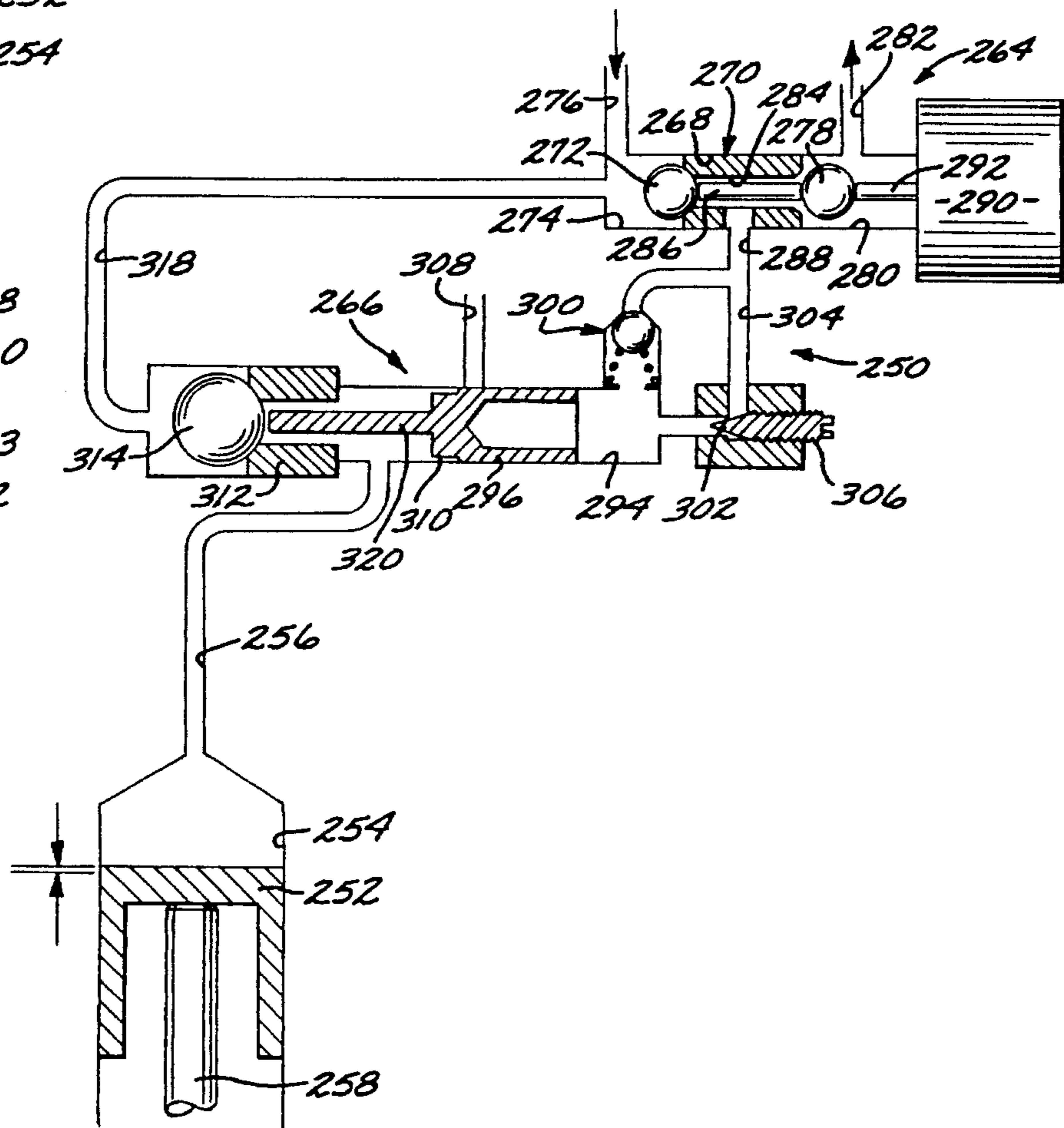
FIG. 19
