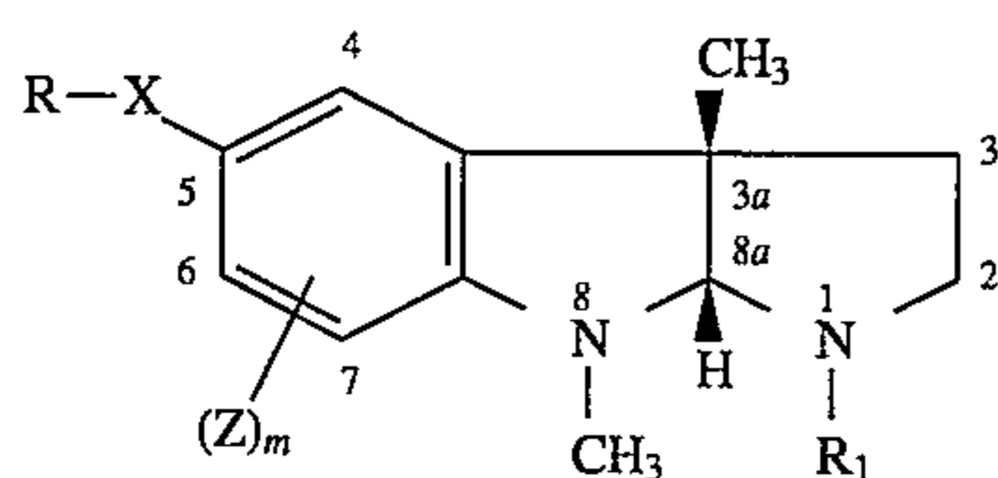
3aS-cis
