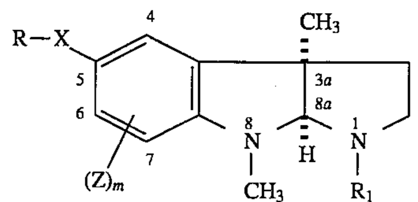
3aR-cis
