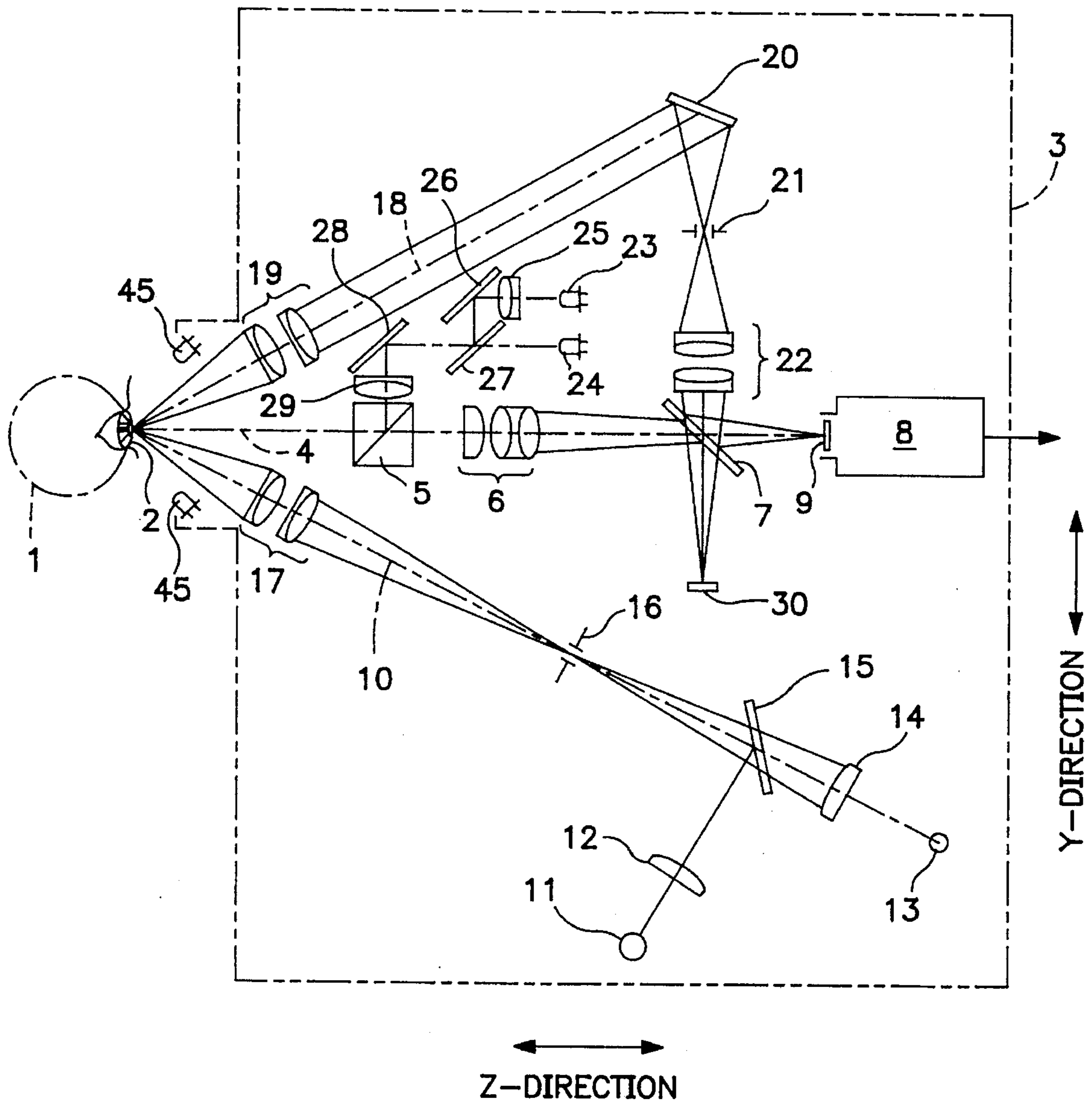
FIG. 6
