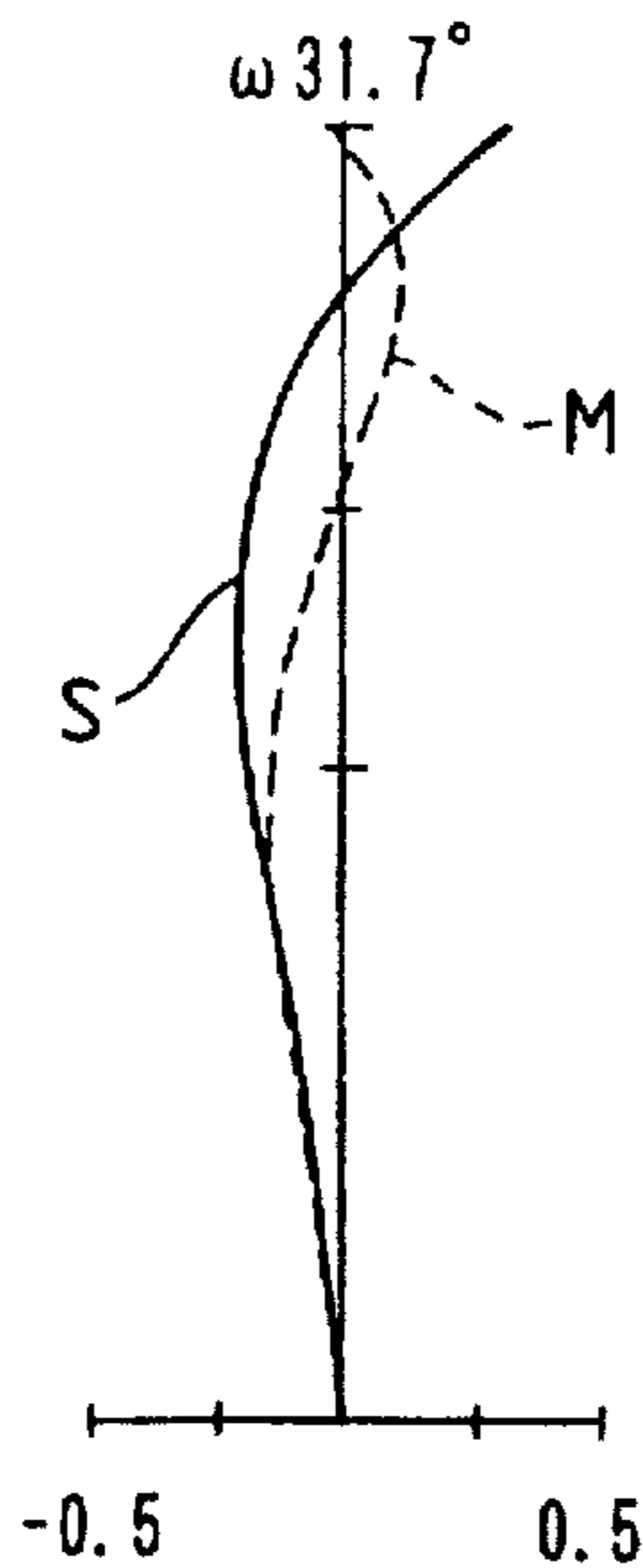
FIG. 8B ASTIGMATISM
