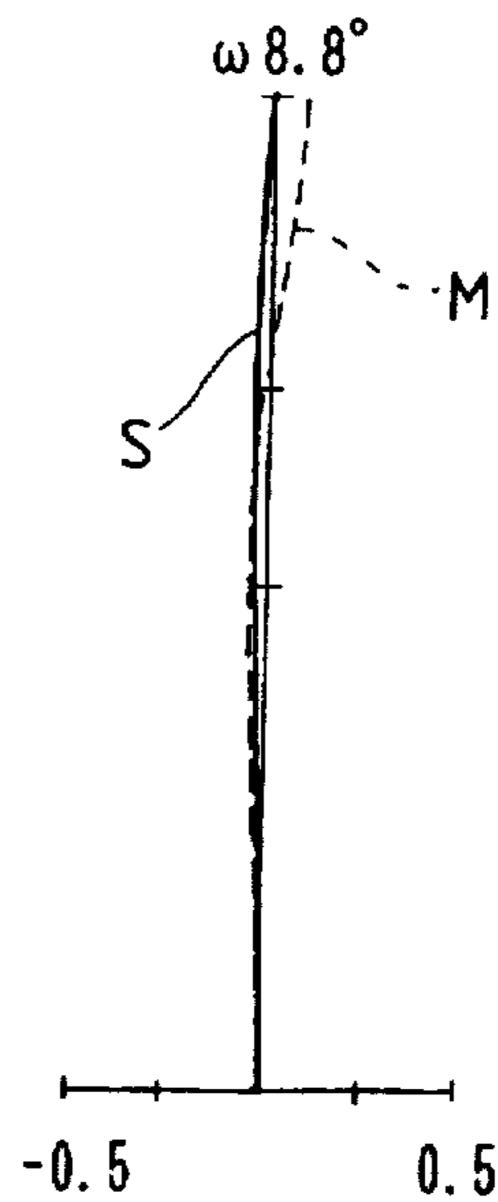
FIG. 7B ASTIGMATISM
