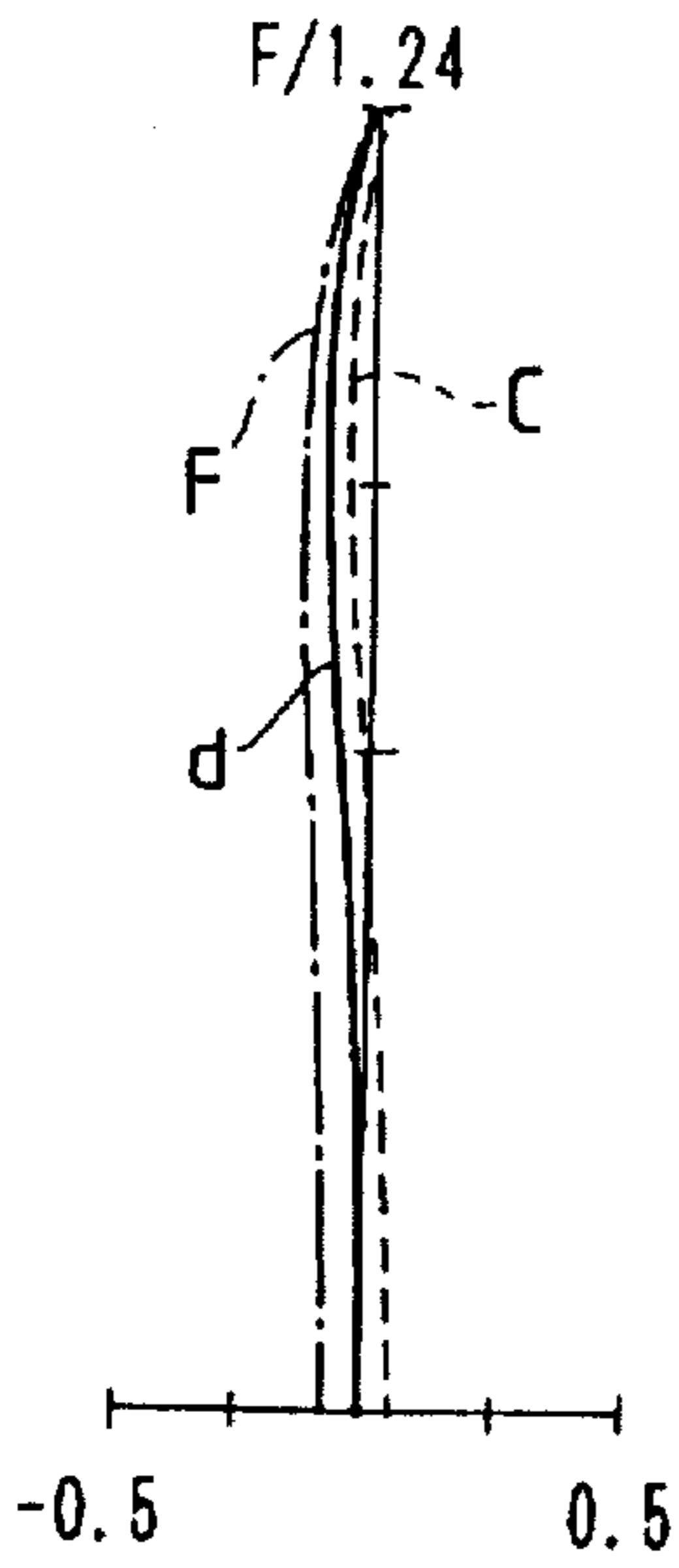
FIG. 9A SPHERICAL ABERRATION
