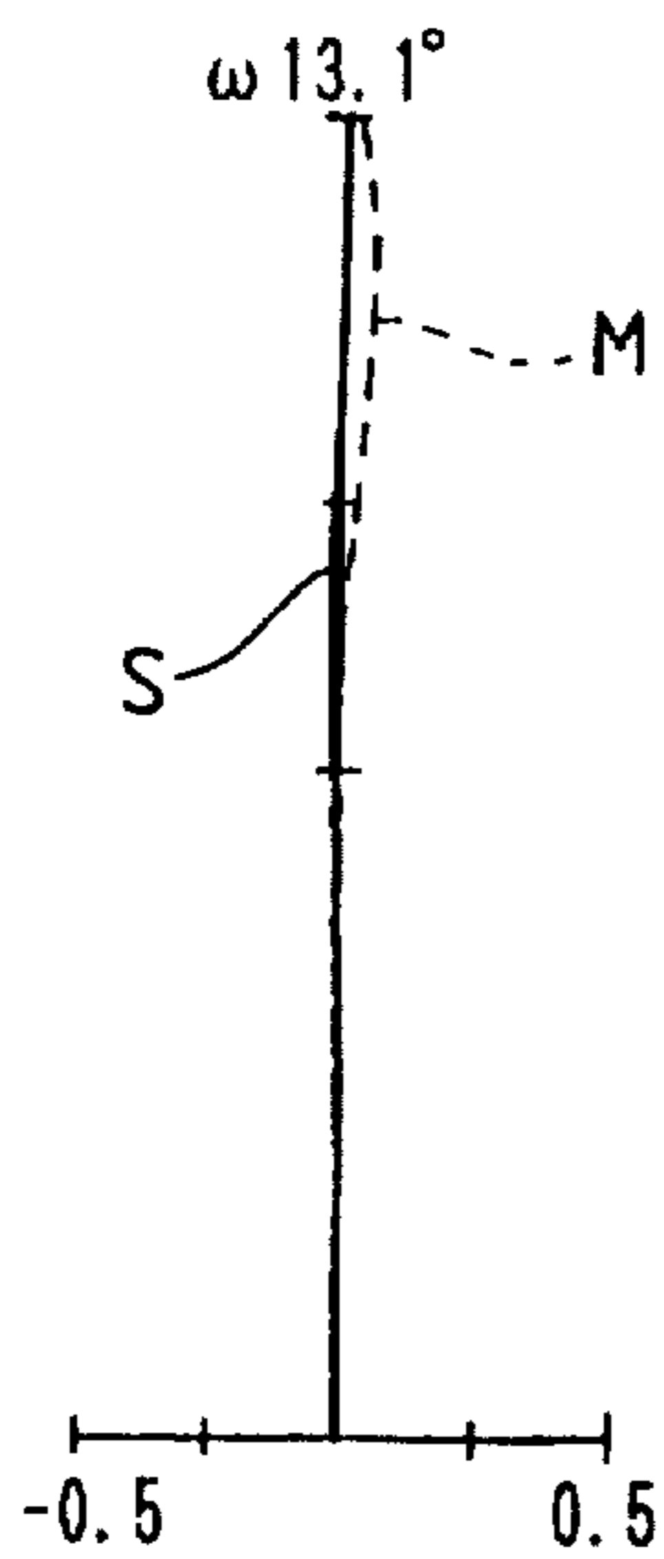
FIG. 6B ASTIGMATISM
