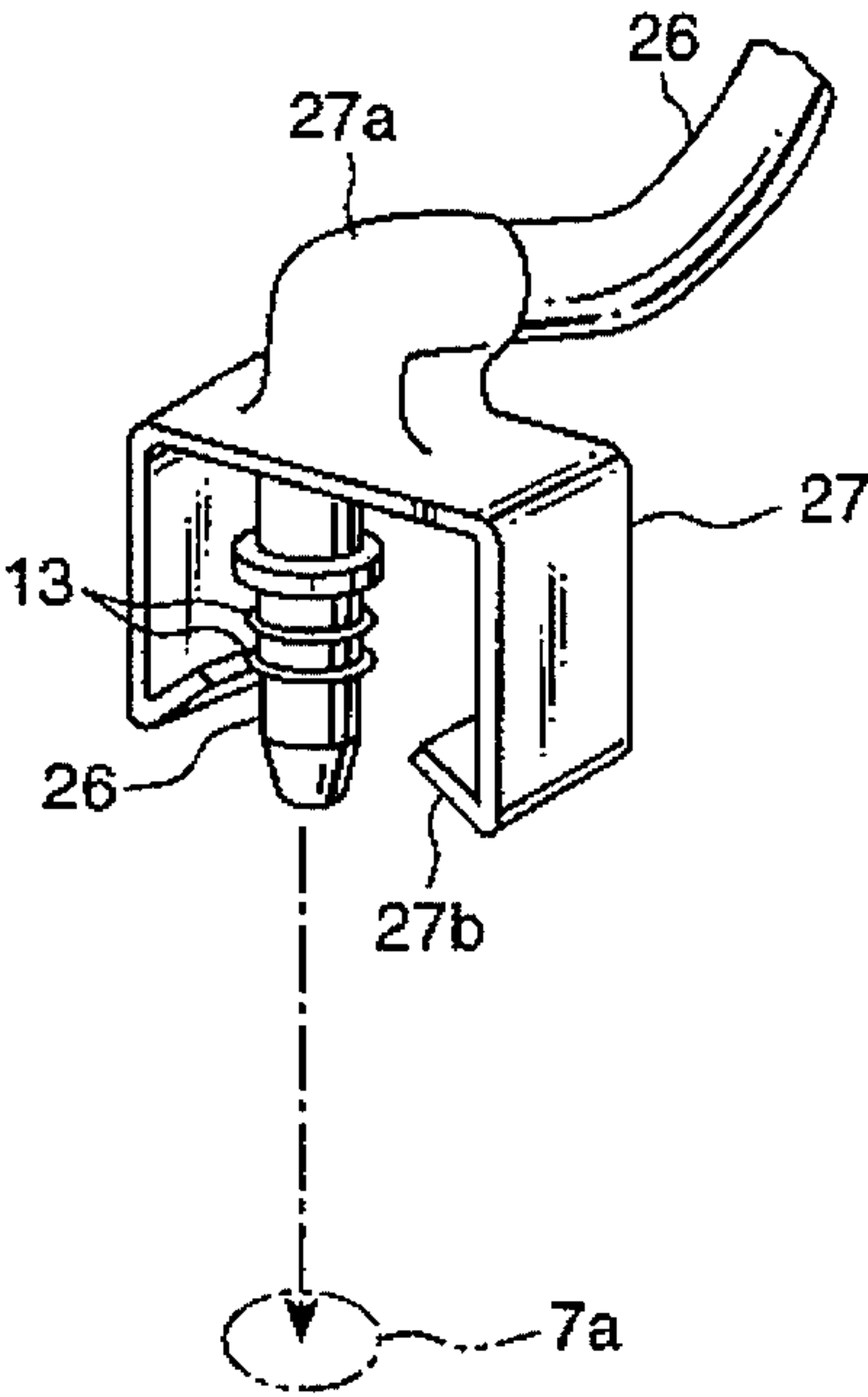
Fig. 11
