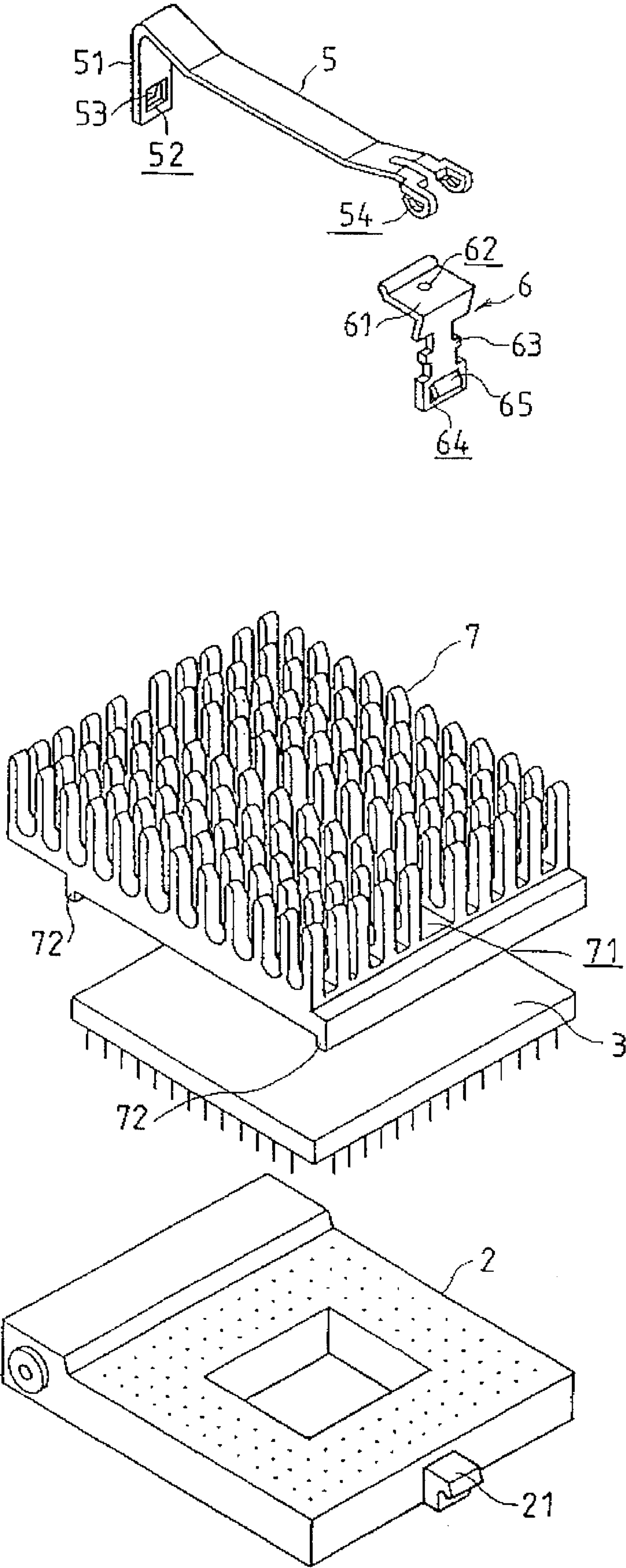
FIG 5
