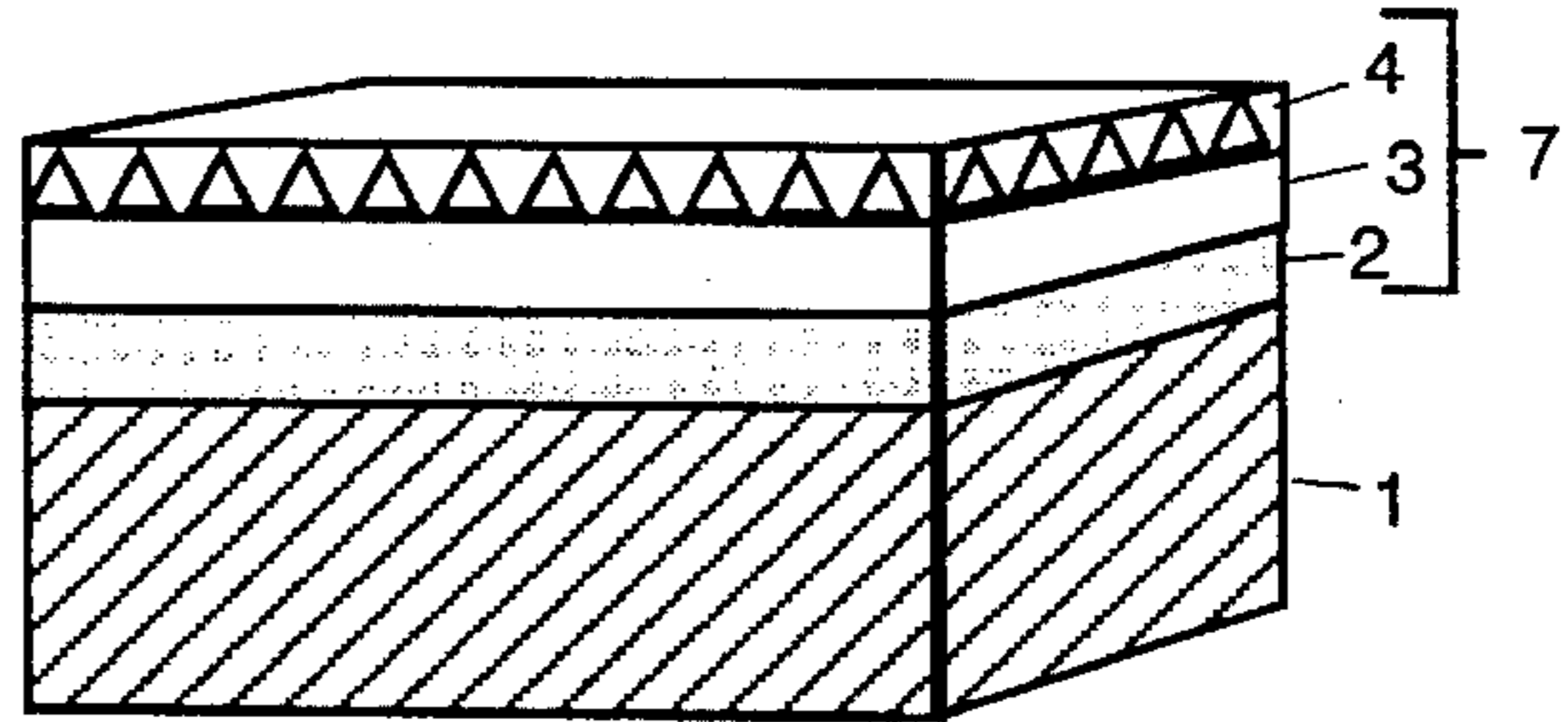
FIG. 6D
