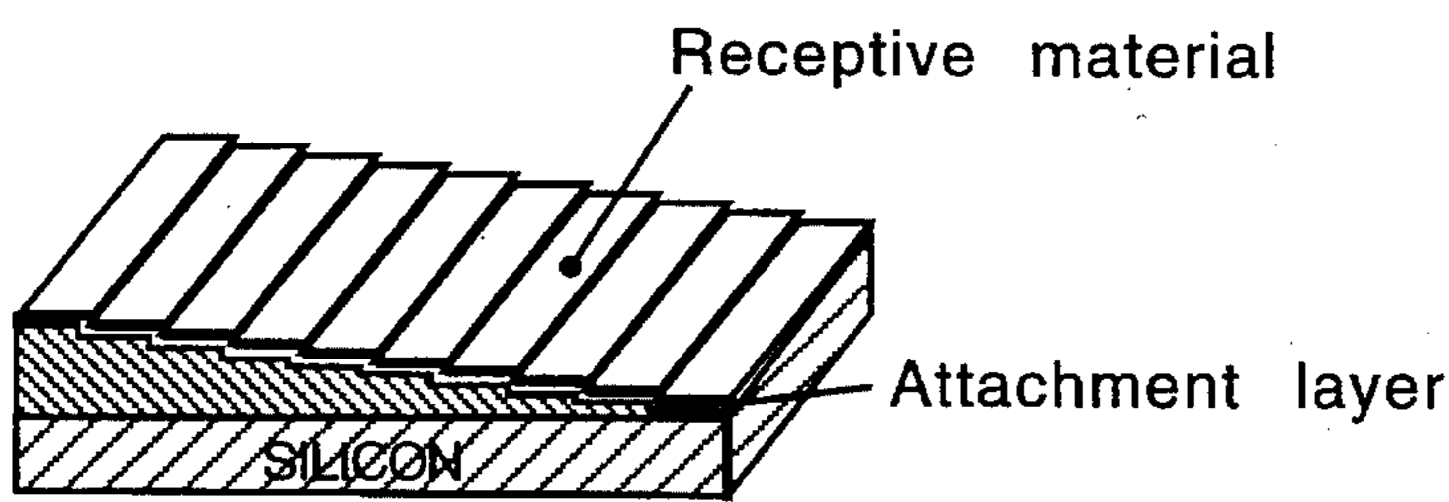
FIG. 3F
