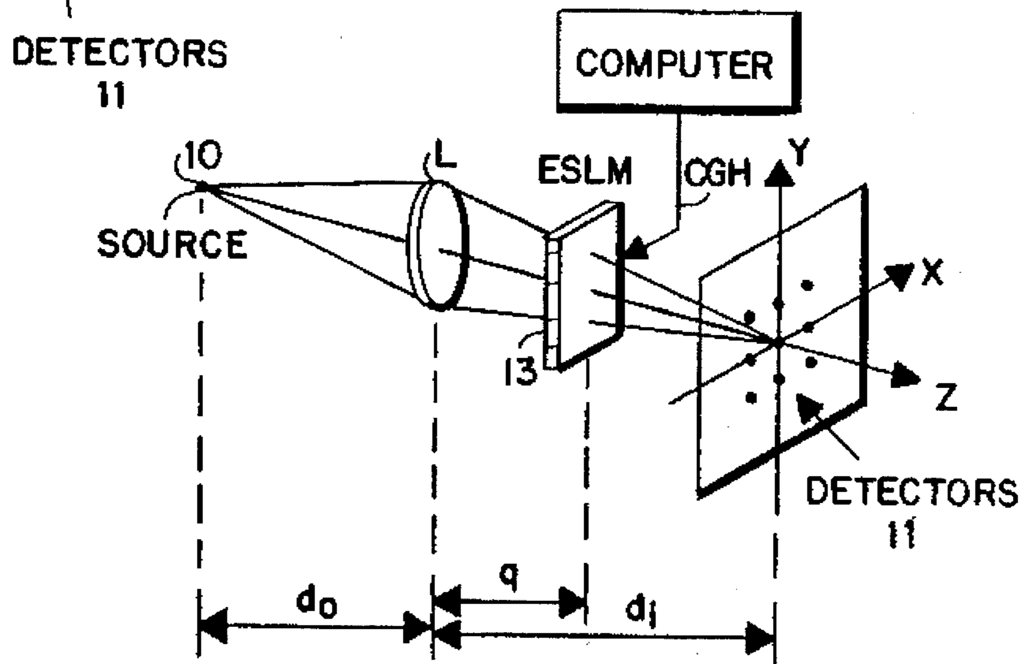
FIG. 2(b) PRIORART
