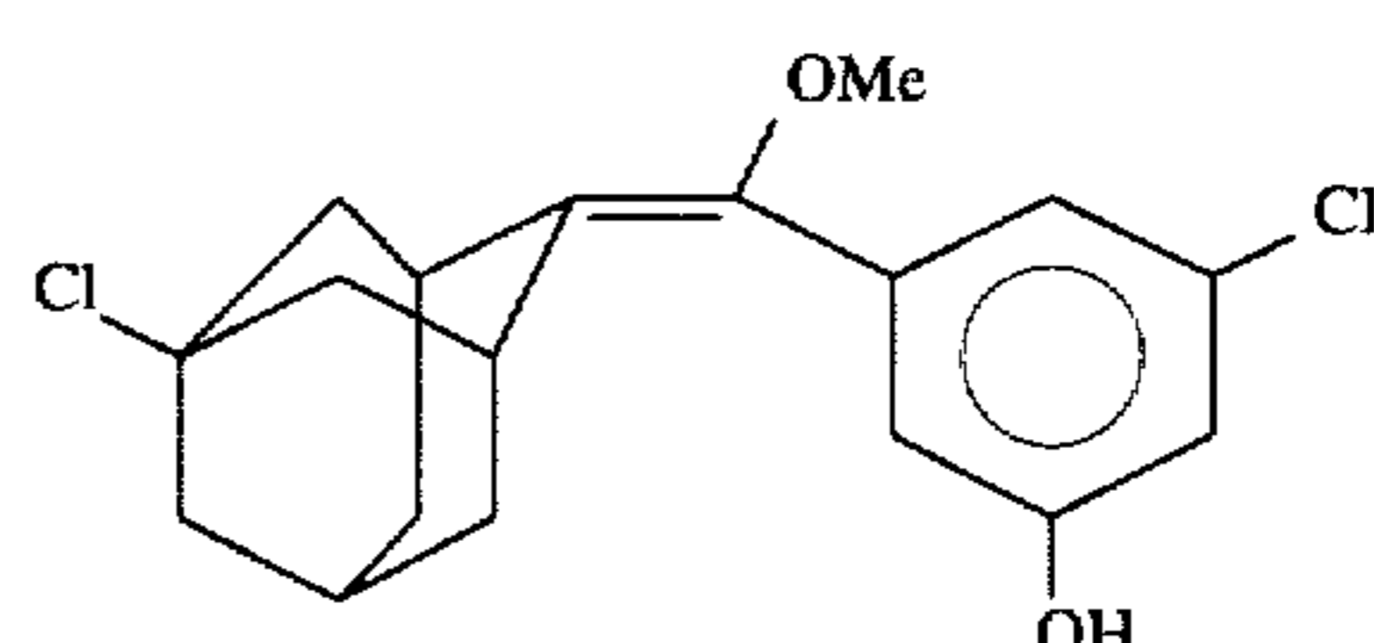
3-Chloro-5-hydroxy-1-(methoxy-5-chloro-tricyclo[3.3.1.1 3,7 ]-dec-2-ylidenemethyl)benzene ( 16 )
