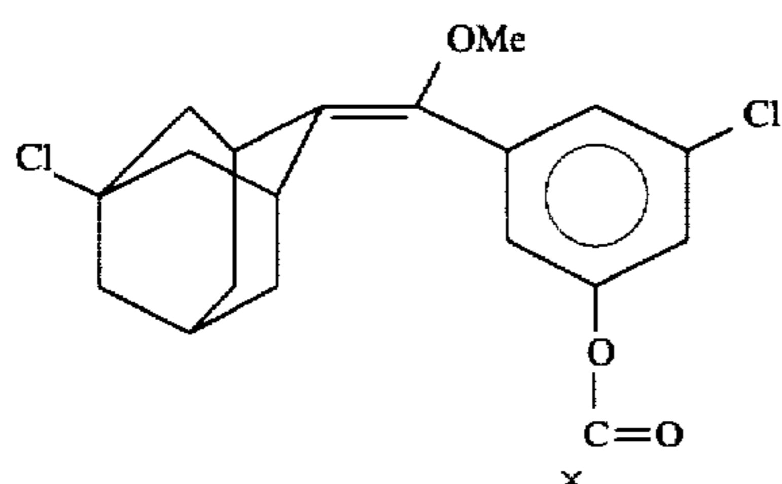
3-Chloro-5-pivaloyloxy-1-(methoxy-5-chloro-tricyclo[3.3.1.1 3,7 ]-dec-2-ylidenemethyl)benzene ( 15 )
