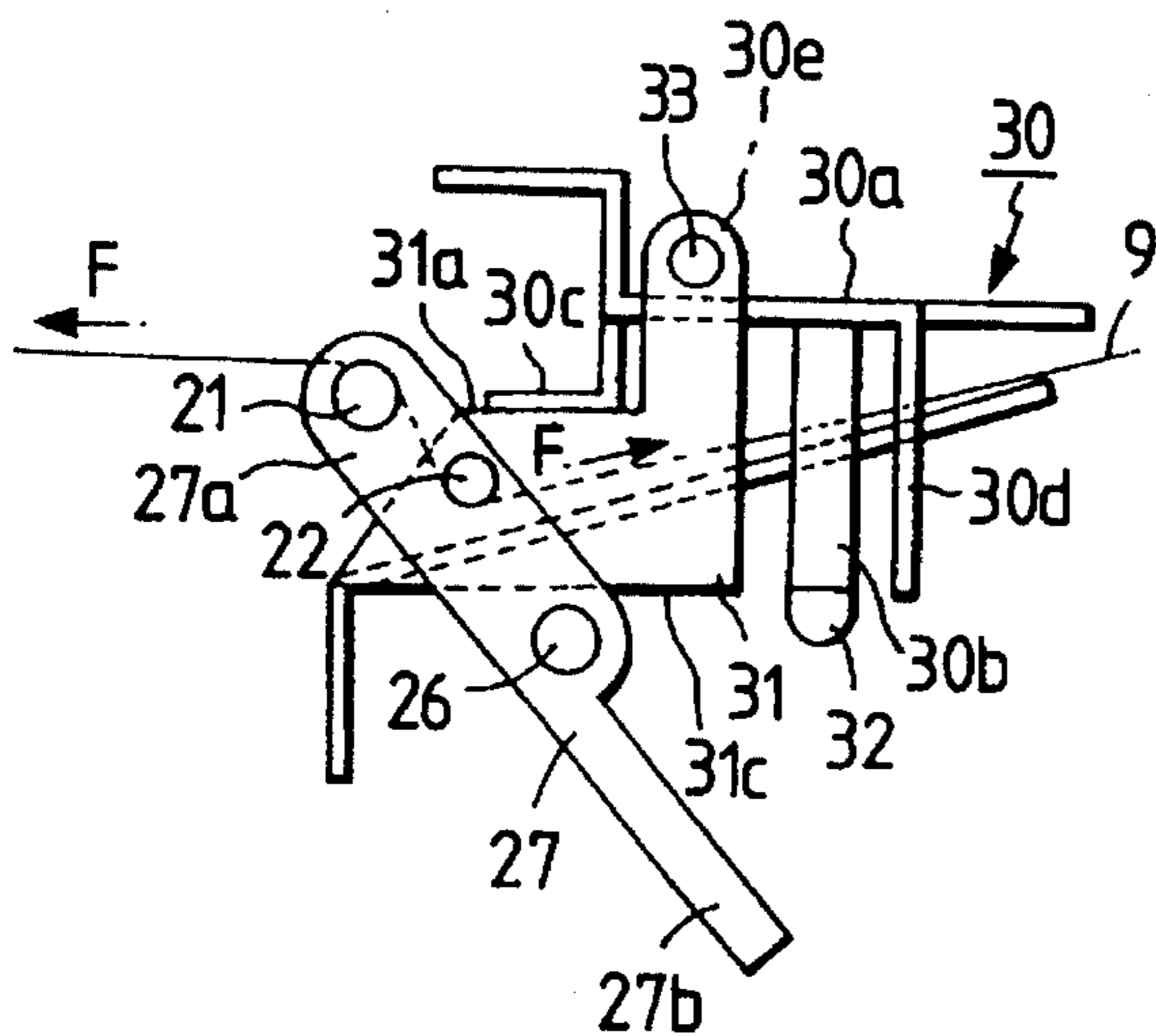
FIG. 3A
