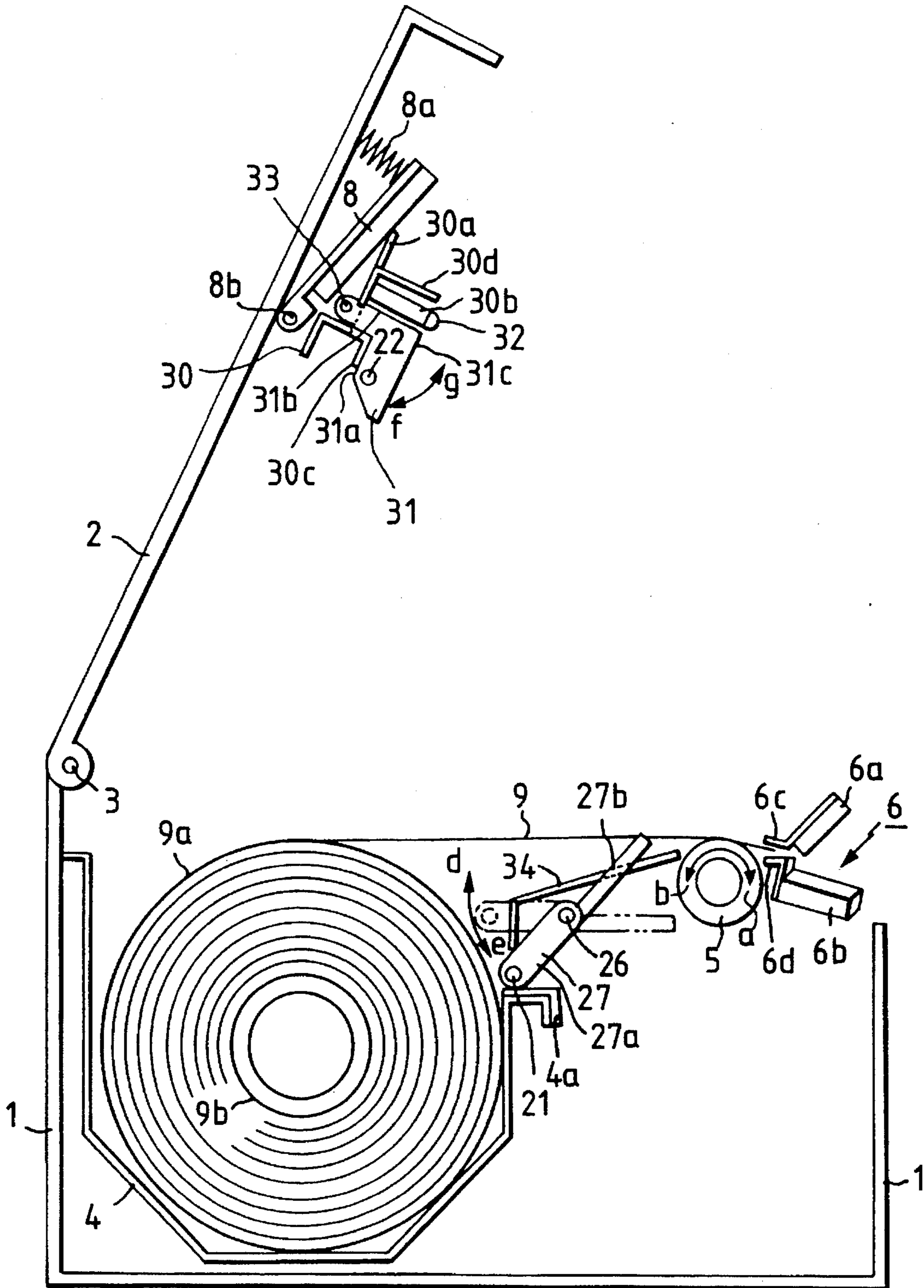
FIG. 8
