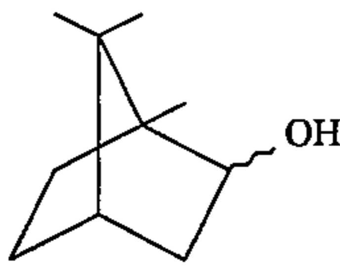
isoborneol;
