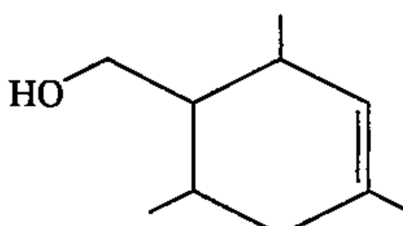
isocyclogeranol;
