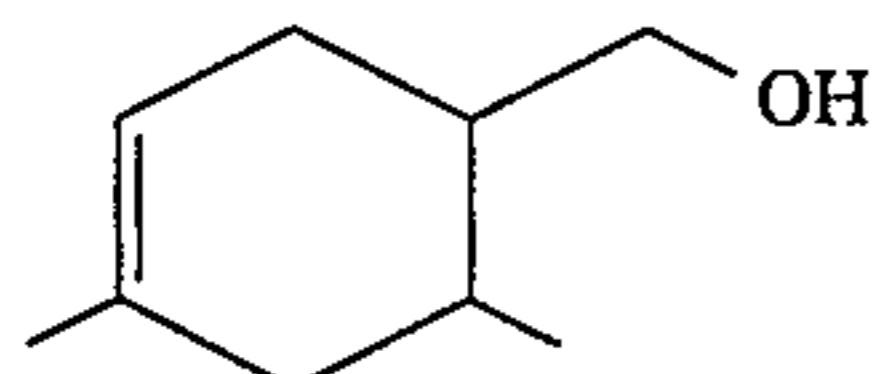
floralol;
