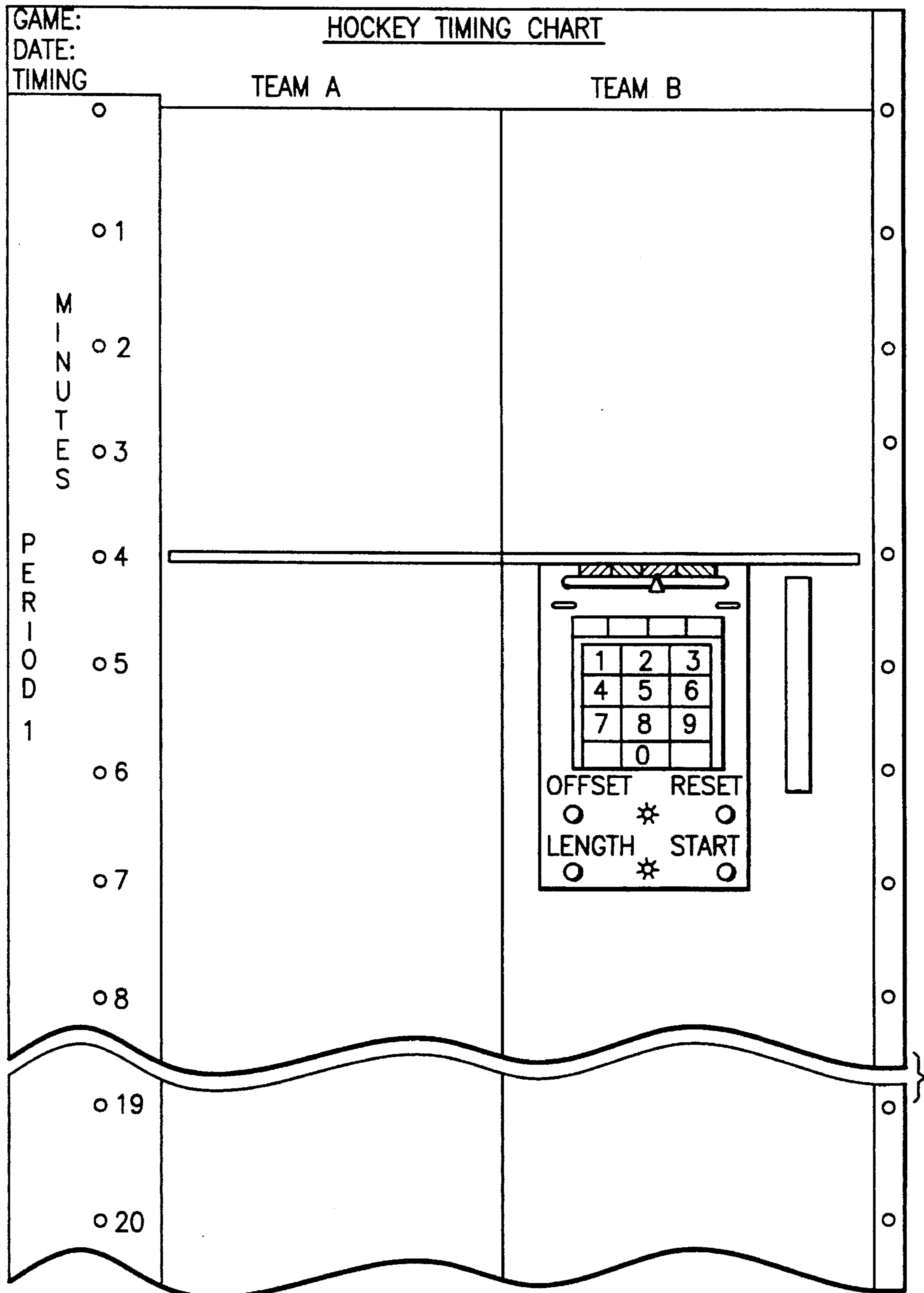
FIG. 18B
