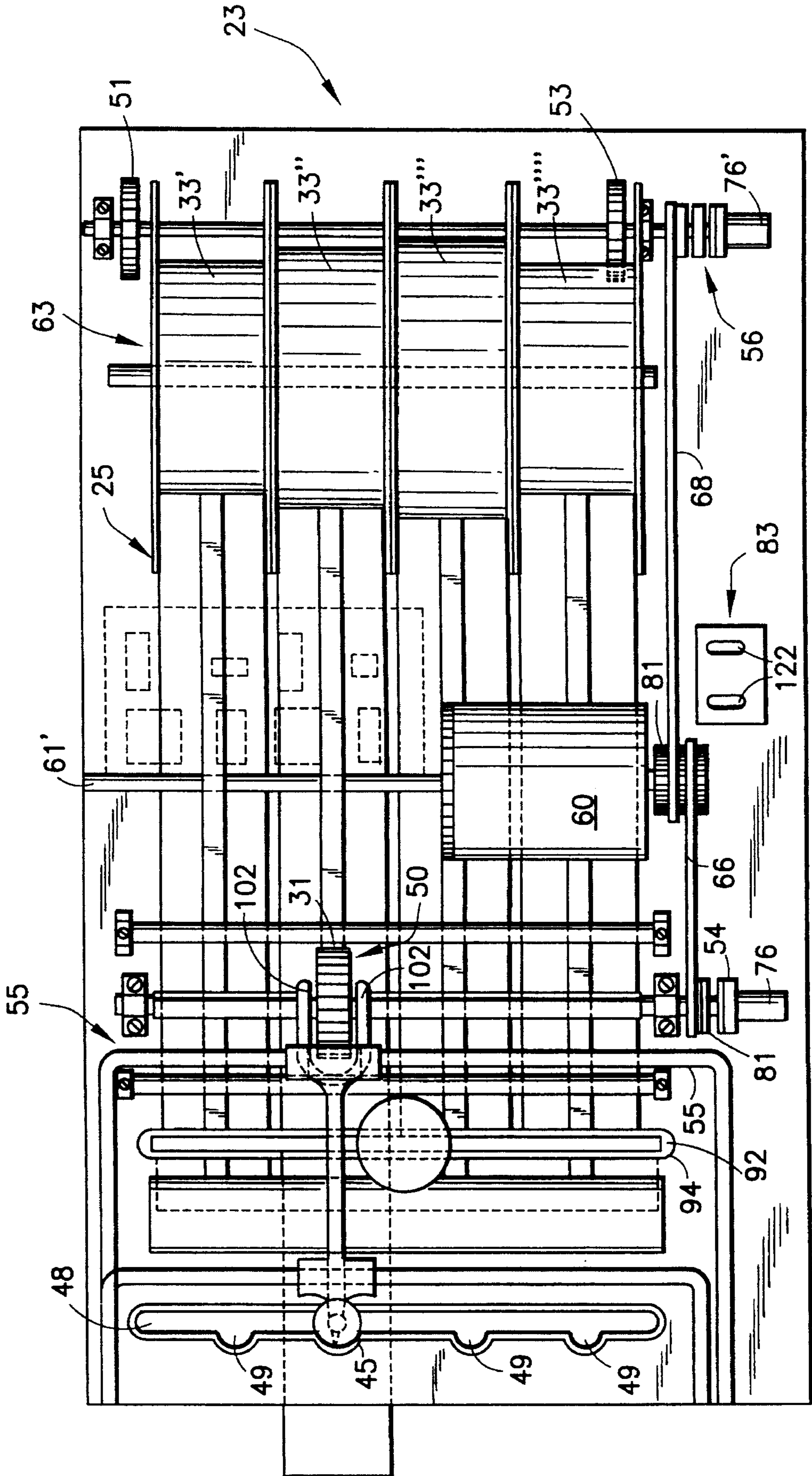
FIG. 6
