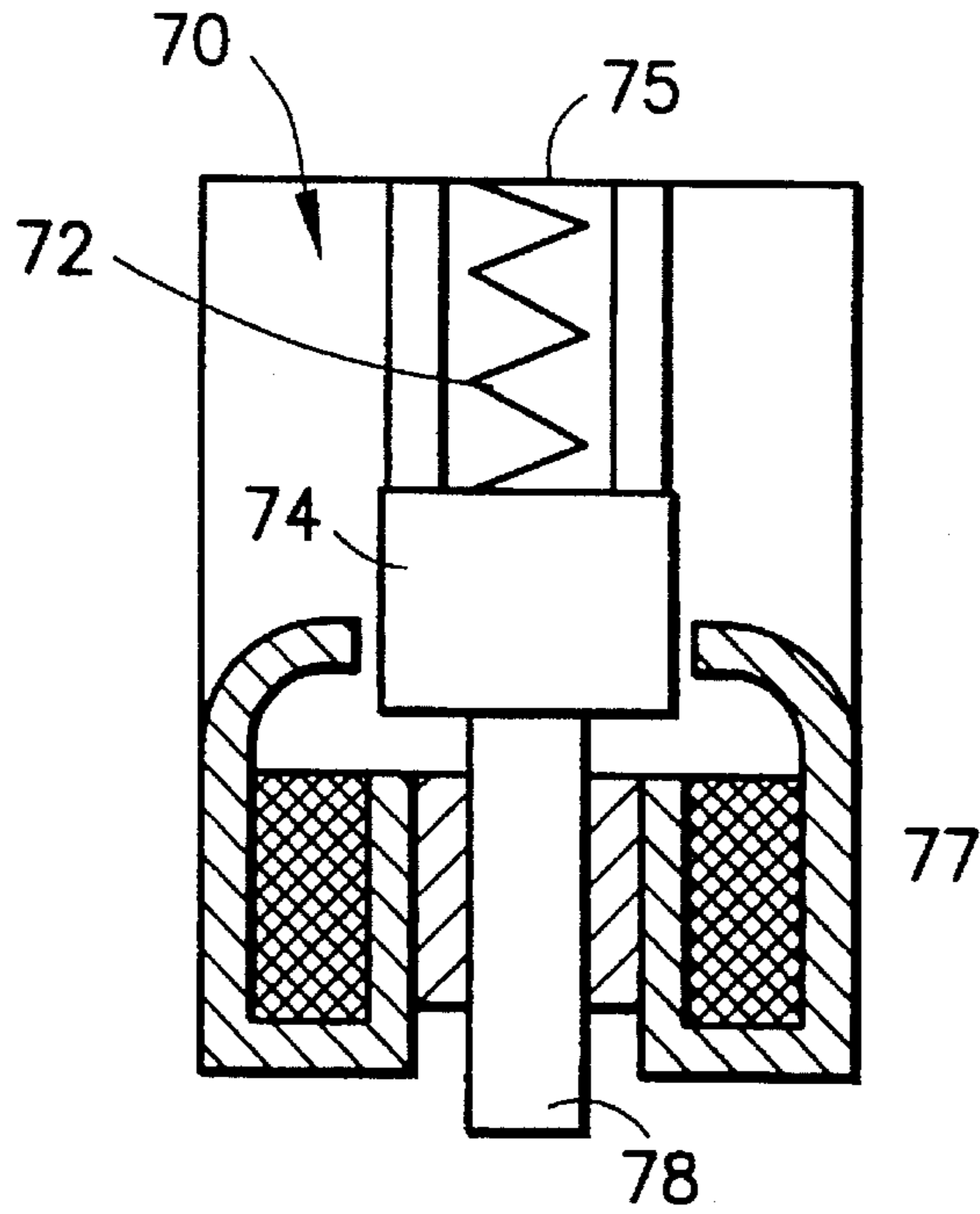
FIG. 6A
