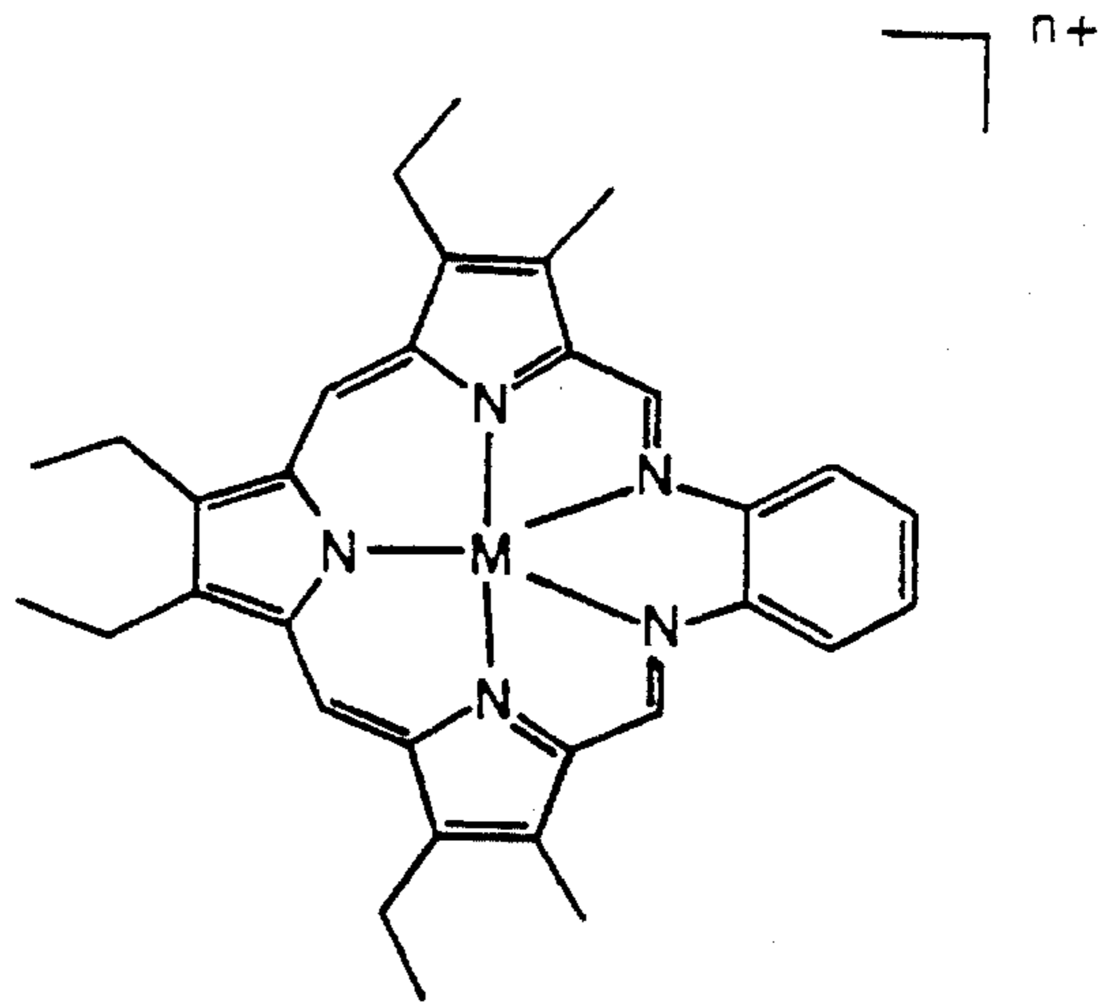
2A. M = H, n = 0 3A. M = Cd, n = 1
