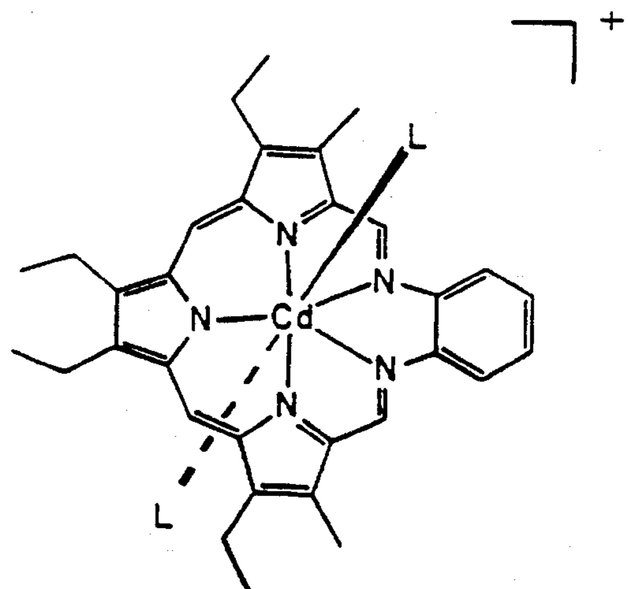
5aA. L = pyr 5bA. L = BzIm
