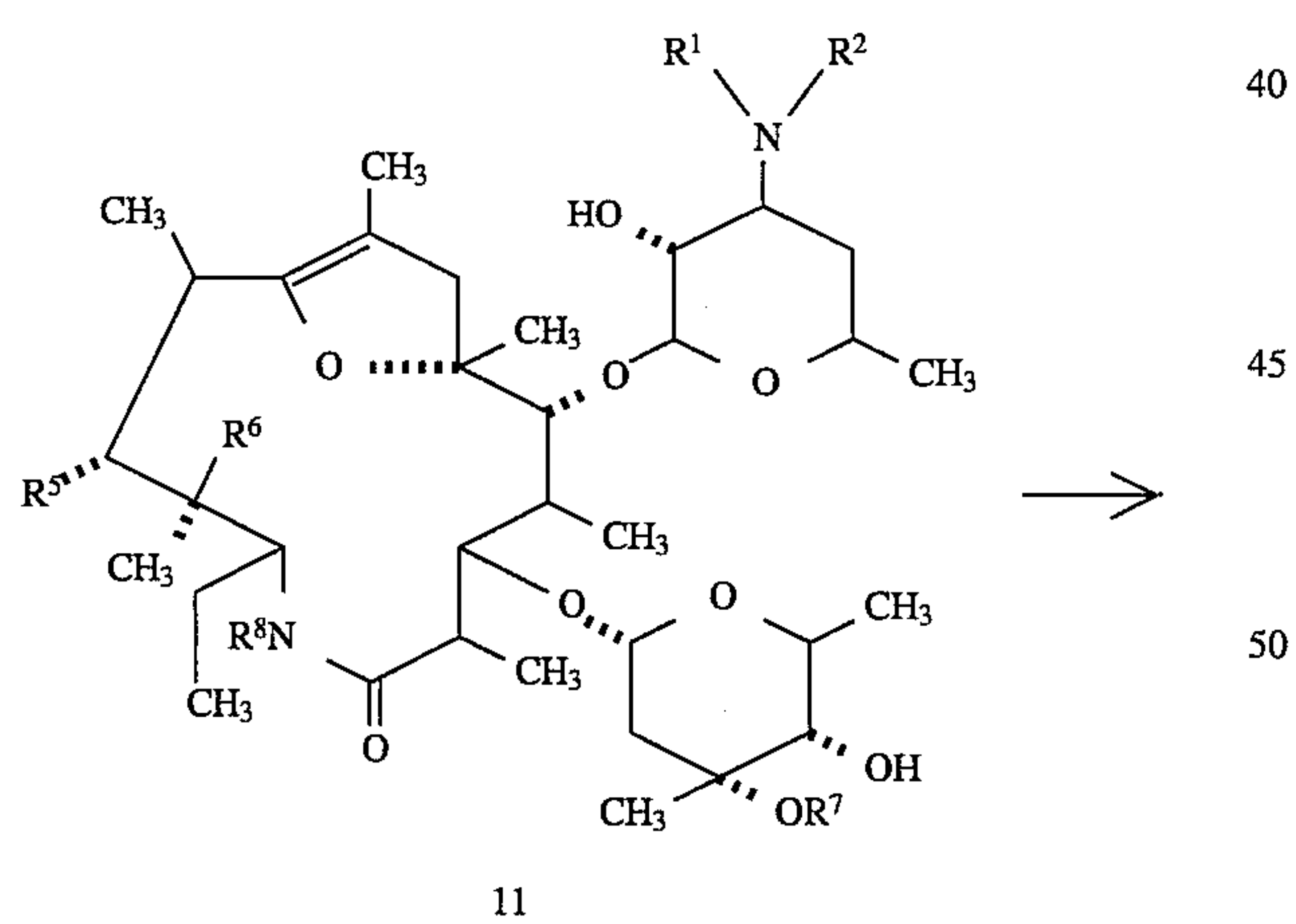
Scheme VI
