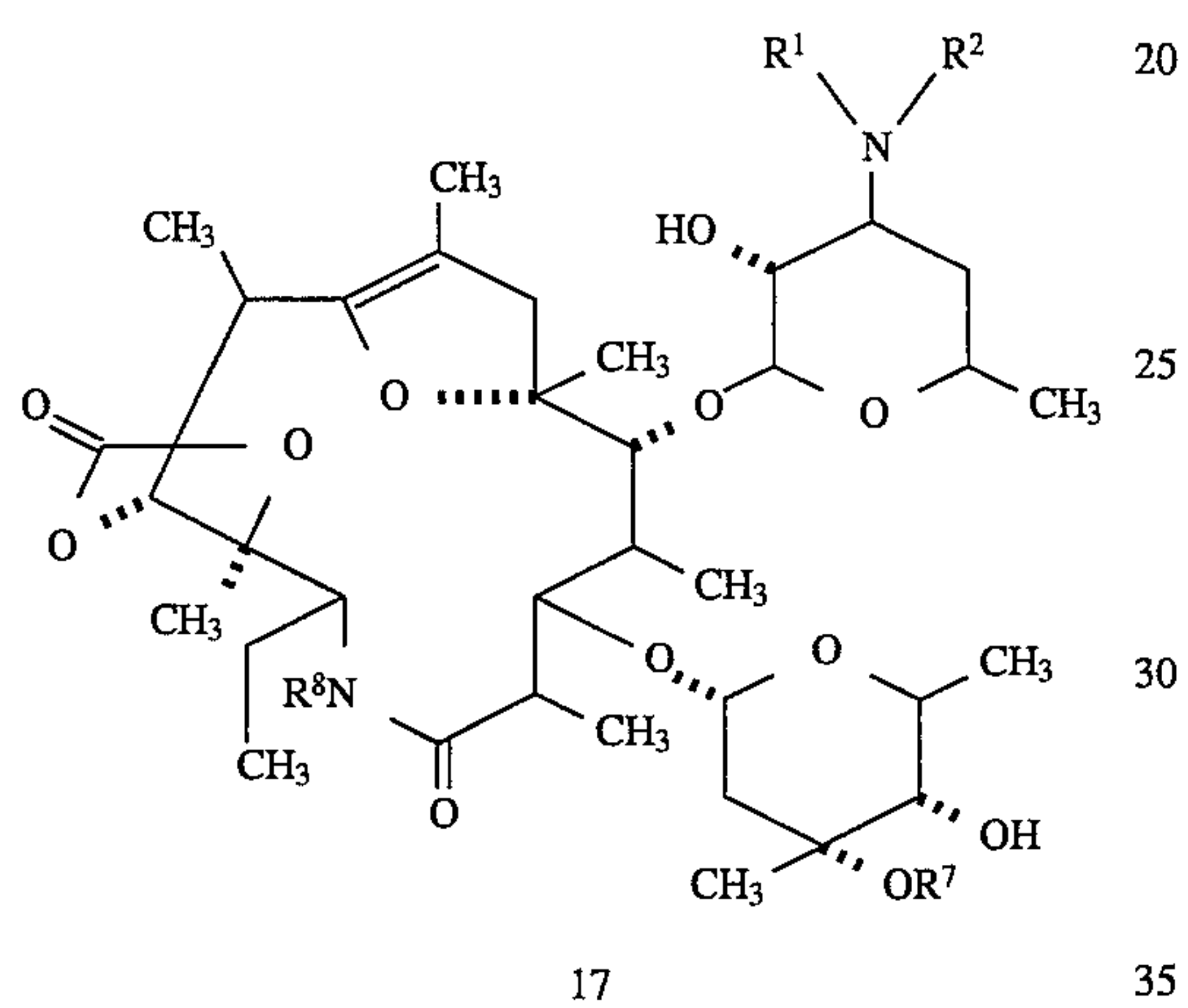
Scheme VI
