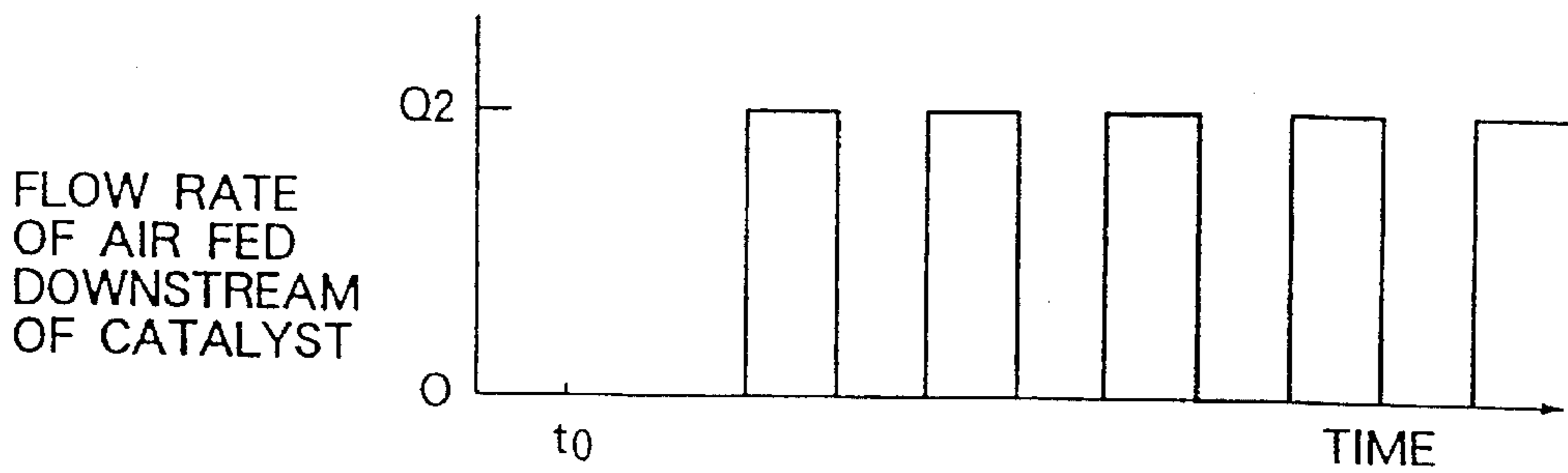
FIG. 18(C)
