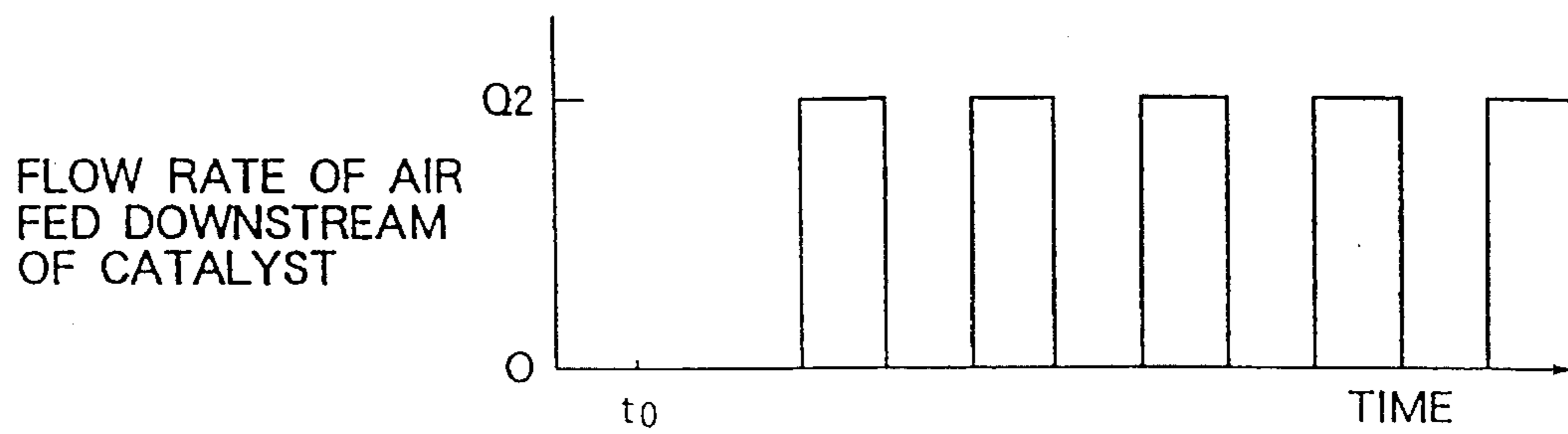
FIG. 21(B)
