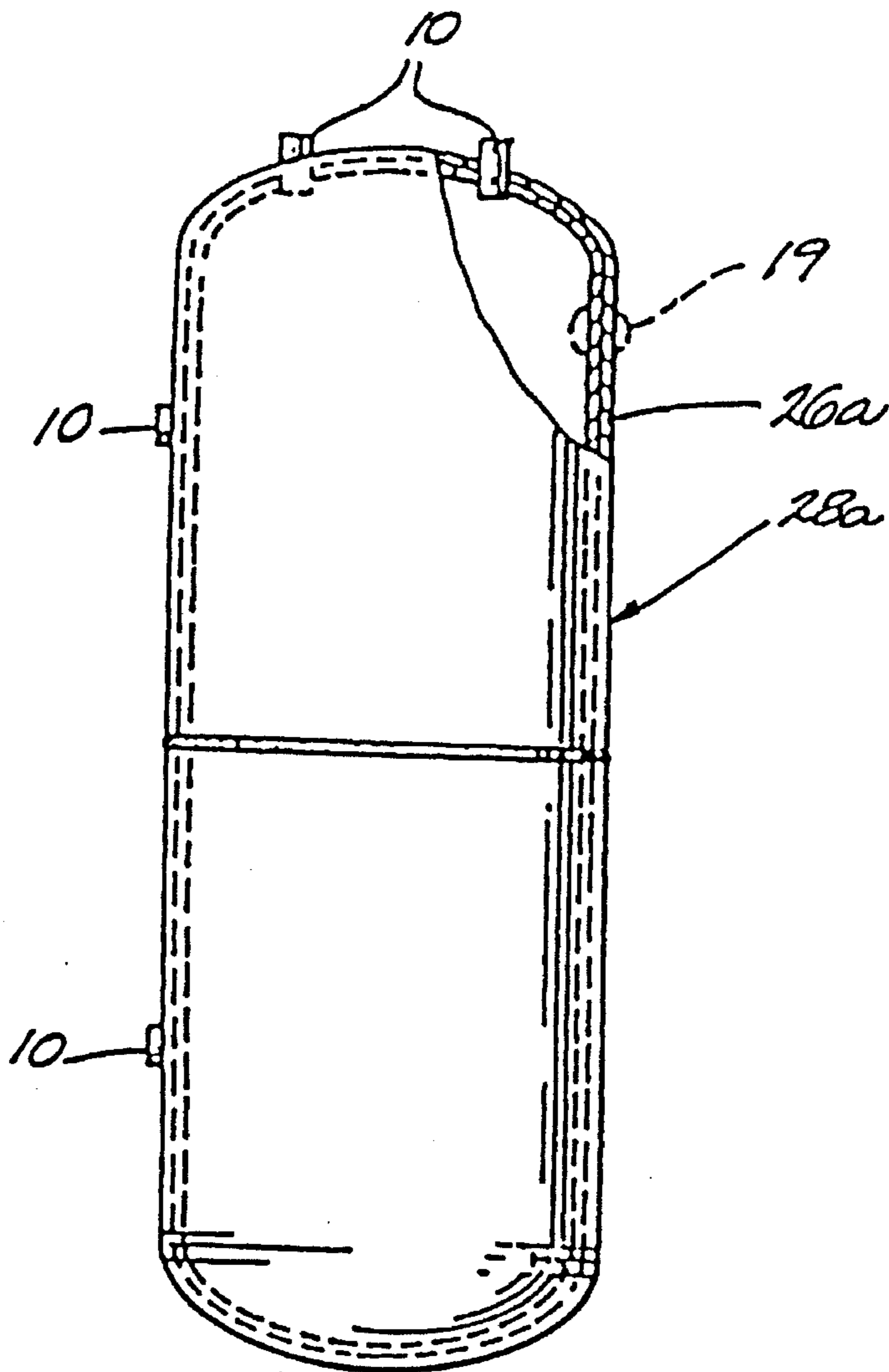
Fig. 12. PRIOR ART
