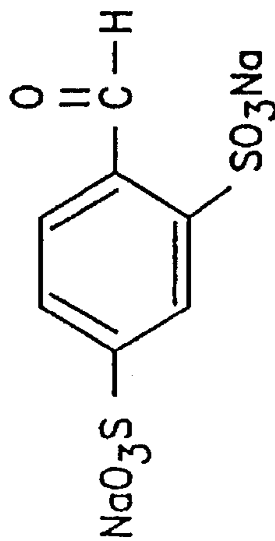
4-Formyl-1,3-benzenesulfonic Acid
