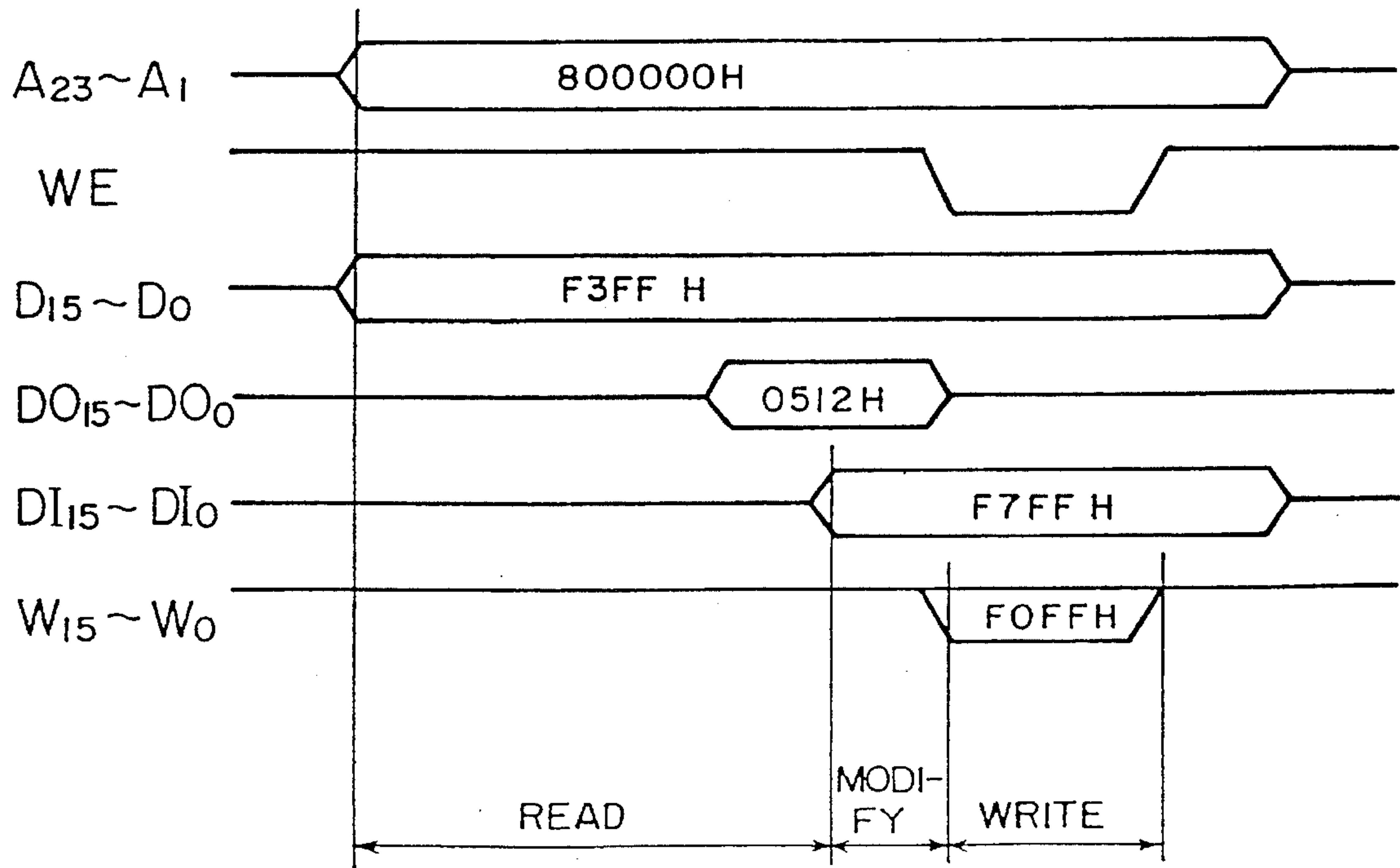
FIG. 37
