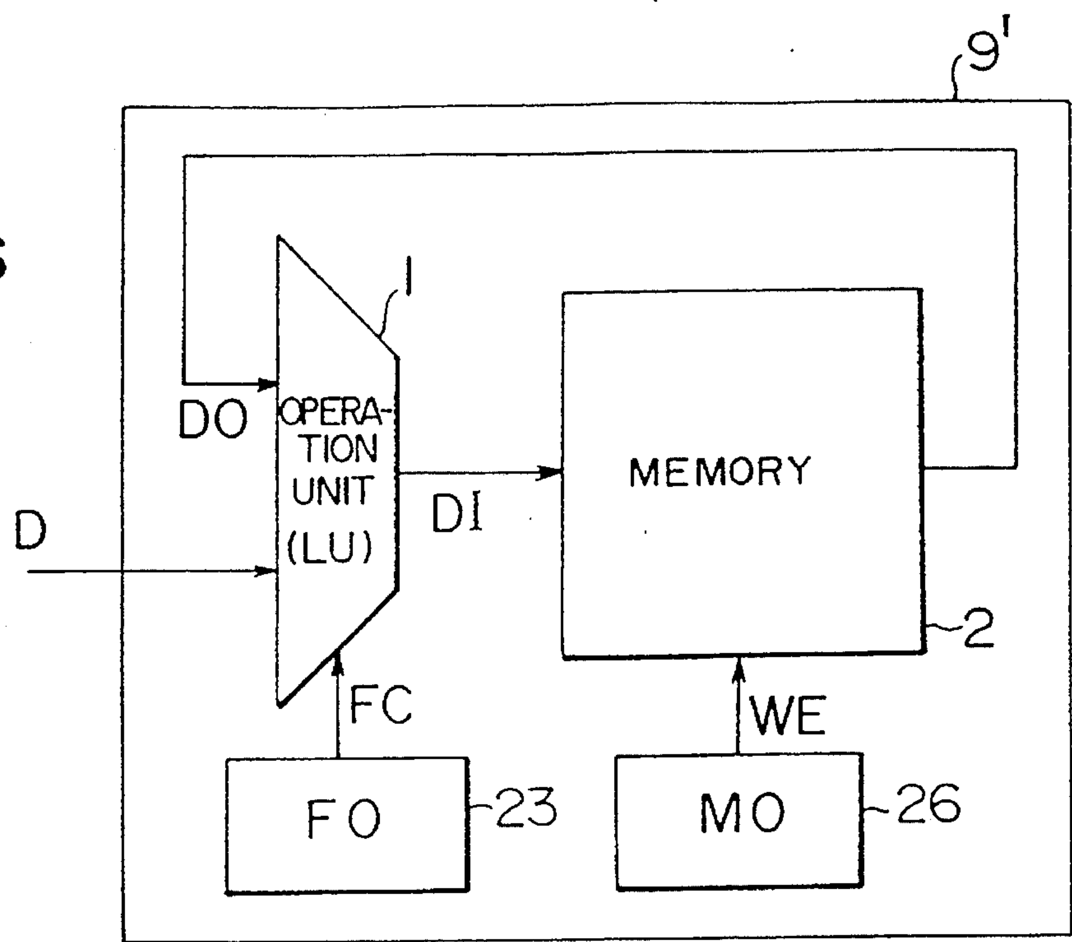
FIG. 26
