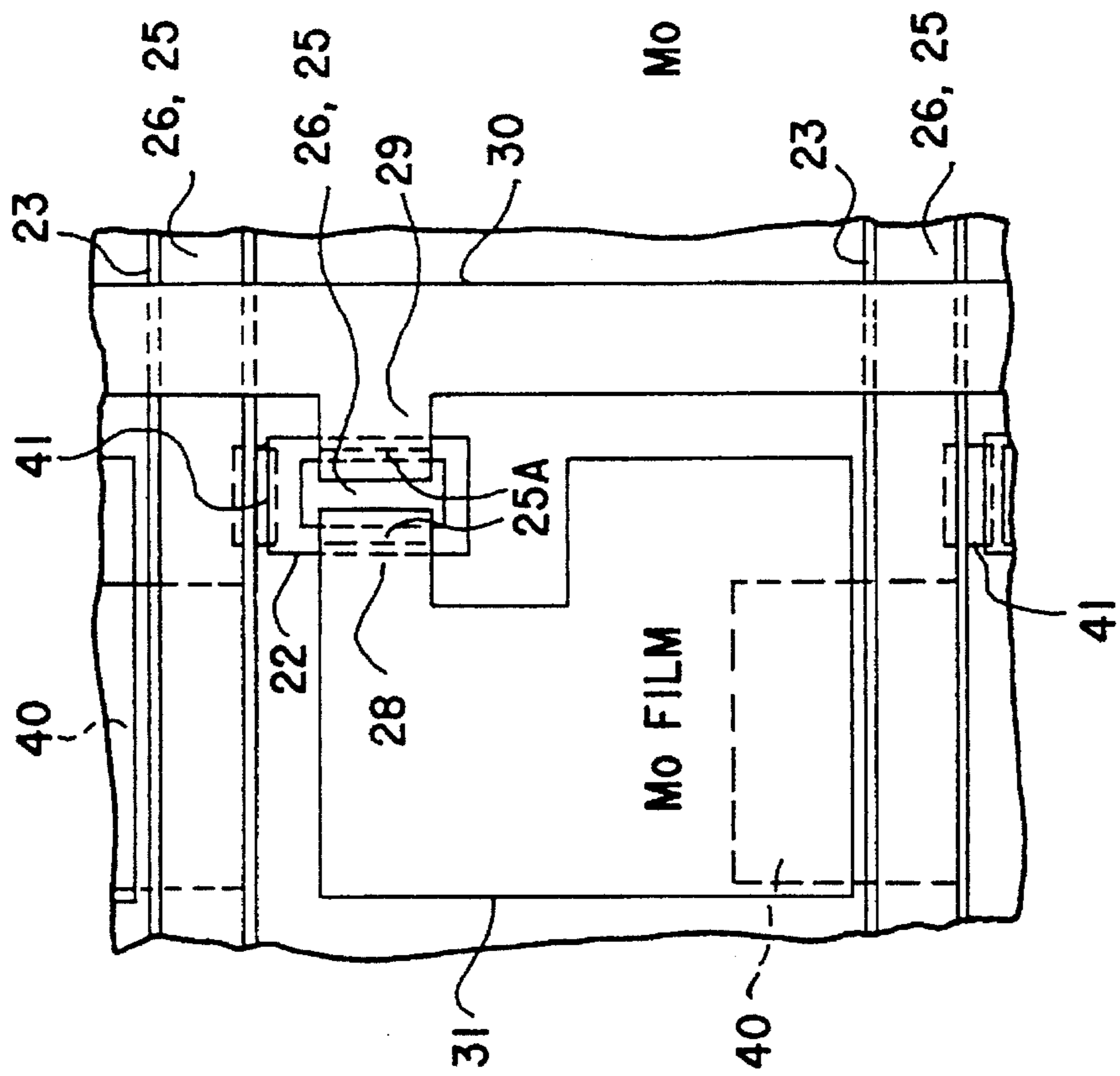
FIG. 35E
