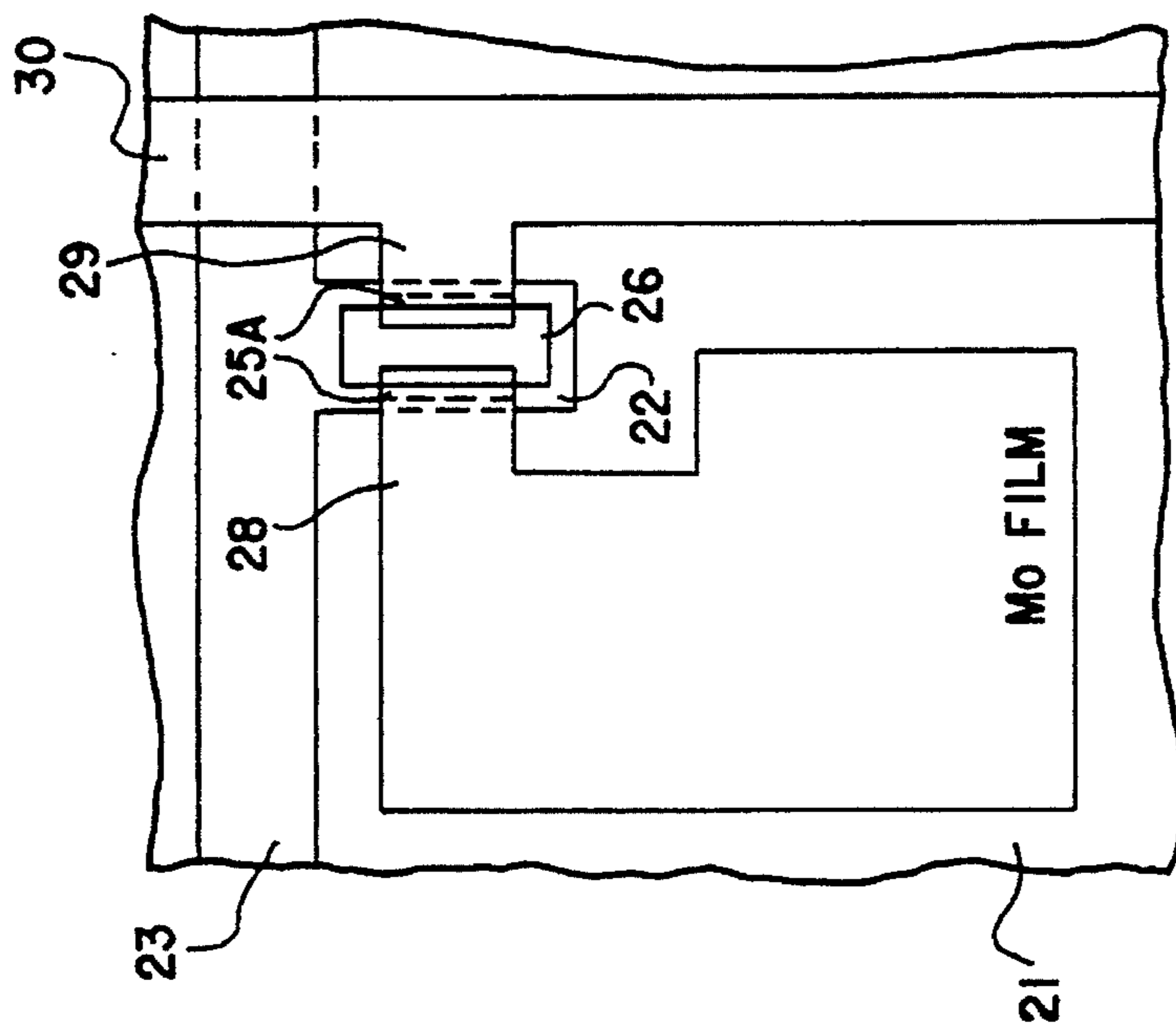
FIG.12A
