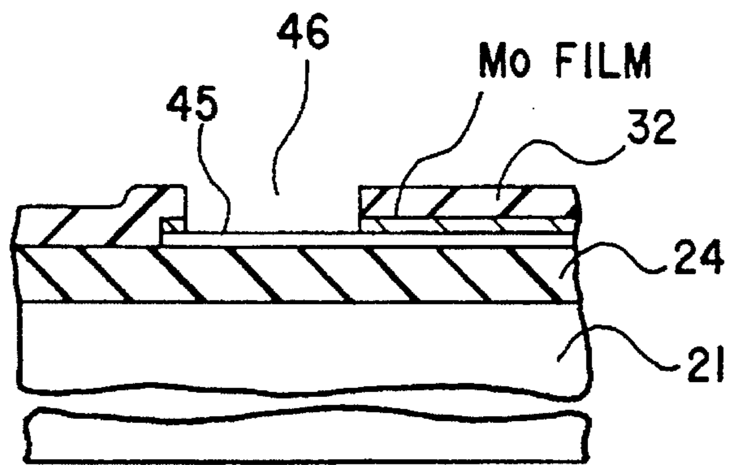
FIG.37B
