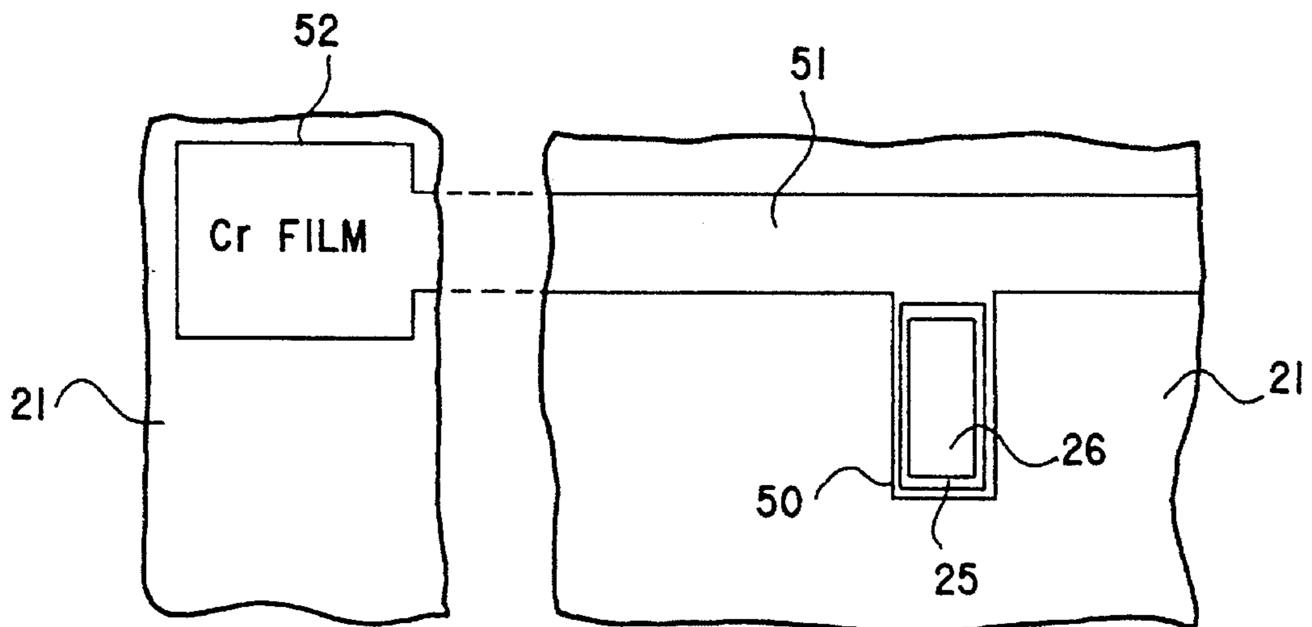
FIG.39B
