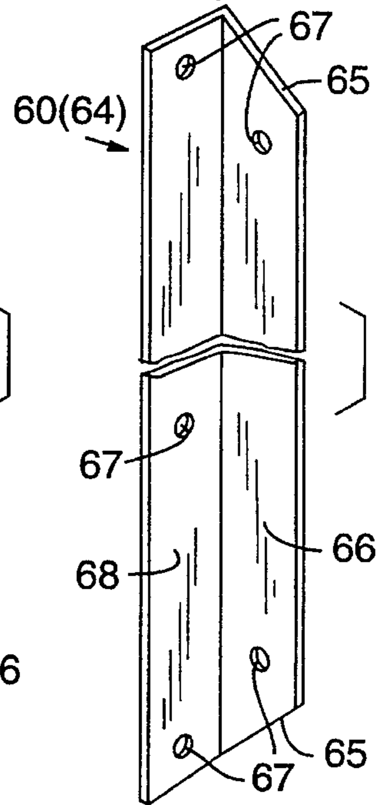
FIG. 6
