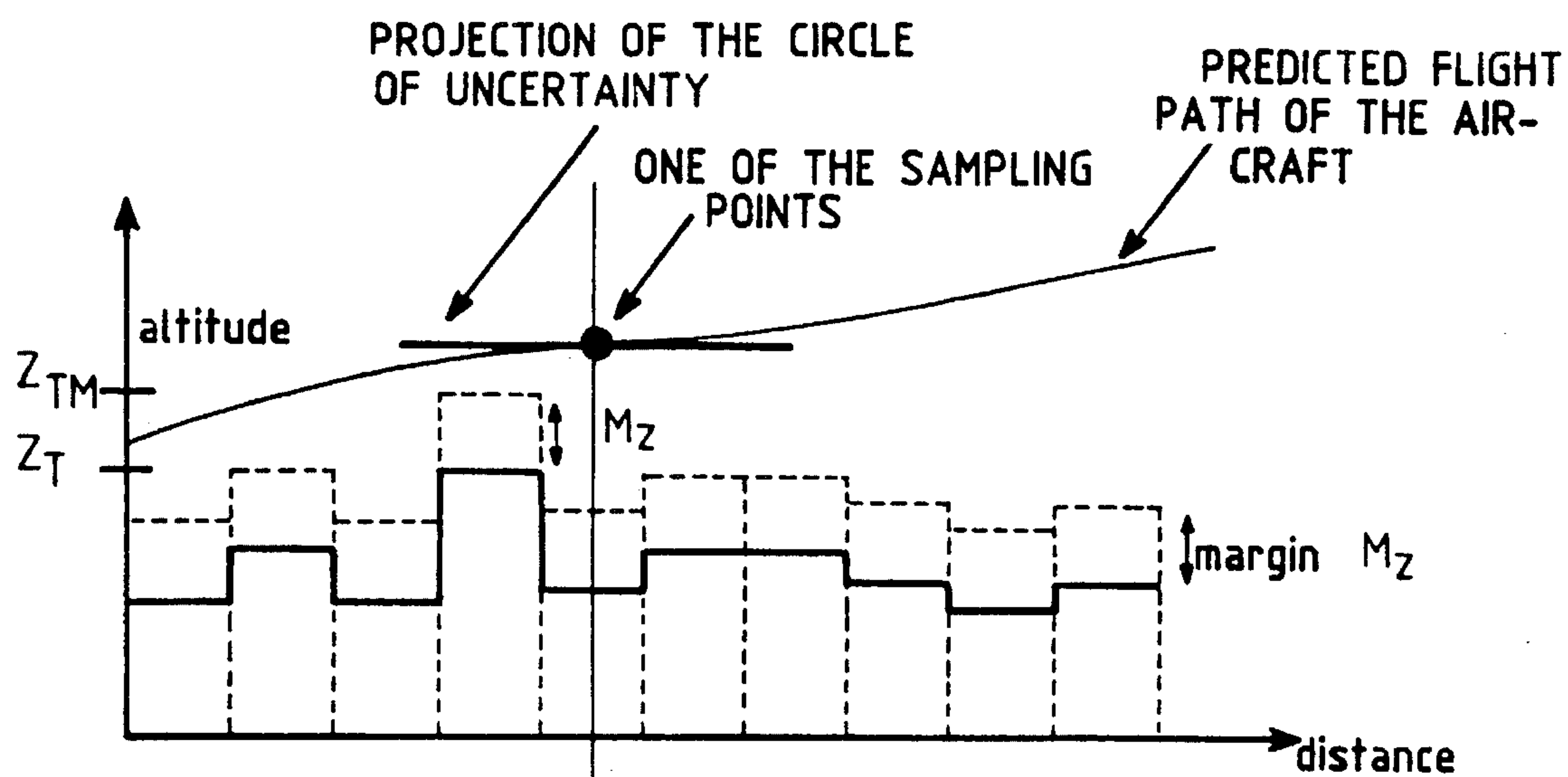
FIG. 17a - ANTICOLLISION LAW
