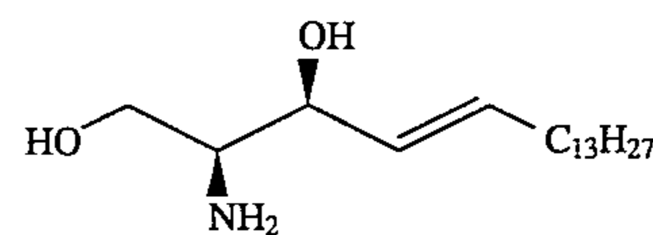
L-threo-sphingosine (2)
