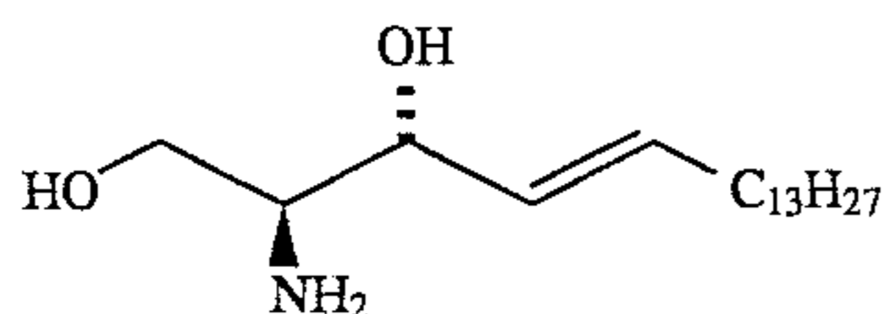
D-erythro-sphingosine (1)
