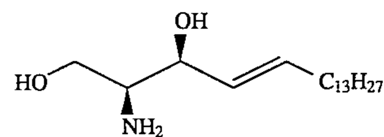
L-threo-sphingosine (2)
