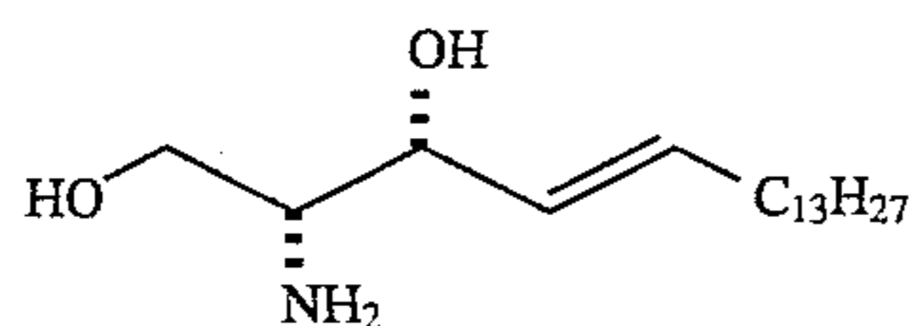
D-threo-sphingosine (4)
