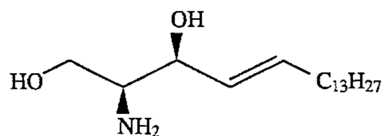
L-threo-sphingosine (2)
