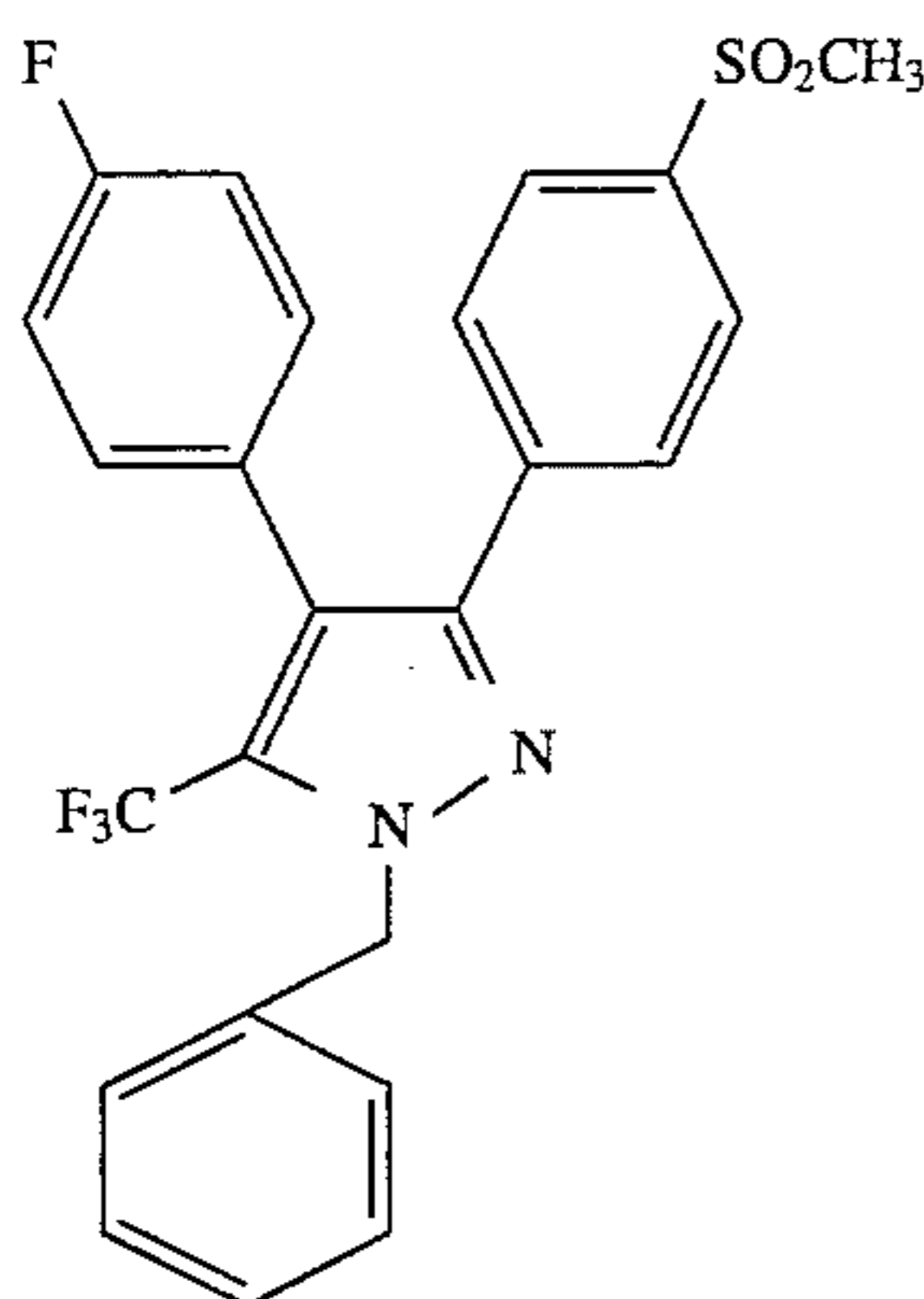
1-Benzyl-4-(4-fluorophenyl)-3-[4-(methylsulfonyl)phenyl]-5-(trifluoromethyl)pyrazole
