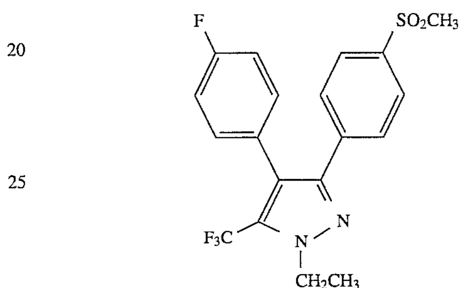
1-Ethyl-4-(4-fluorophenyl)-3-[4-(methylsulfonyl)phenyl]-5-(trifluoromethyl)-1H-pyrazole
