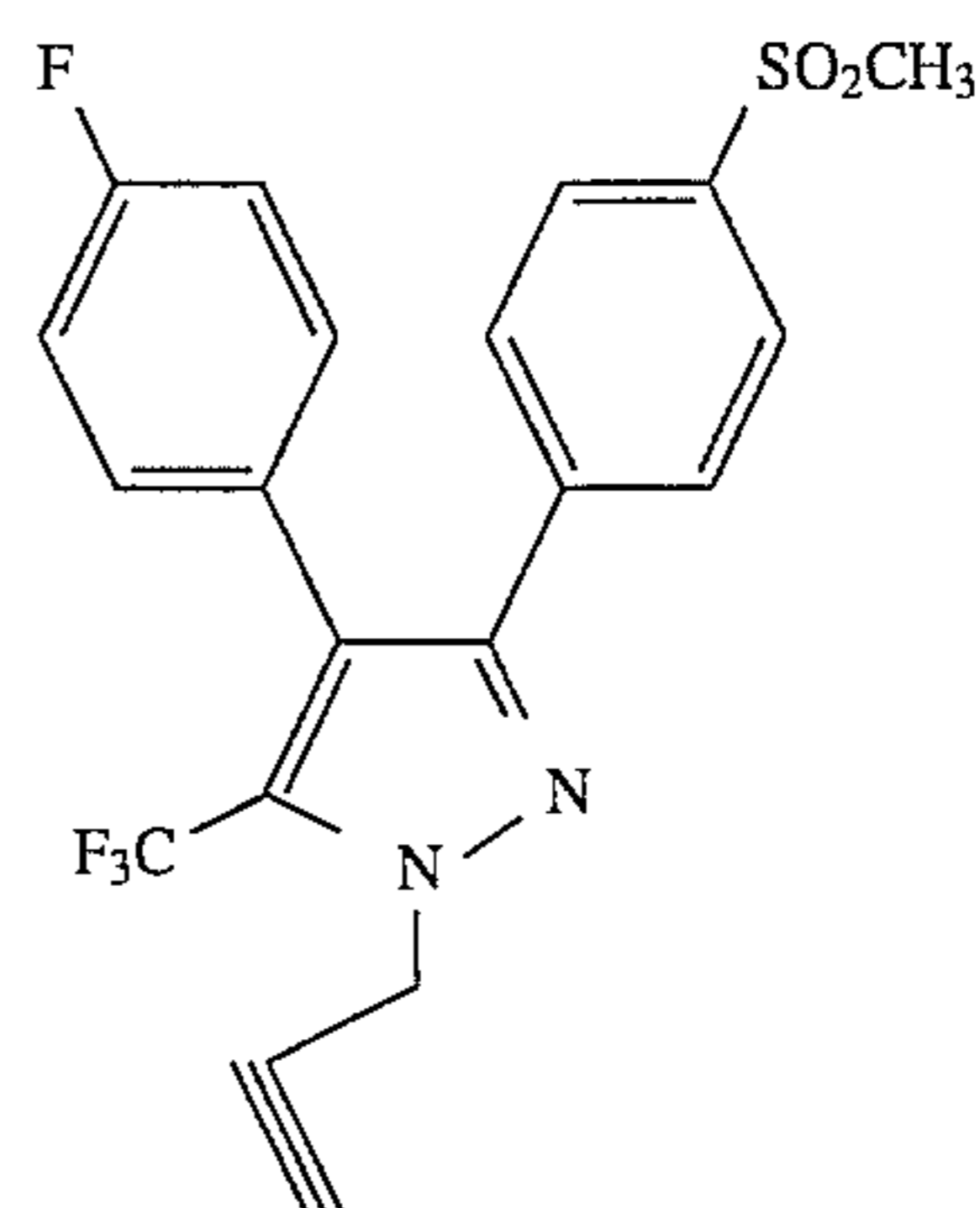
4-(4-Fluorophenyl)-3-[4-(methylsulfonyl)phenyl]-1-propargyl-5-(trifluoromethyl)-1H-pyrazole
