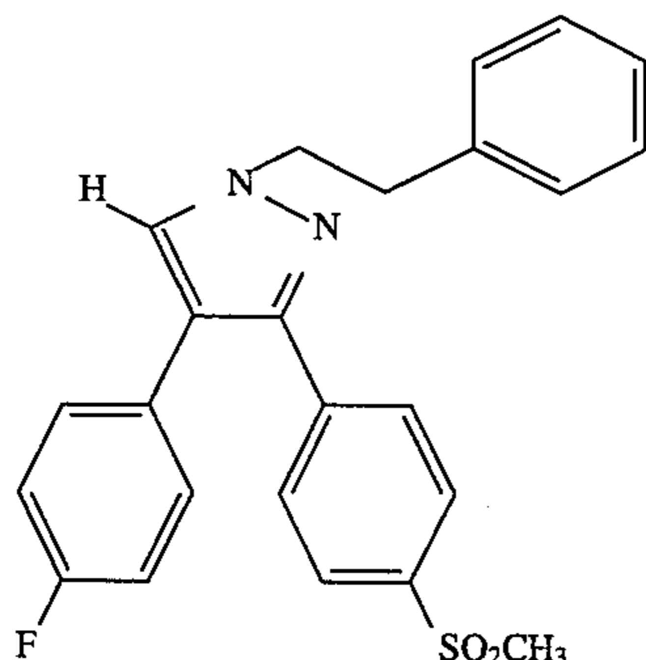
4-(4-Fluorophenyl)-3-[4-(methylsulfonyl)phenyl]-1-(2-phenylethyl)-1H-pyrazole
