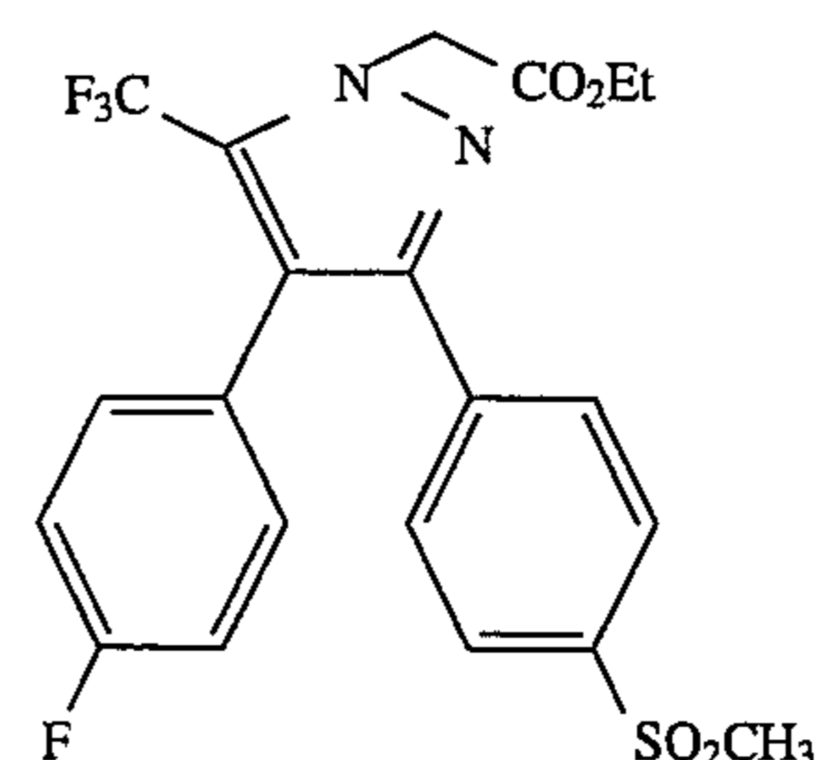
Ethyl[4-(4-fluorophenyl)-3-[4-(methylsulfonyl)phenyl]-5-(trifluoromethyl)-1H-pyrazol-1-yl]acetate
