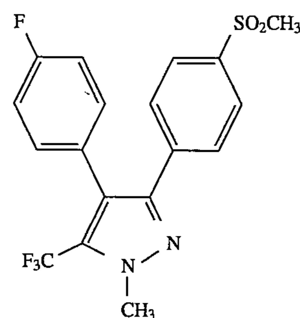
4-(4-Fluorophenyl)-1-methyl-3-[4-(methylsulfonyl)phenyl]-5-(trifluoromethyl)pyrazole
