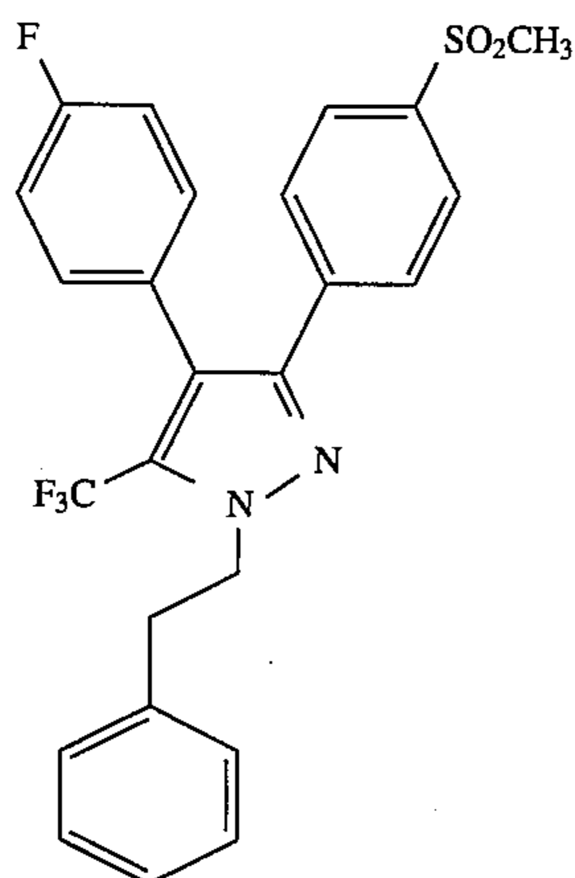
4-(4-Fluorophenyl)-3-[4-(methylsulfonyl)phenyl]-1-(2-phenylethyl)-5-(trifluoromethyl)pyrazole
