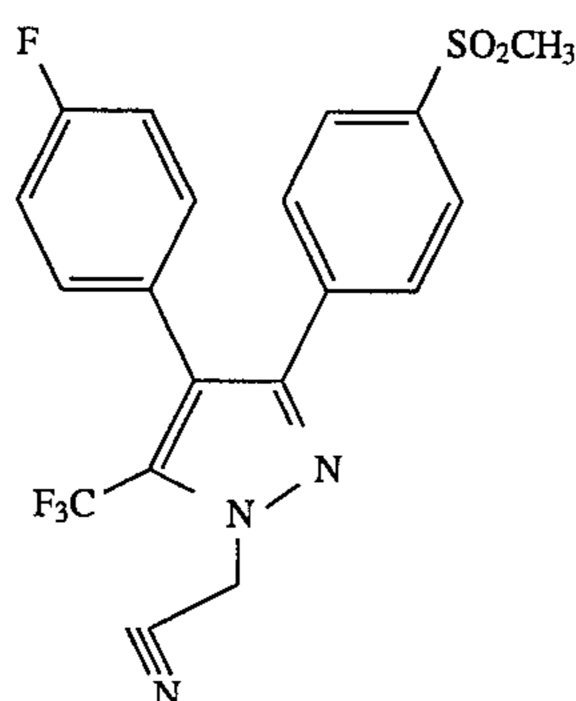
1-Cyanomethyl-4-(4-fluorophenyl)-3-[4-(methylsulfonyl)phenyl]-5-(trifluoromethyl)-1H-pyrazole
