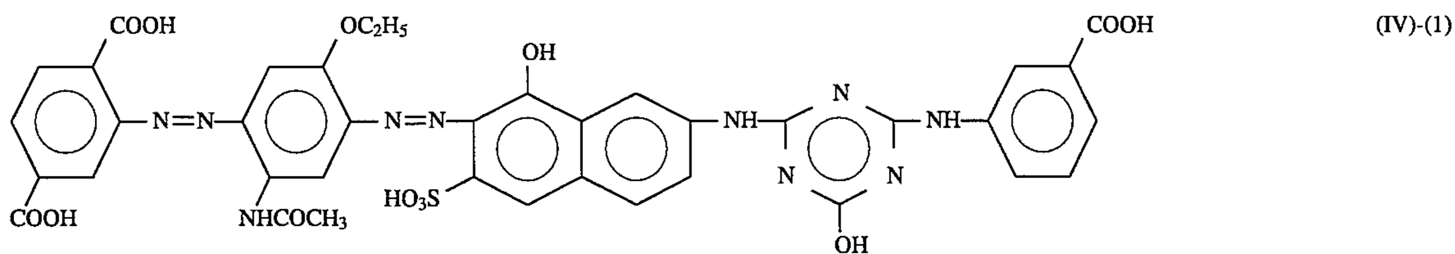
(IV)-(2)
