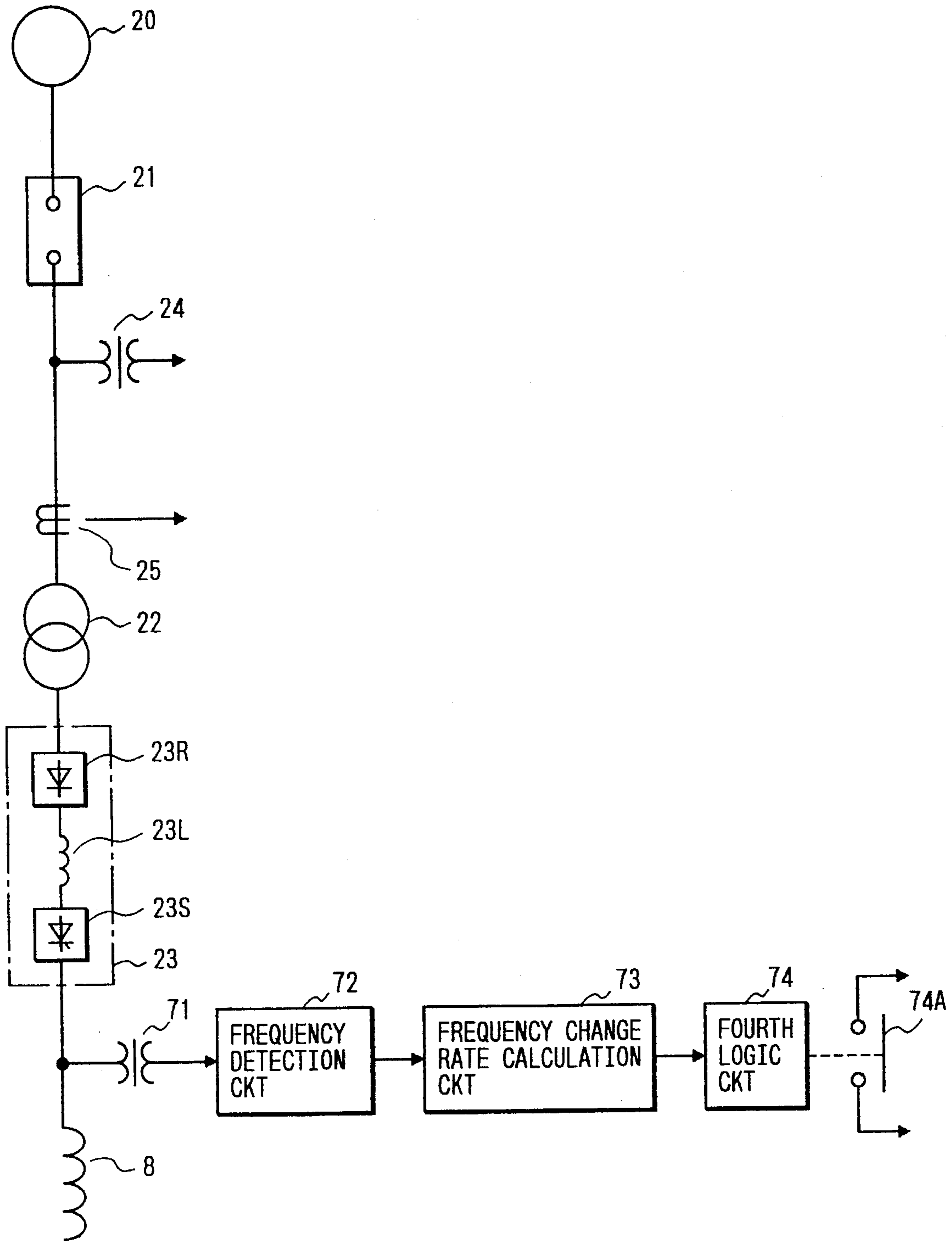
FIG. 12
