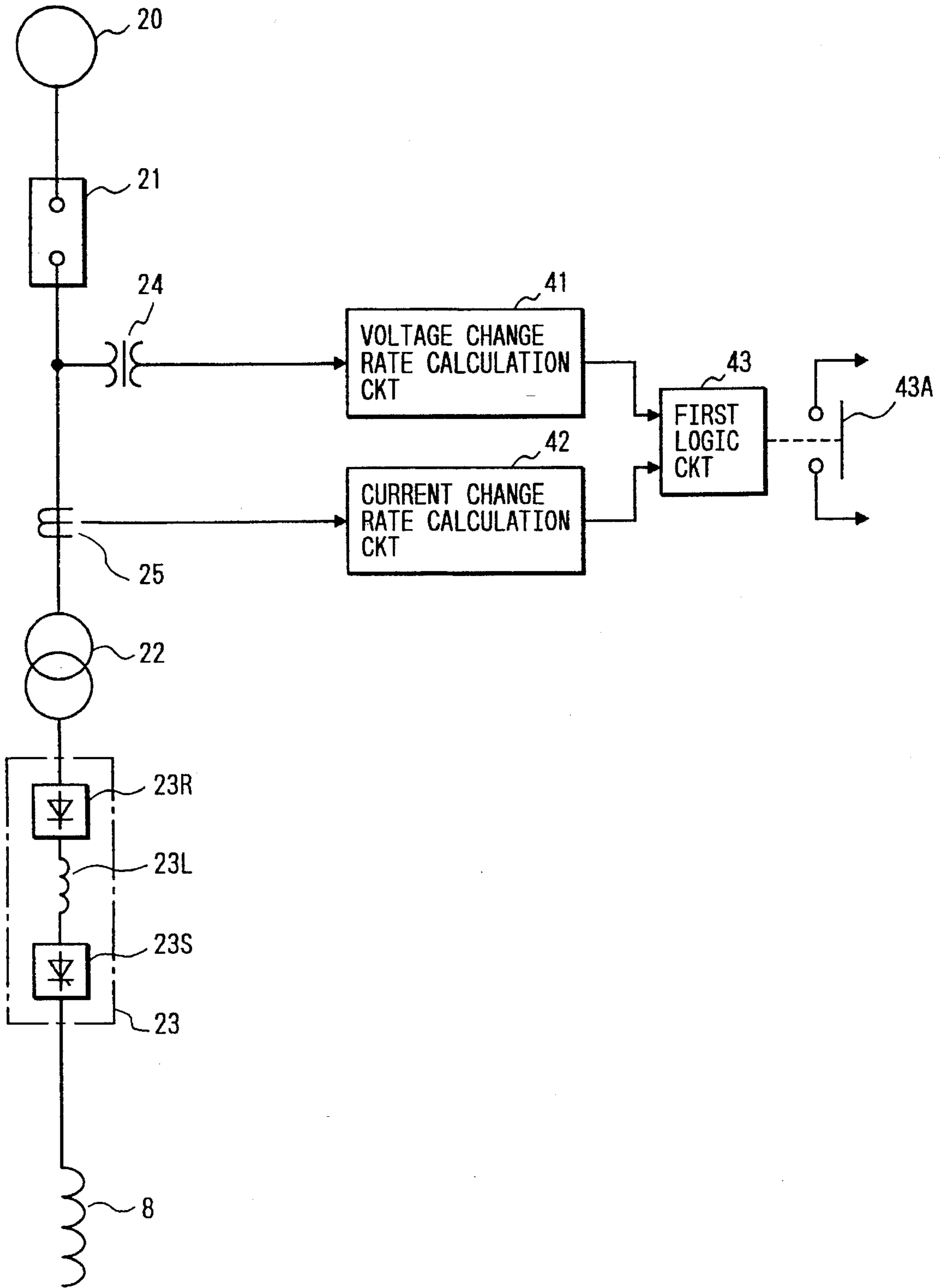
FIG. 5
