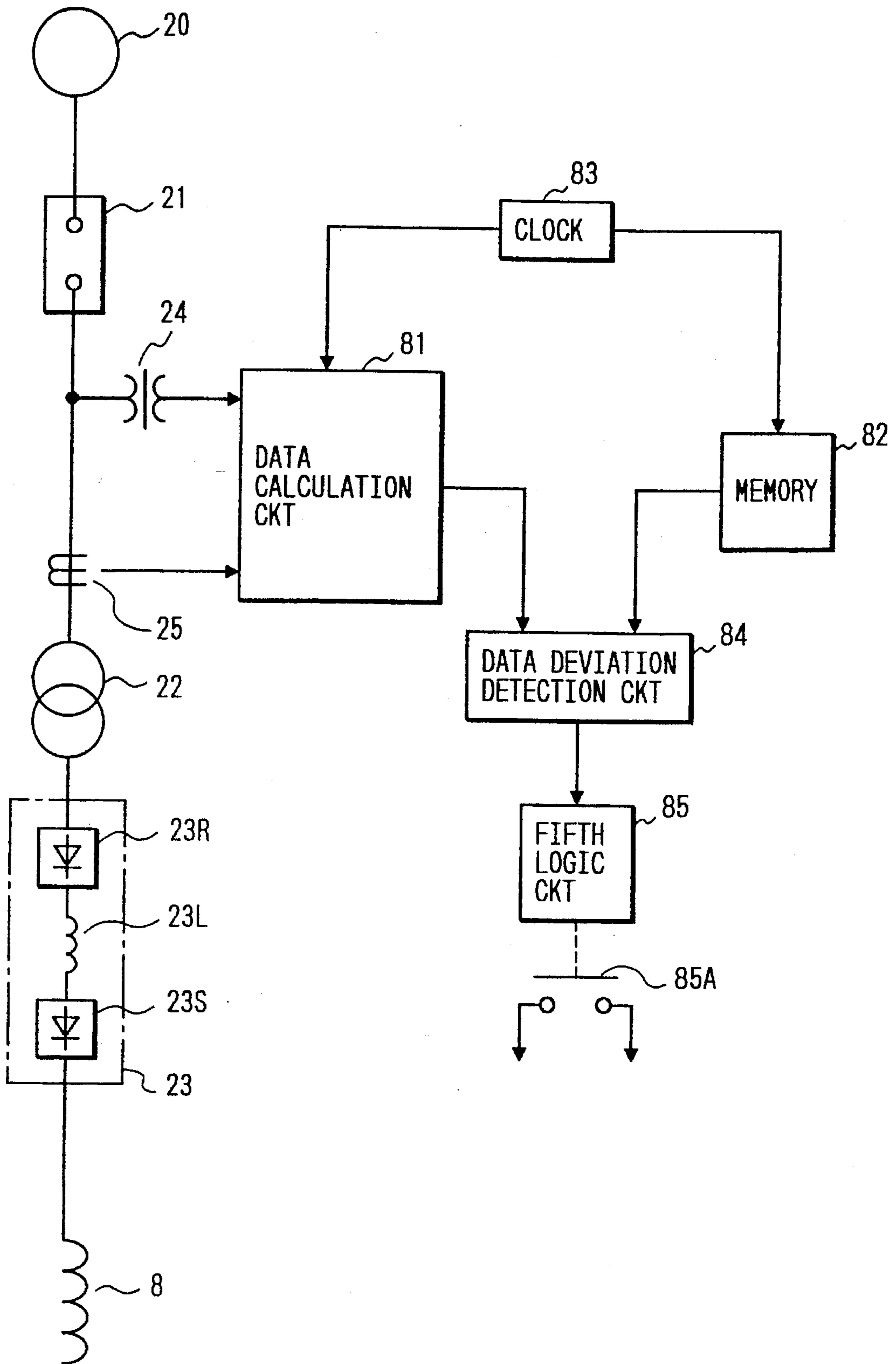
FIG. 13
