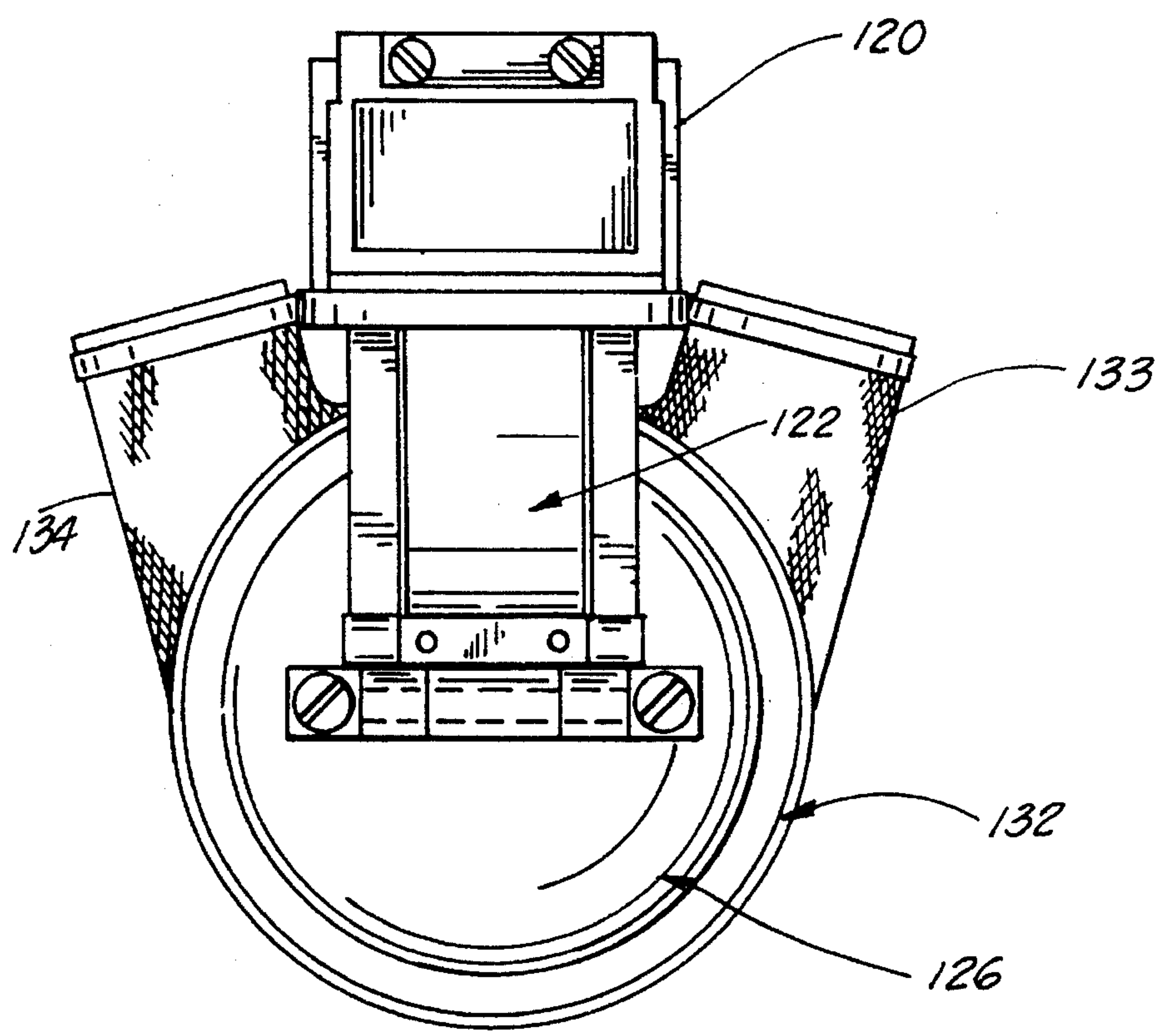
FIG. 9A
