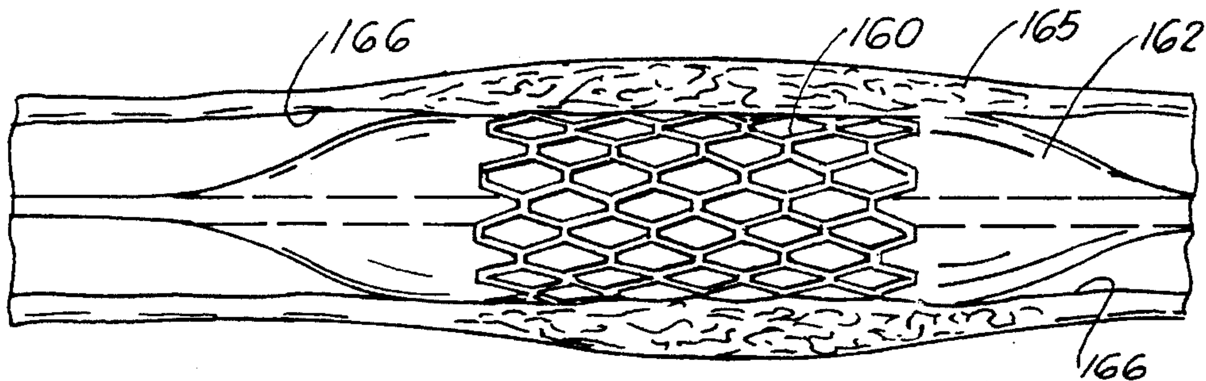
FIG. 11B
