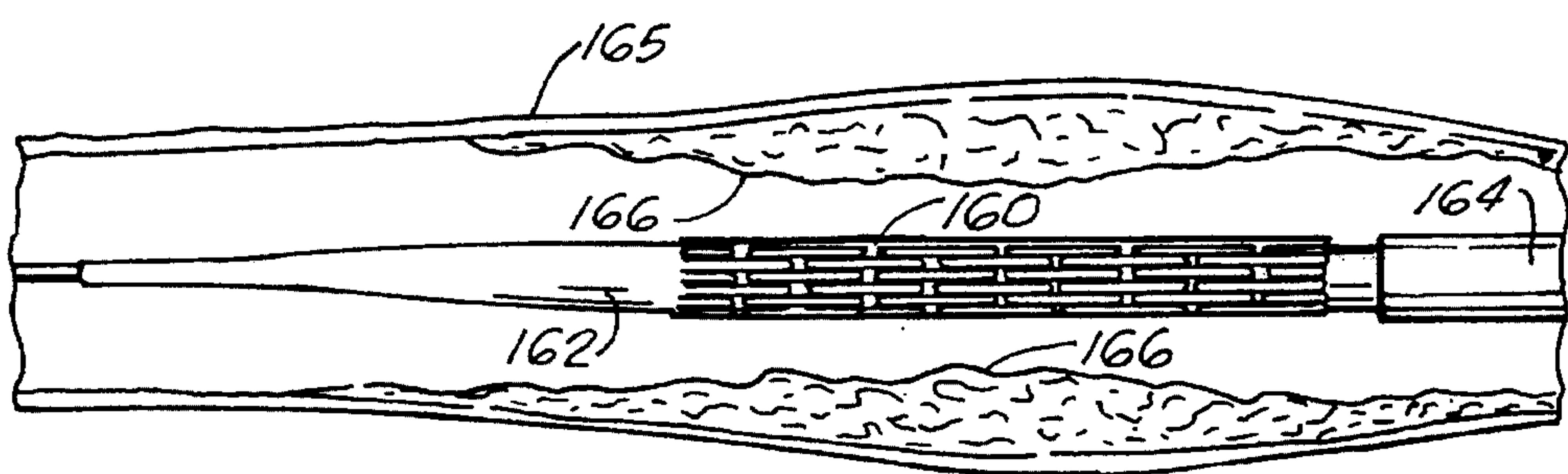
FIG. 11A
