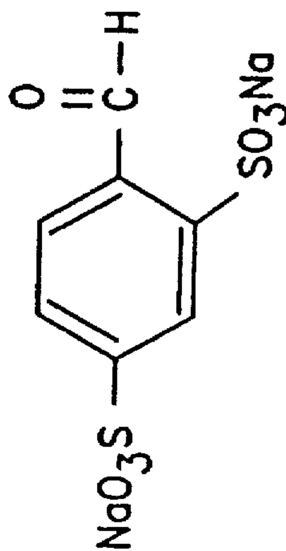
4-Formyl-1,3-benzenesulfonic Acid
