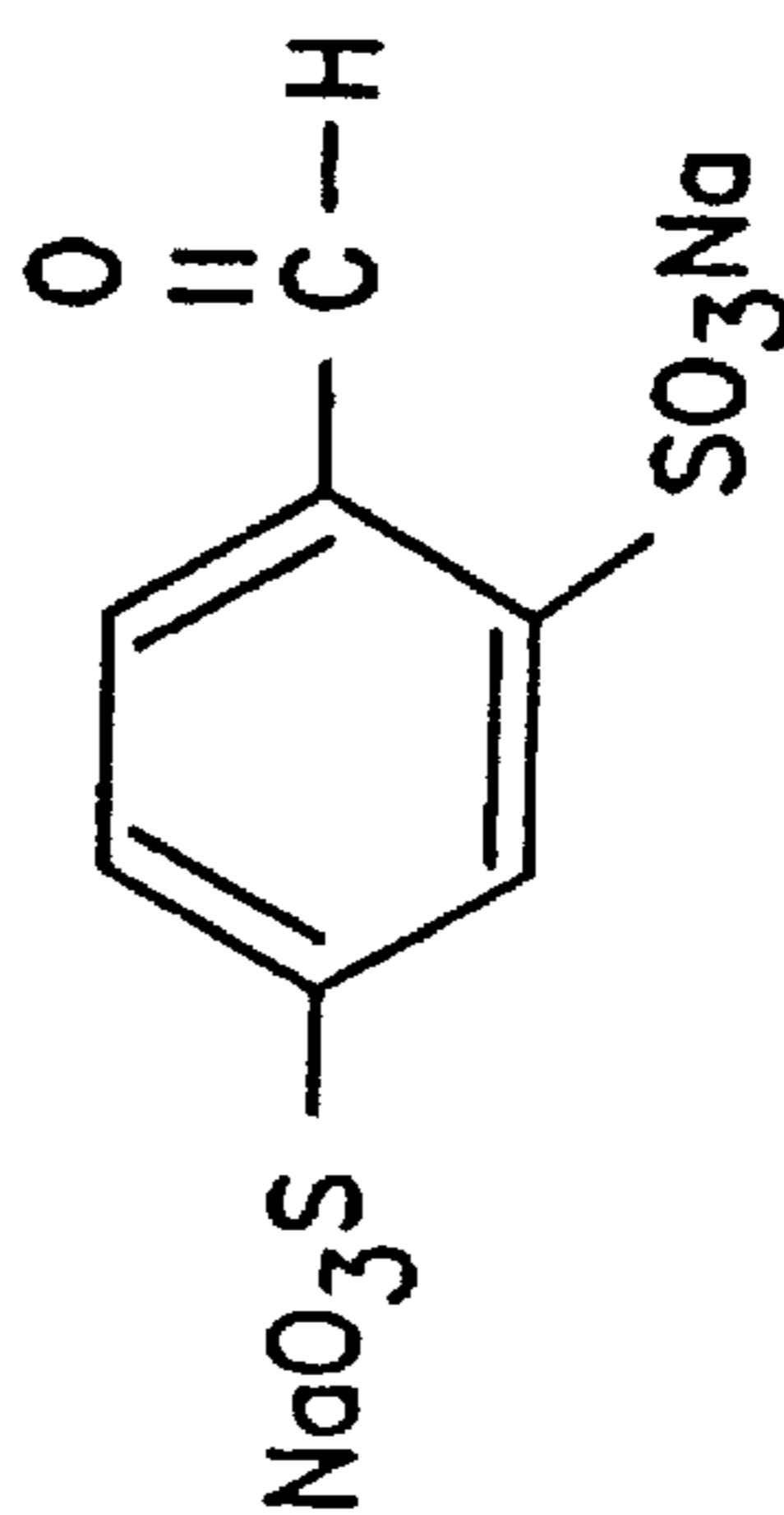
4-Formyl-1,3-benzenesulfonic Acid
