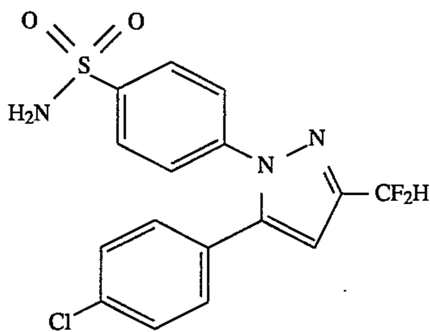
4-[5-(4-Chlorophenyl)-3-(difluoromethyl)-1H-pyrazol-1-yl]benzenesulfonamide
