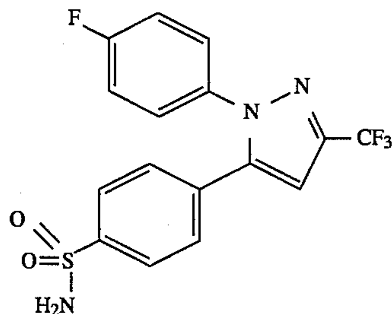
4-[1-(4-Fluorophenyl)-3-(trifluoromethyl)-1H-pyrazol-5-yl]benzenesulfonamide
