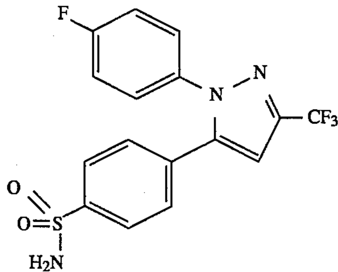
4-[1-(4-Fluorophenyl)-3-(trifluoromethyl)-1H-pyrazol-5-yl]benzenesulfonamide
