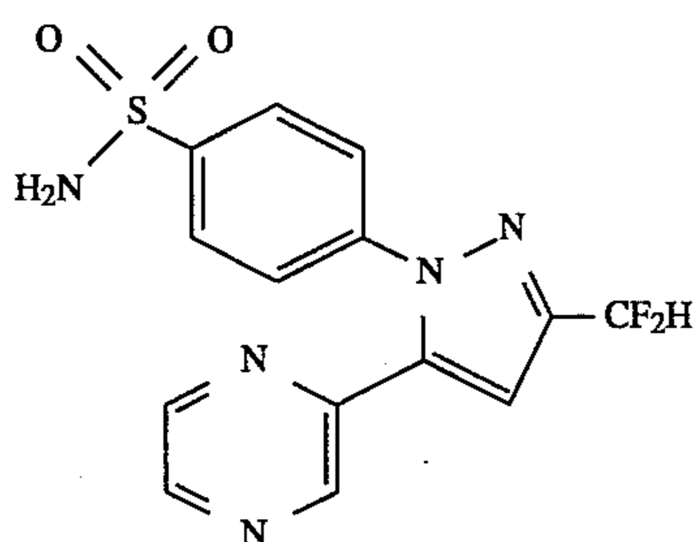
4-[5-(4-Pyrazinyl)-3-(difluoromethyl)-1H-pyrazol-1-yl]benzenesulfonamide
