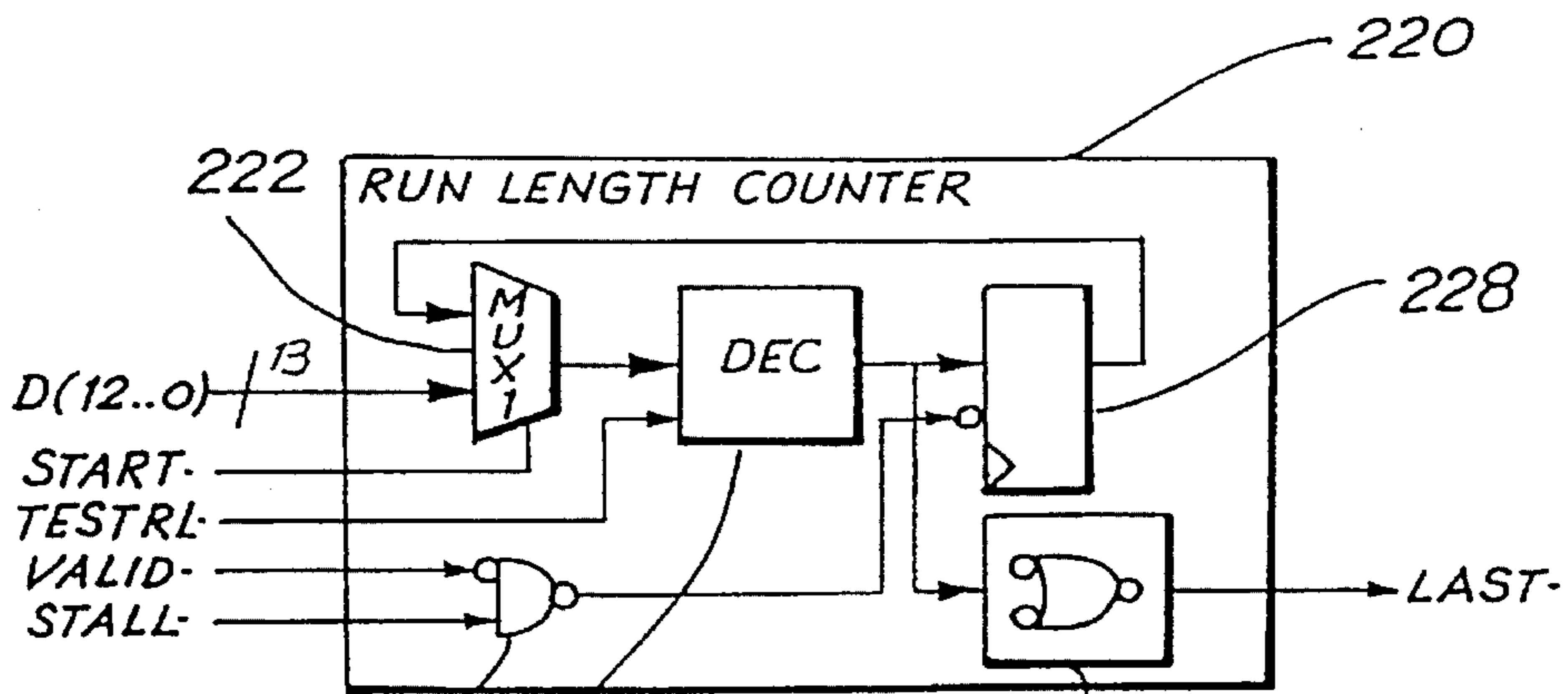
FIG.9
