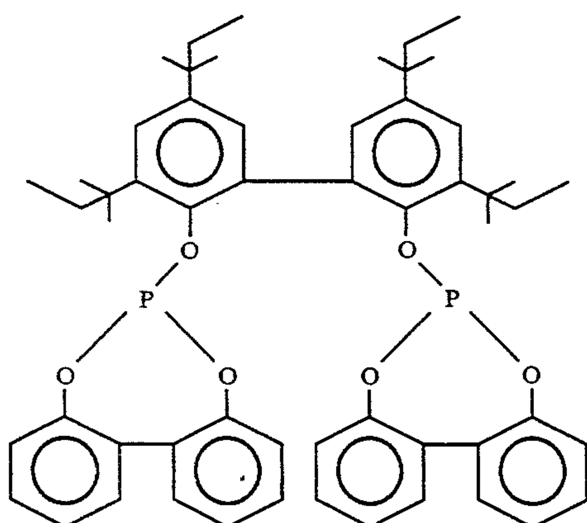
LIGAND I
