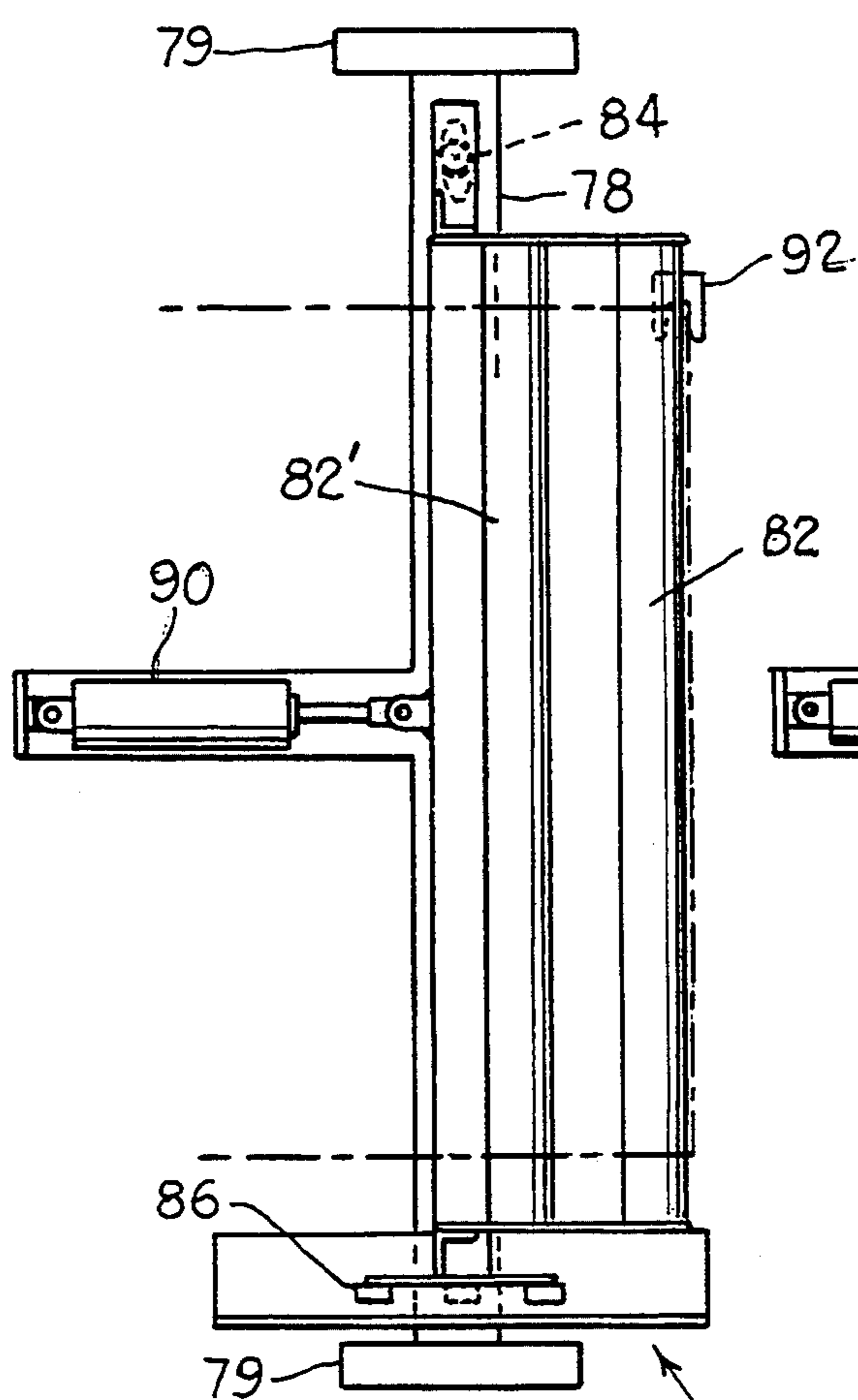
Fig. 7.
