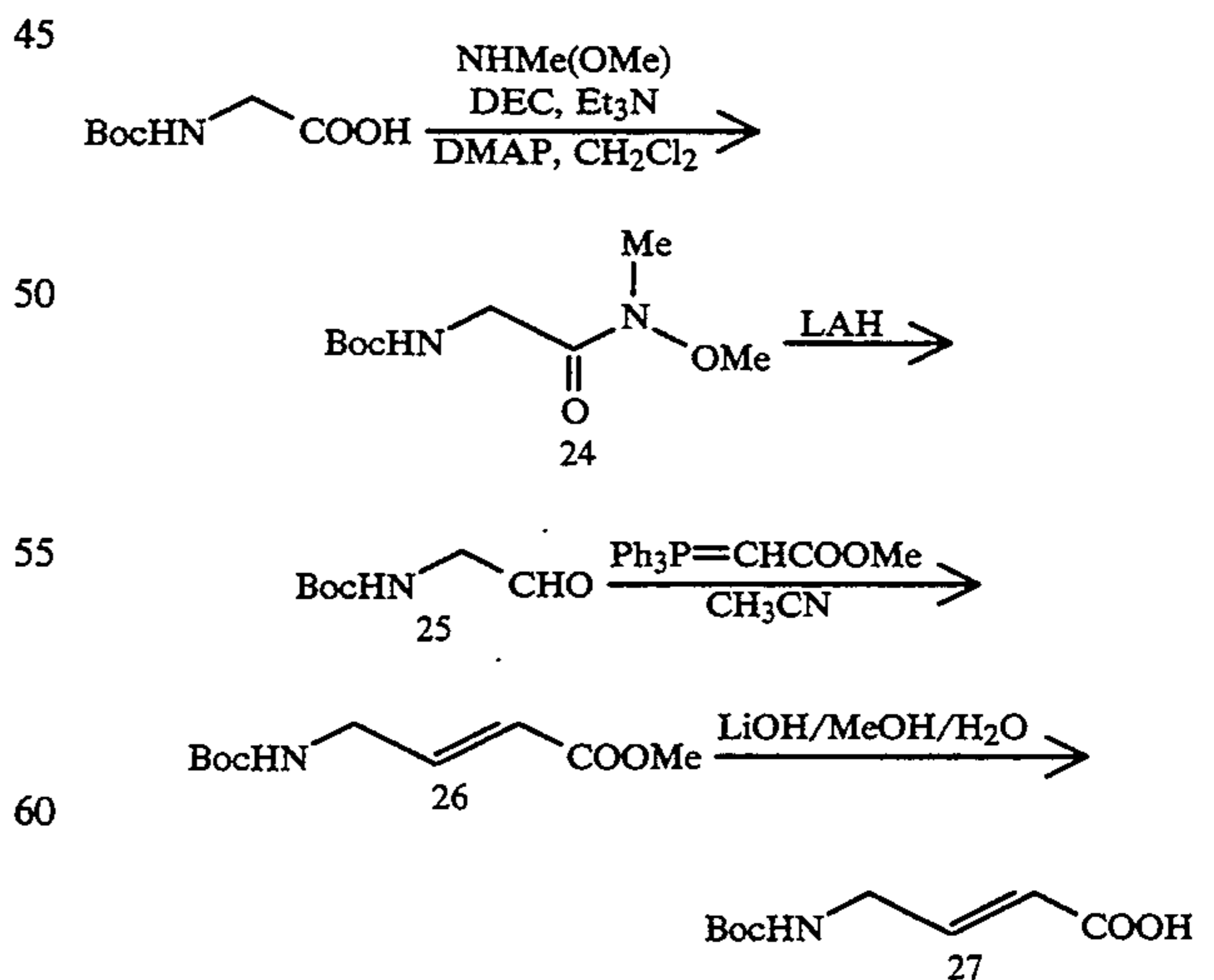
Scheme VI
