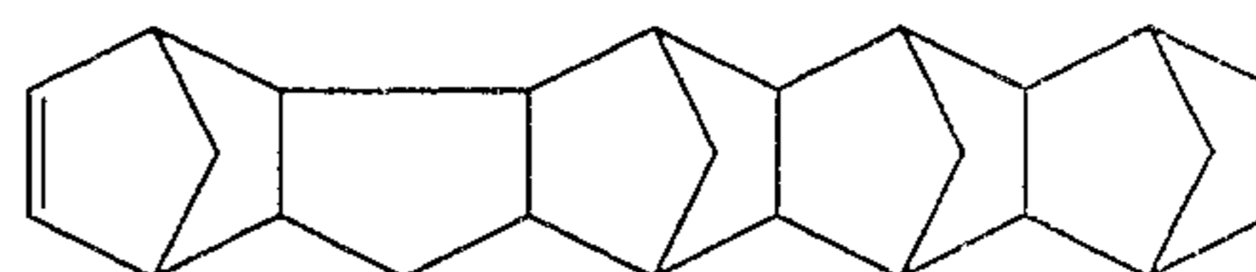
Nonacyclo[9,10,1,1 4,7 ,0 3,8 ,0 2,10 ,0 12,21 ,1 13,20 ,0 14,19 ,1 15,18 ]-5-pentacosene
