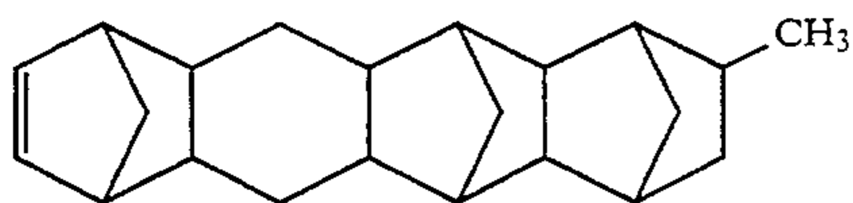
15-Methylheptacyclo[8,8,0,1 4,7 ,1 11,18 ,1 13,16 ,0 3,8 ,0 12,17 ]-5-heneicosene
