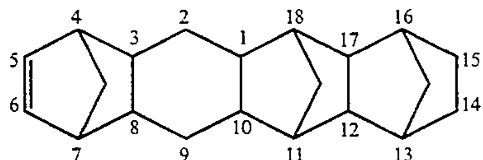
Heptacyclo[8,8,0,1 4,7 ,1 11,18 ,1 13,16 ,0 3,8 ,0 12,17 ]-5-heneicosene
