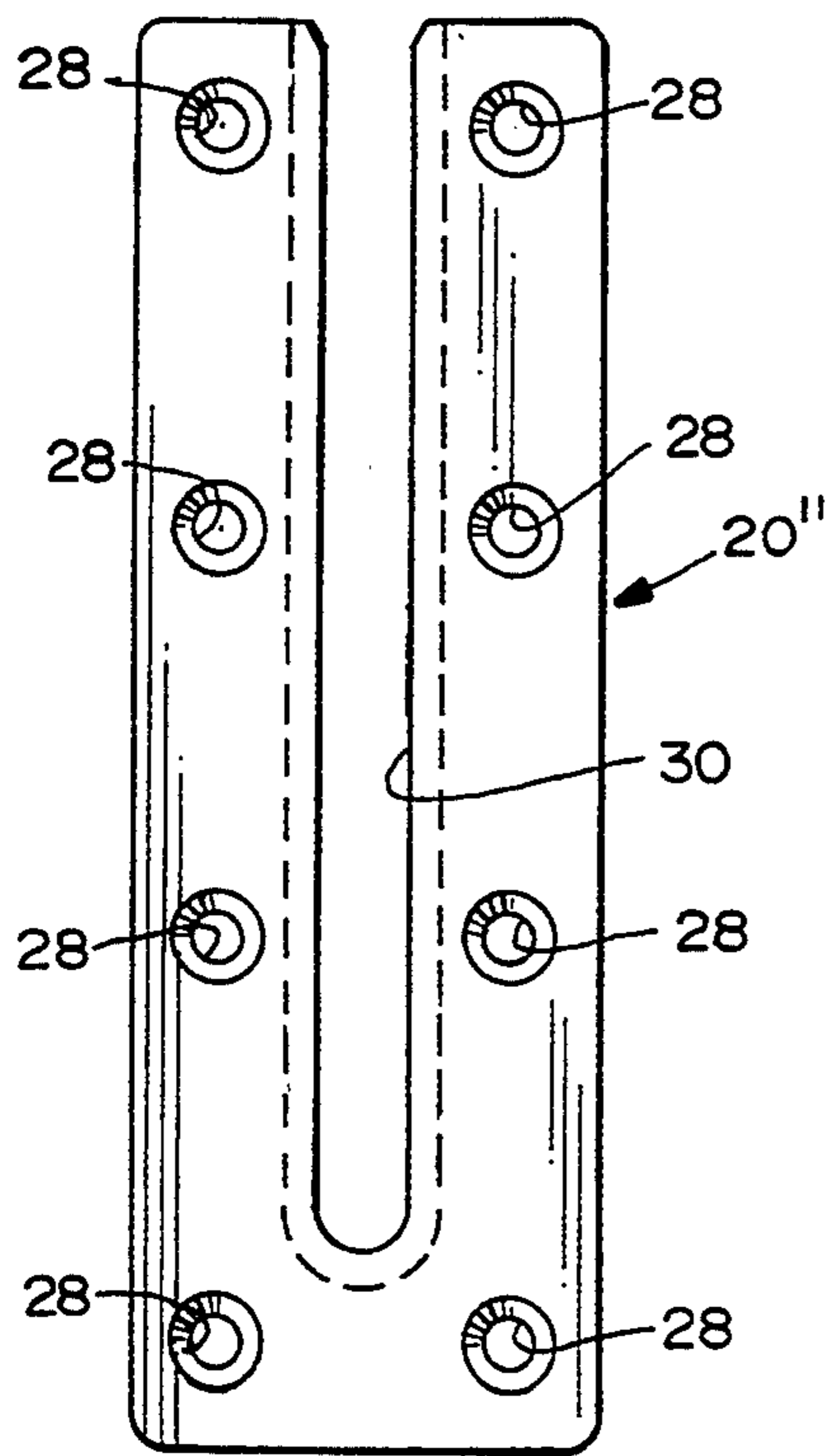
Fig.10
