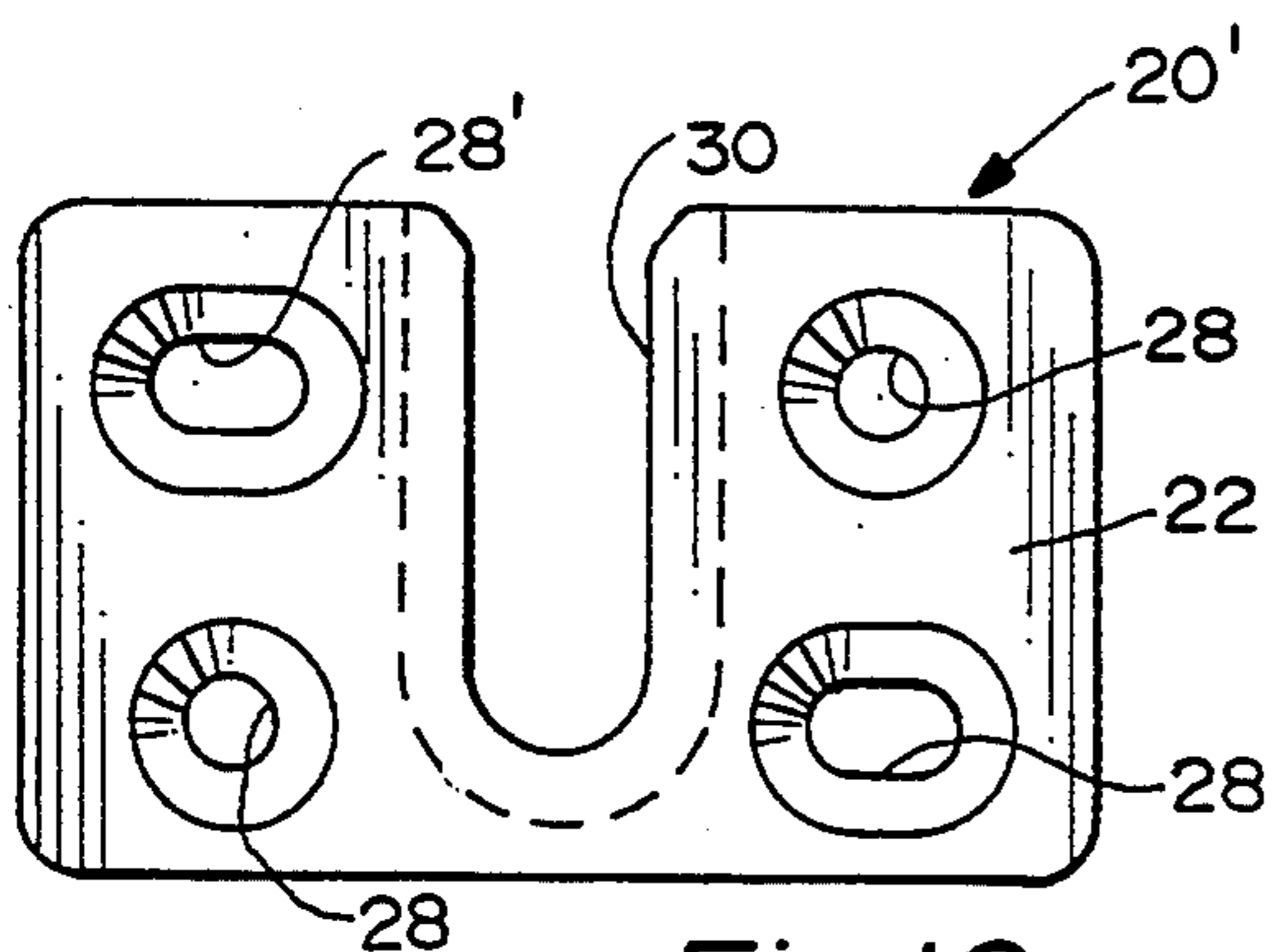
Fig. 16
