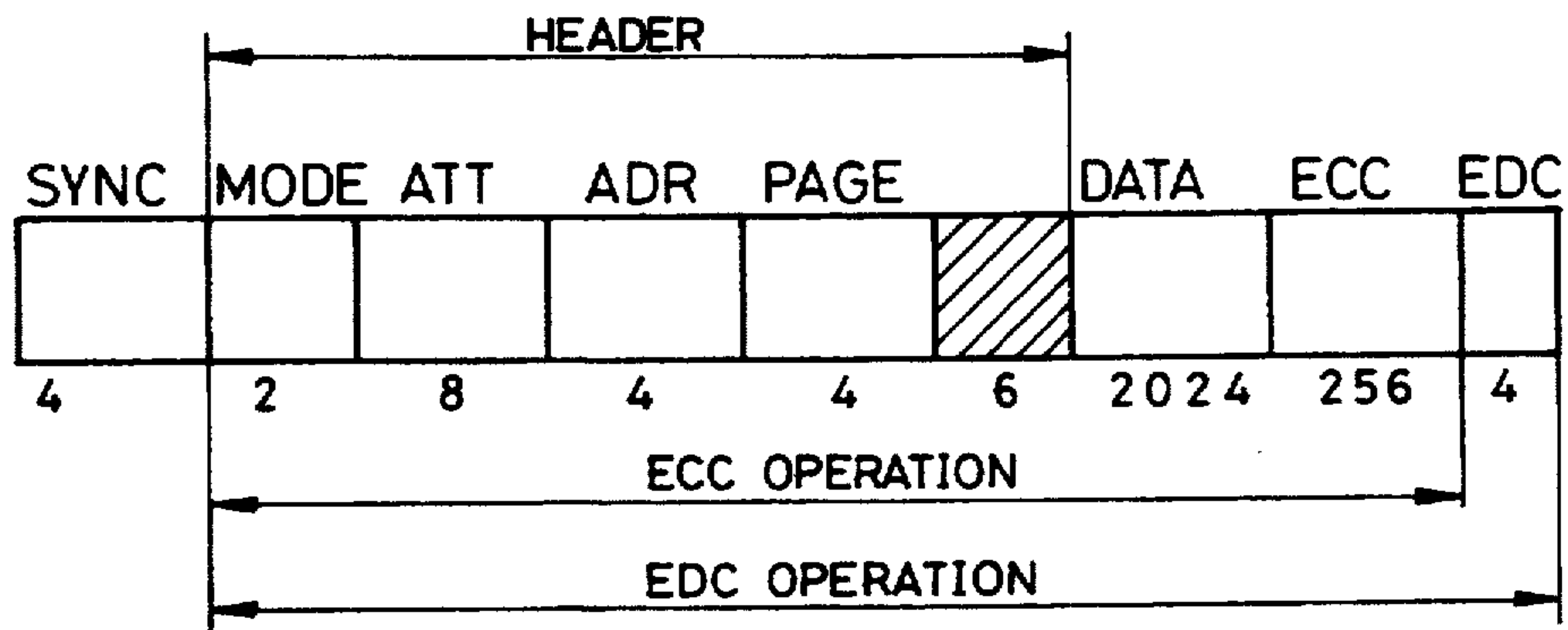
HEADER FORMAT
