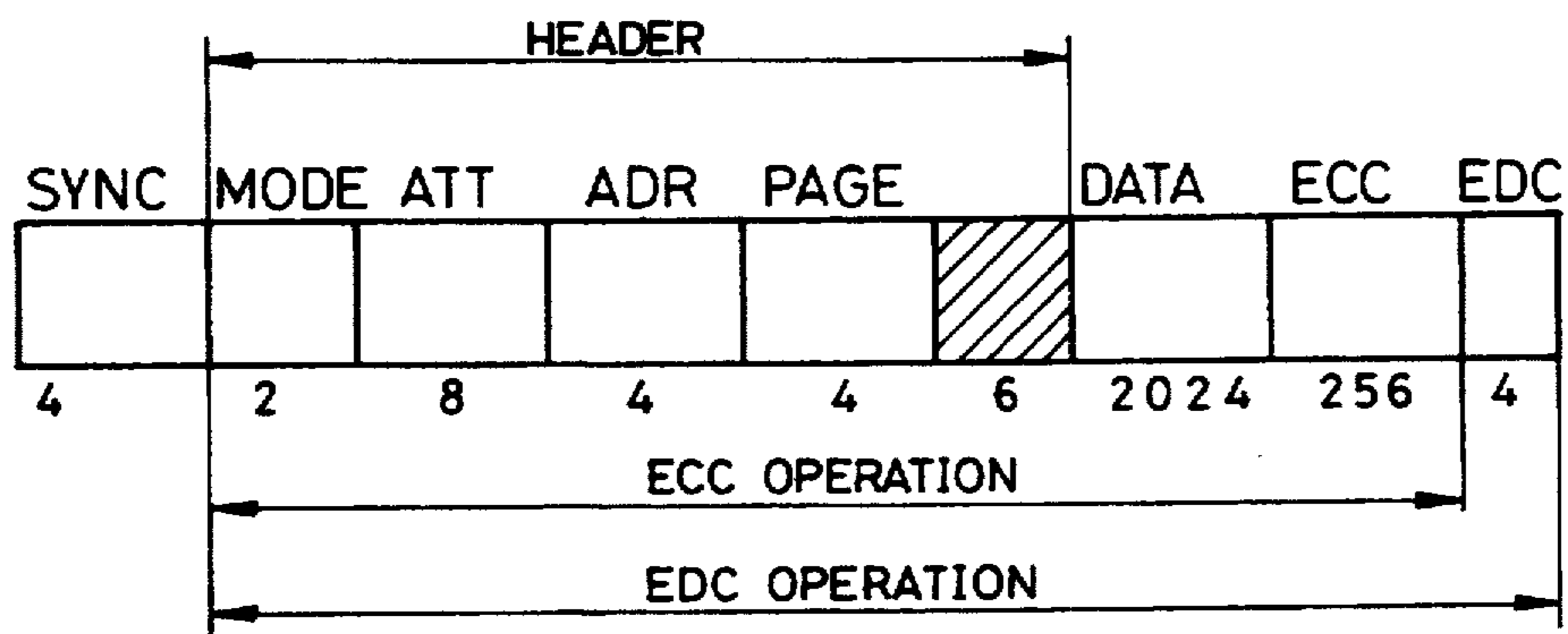
HEADER FORMAT
