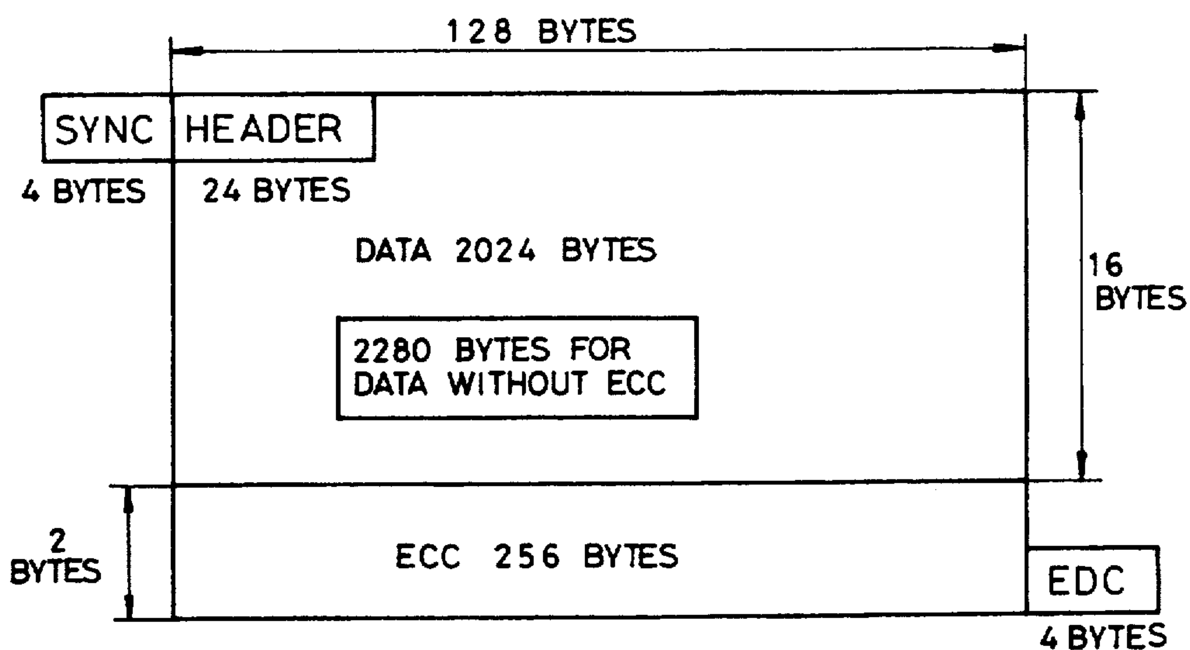
DATA FORMAT
