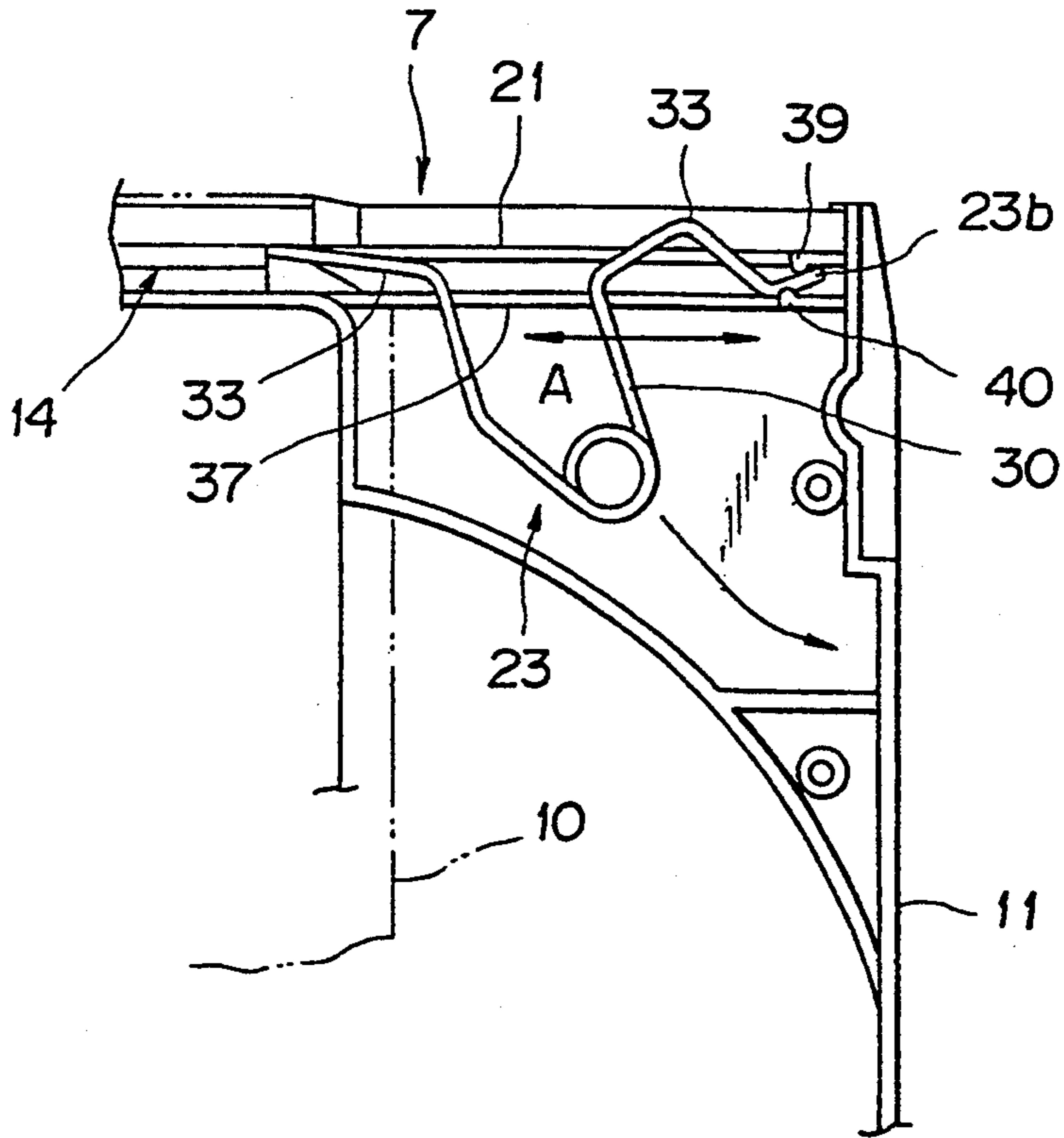
FIG. 18
