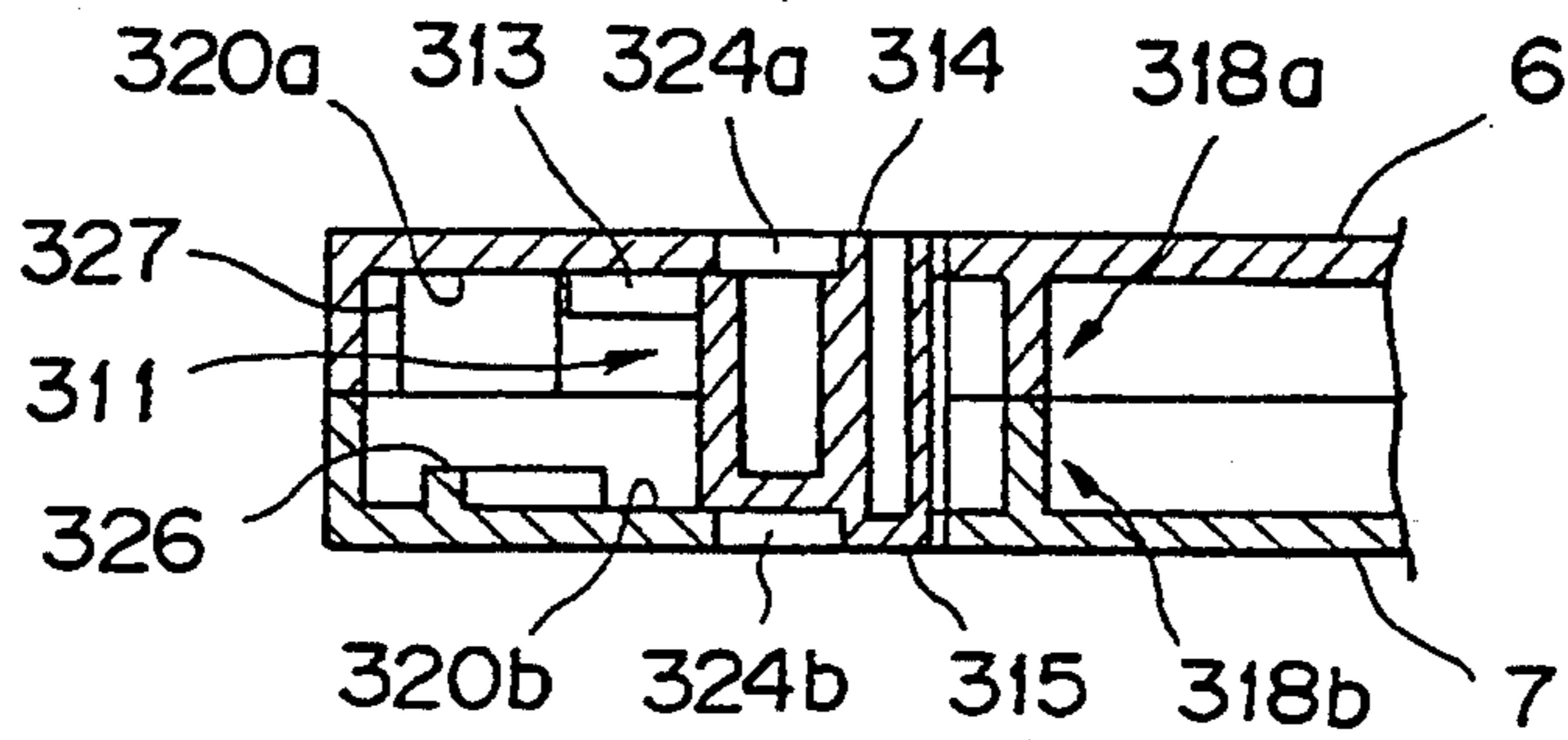
FIG. 52
