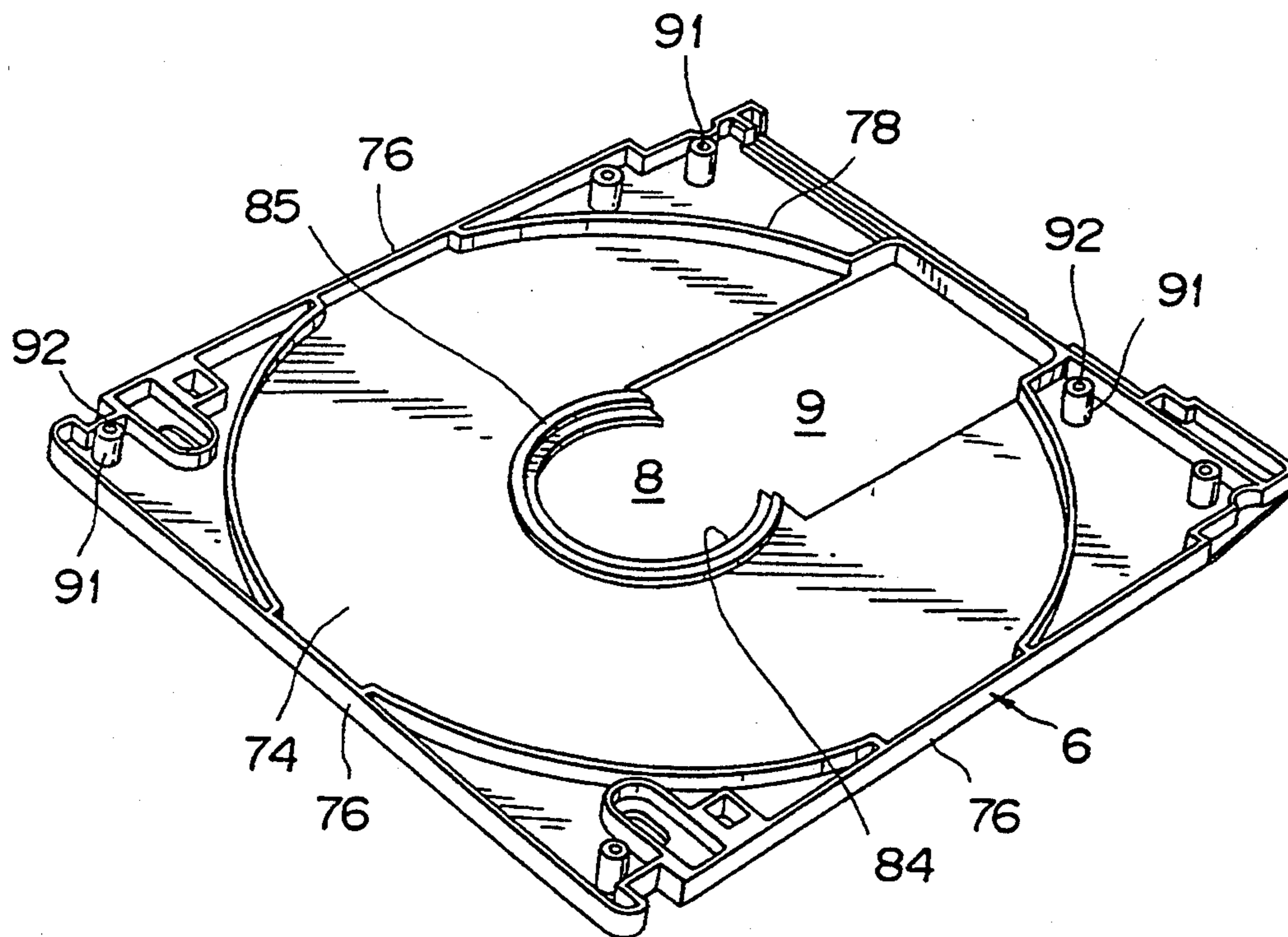
FIG. 33
