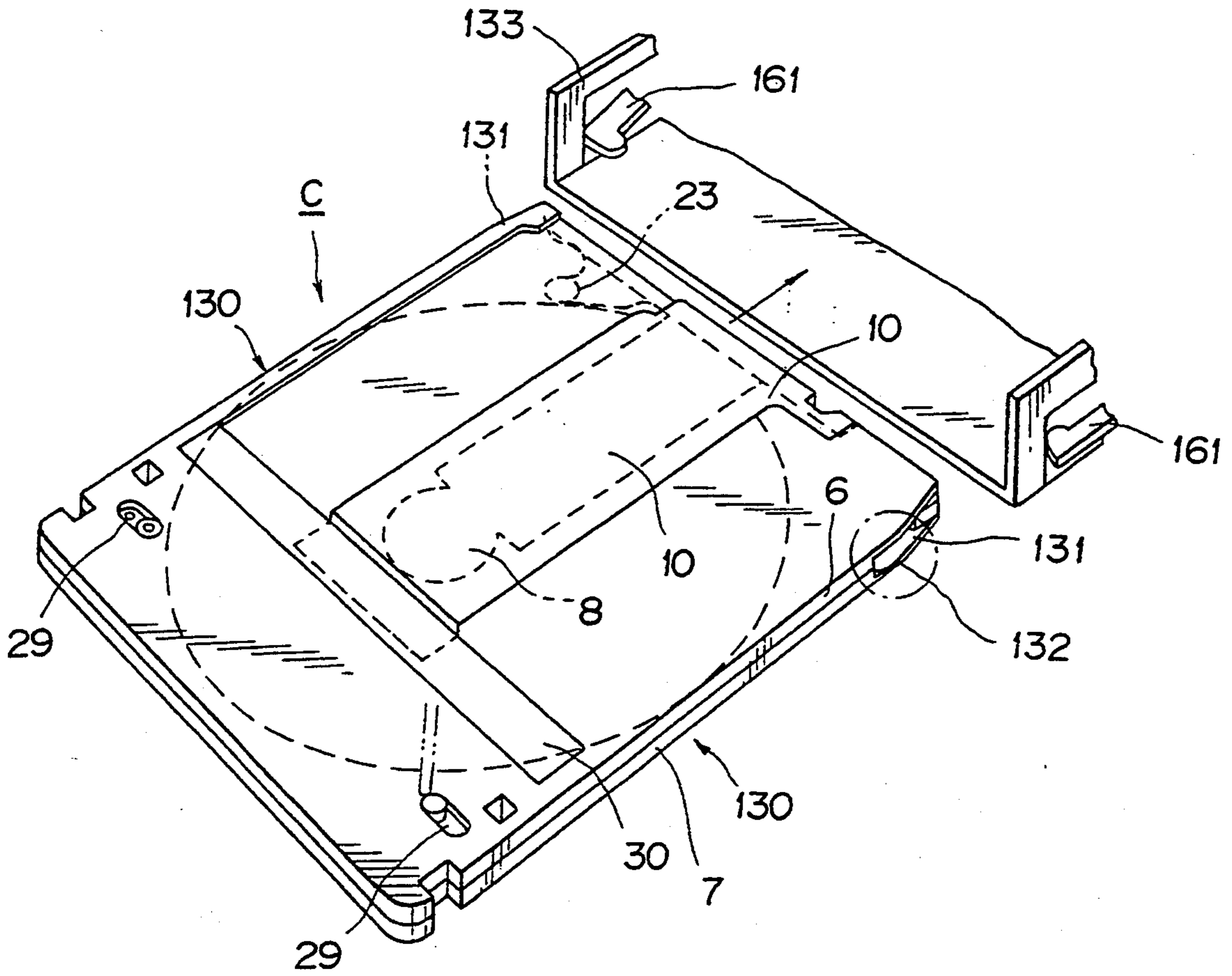
FIG. 45
