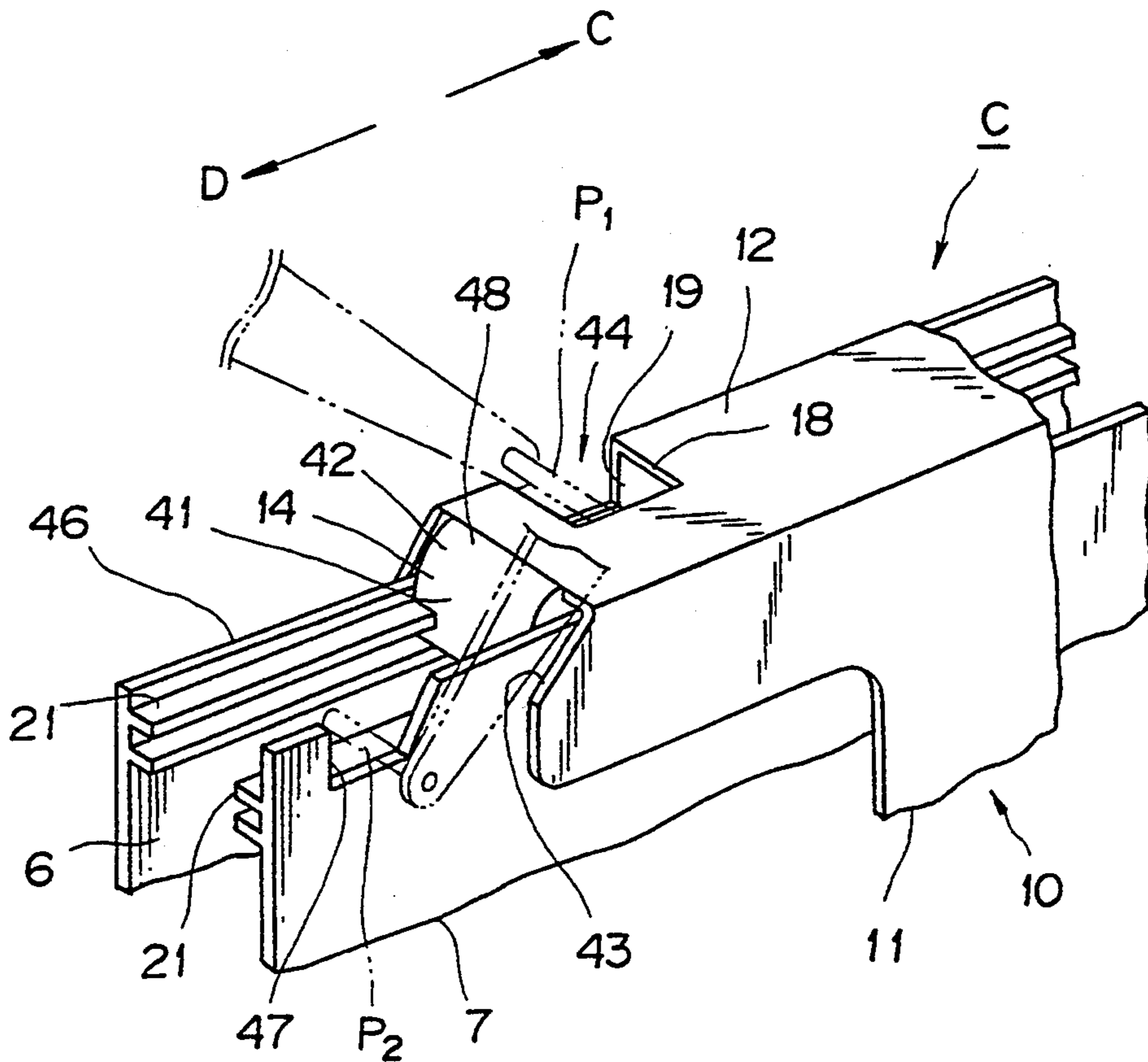
FIG. 21
