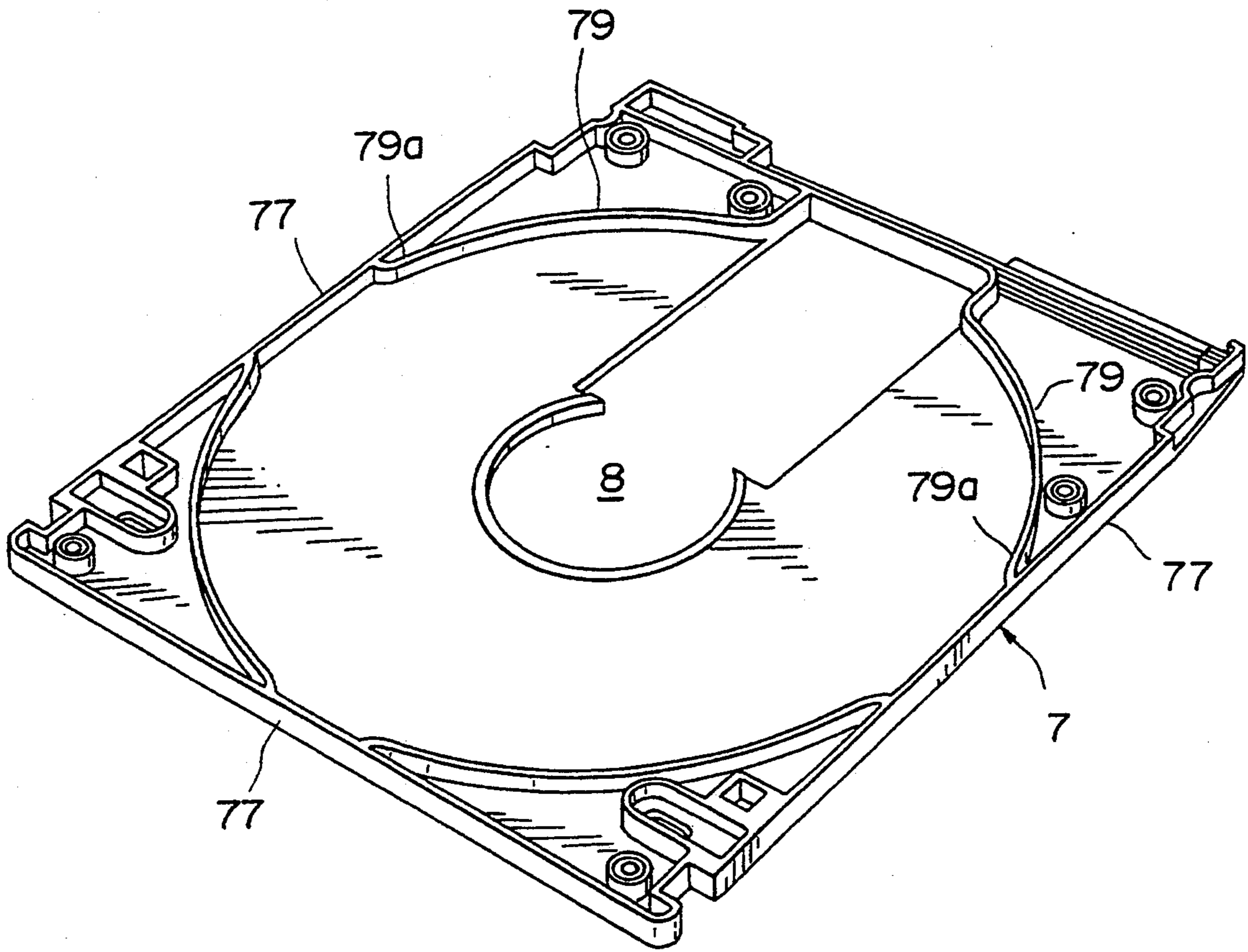
FIG. 42
