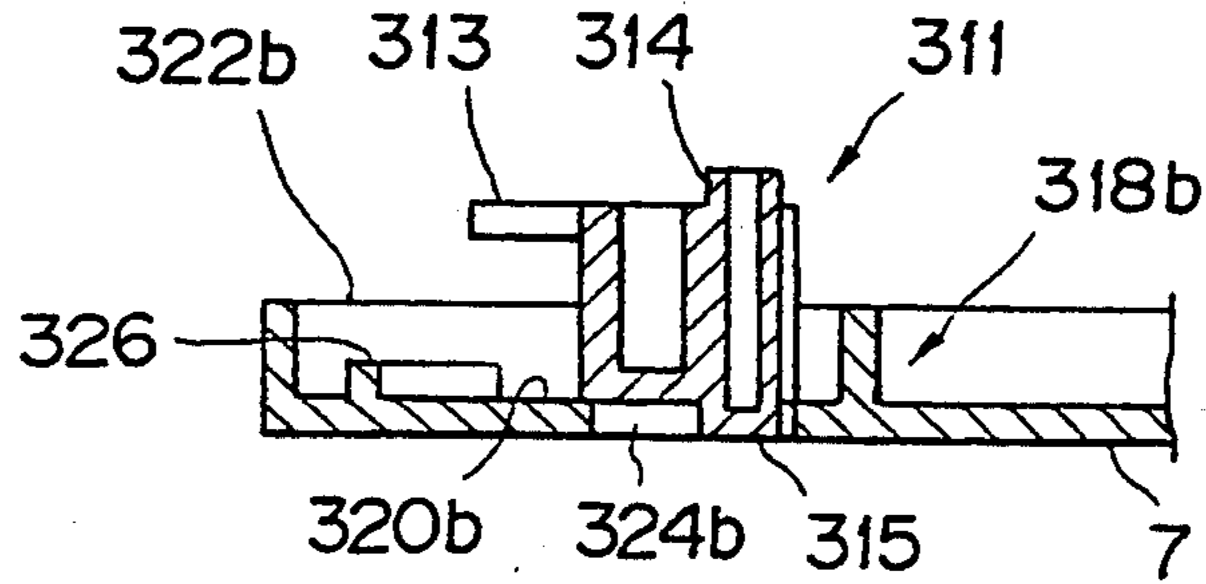
FIG. 51
