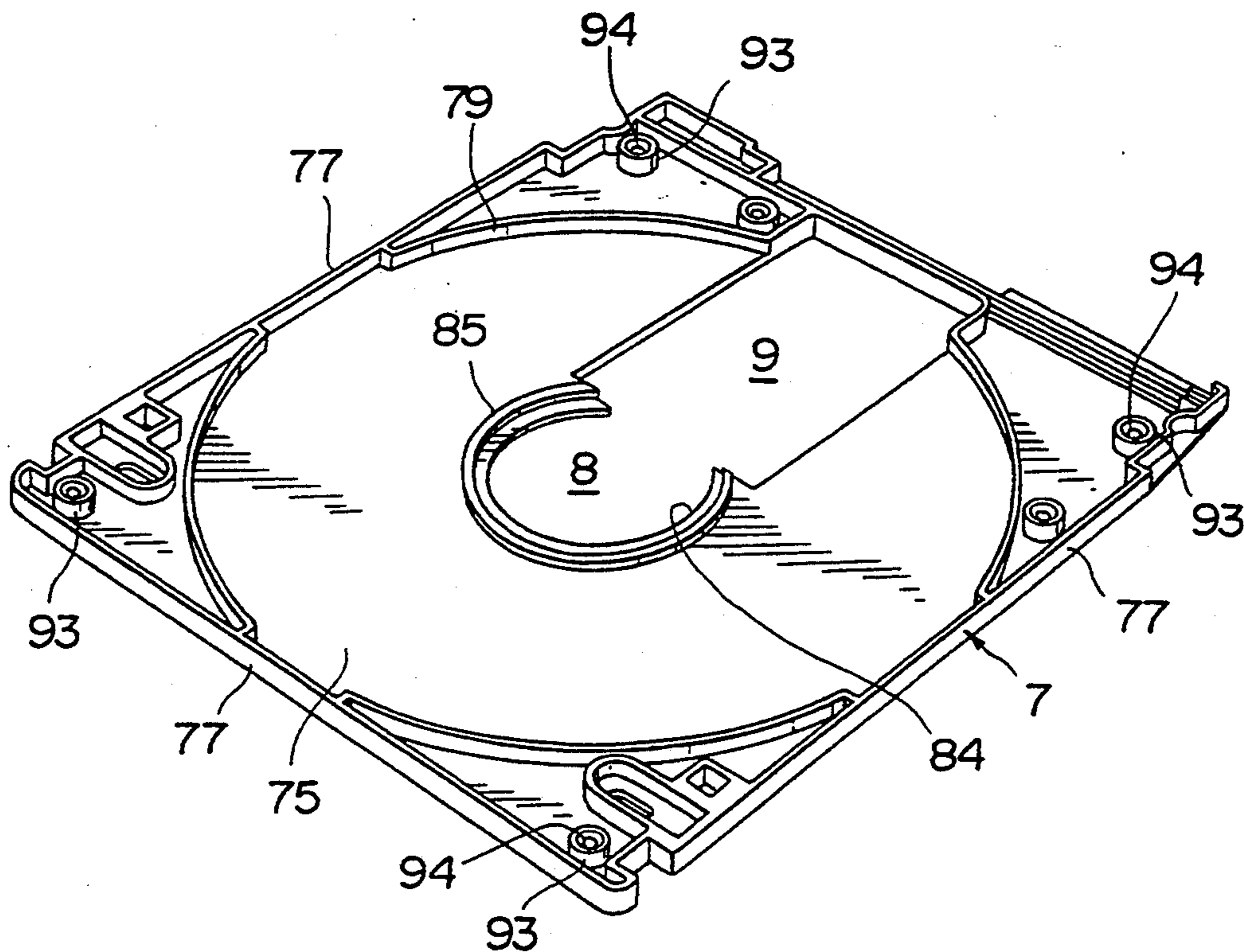
FIG. 34
