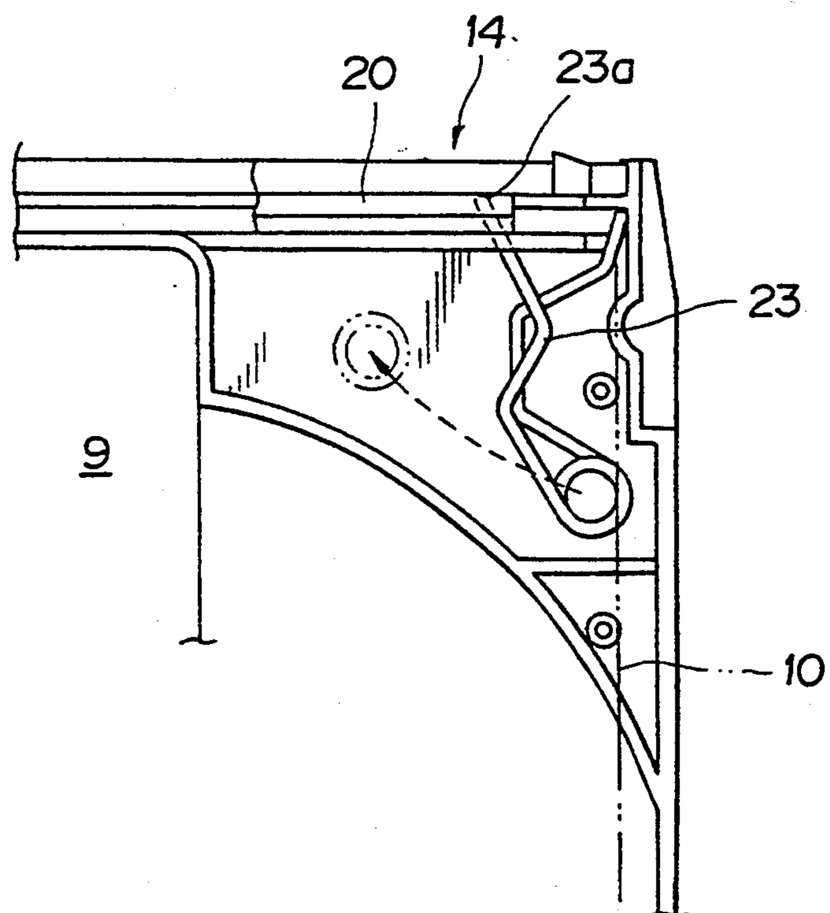
FIG. 6
