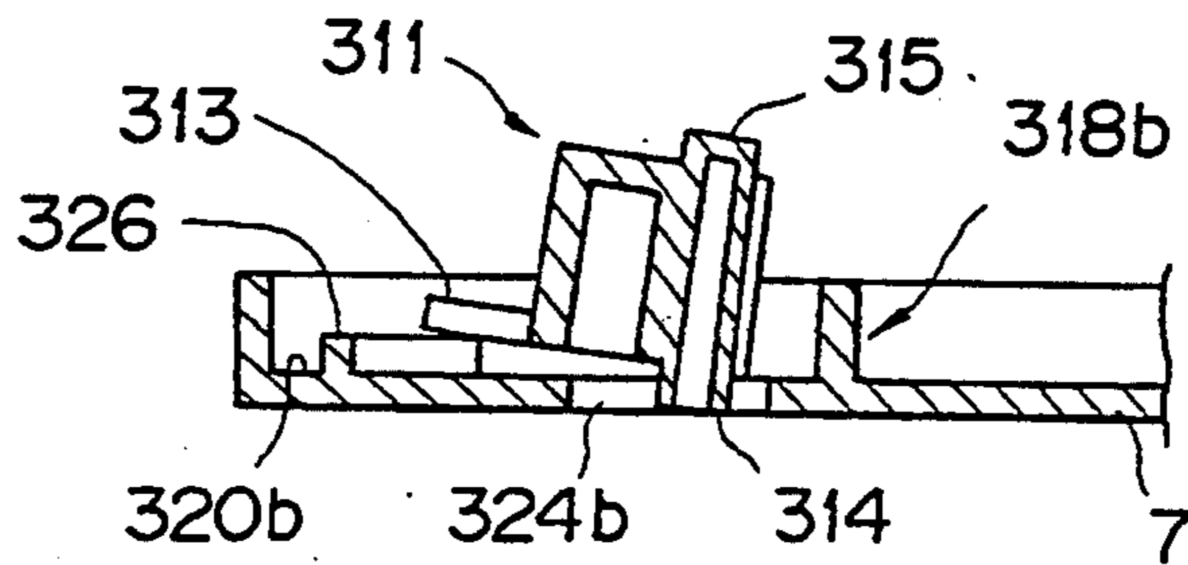
FIG. 53
