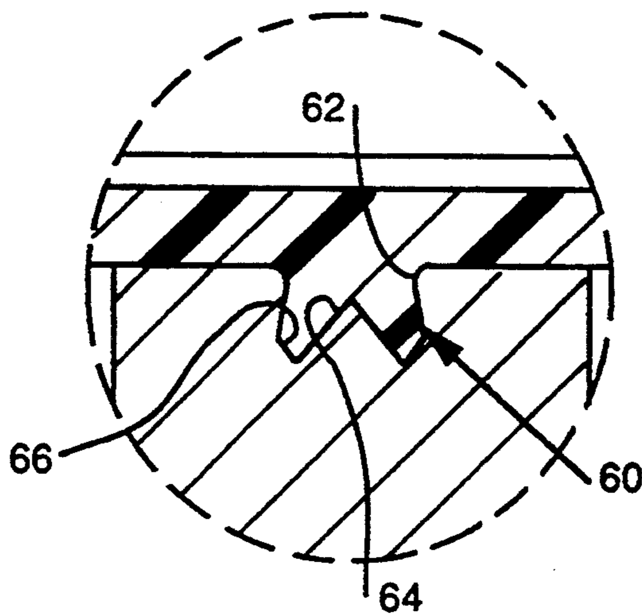
FIG. 4A
