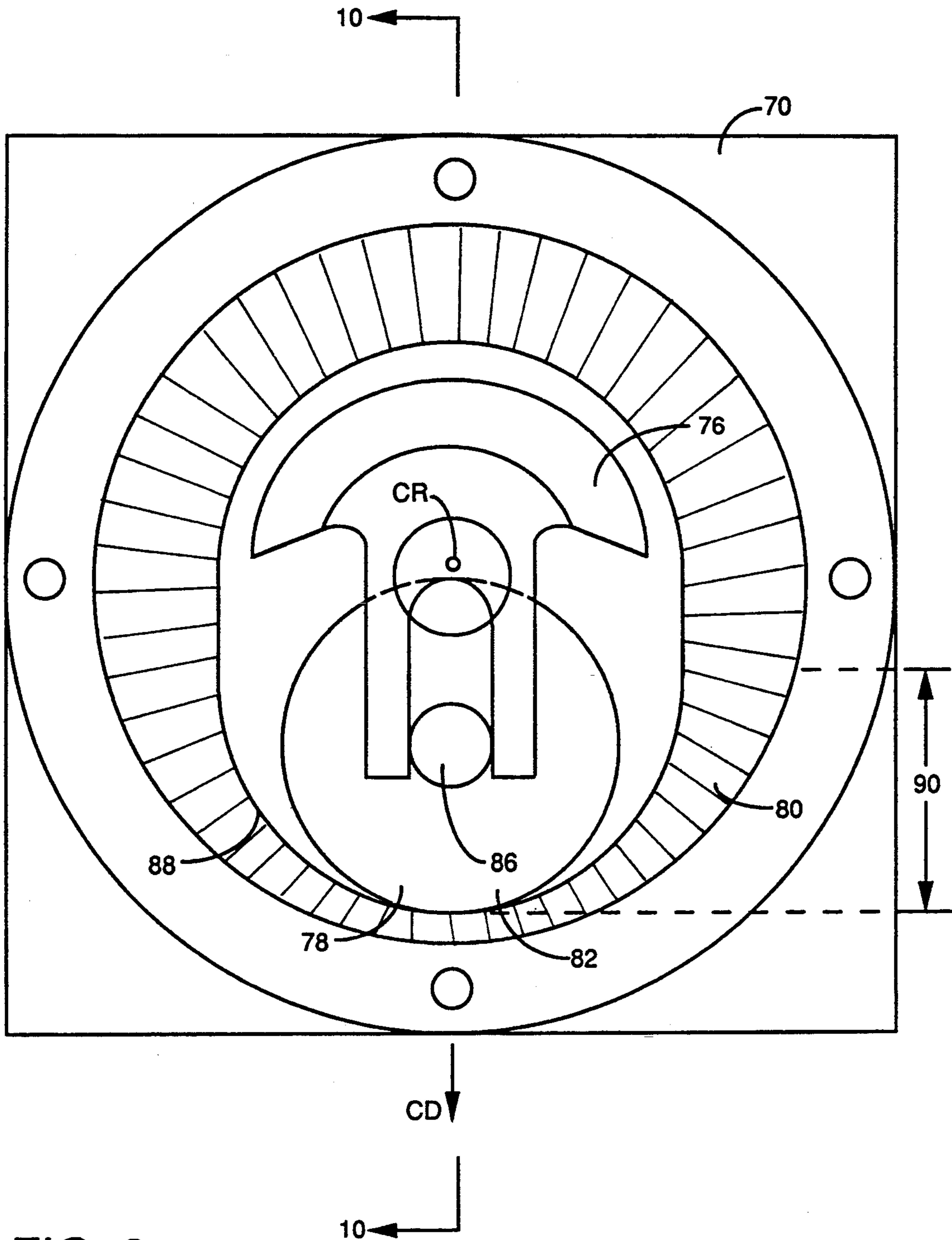
FIG. 9
