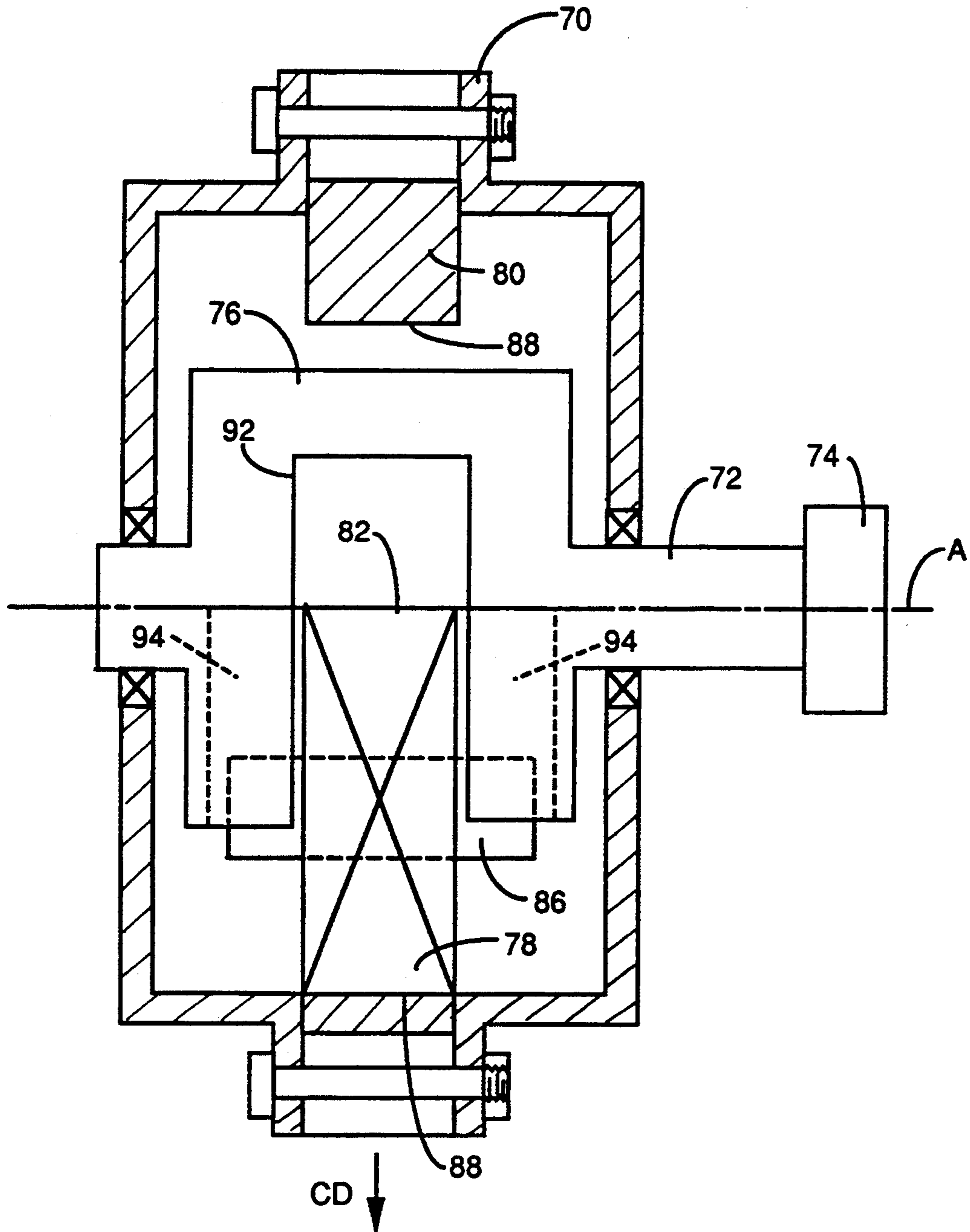
FIG. 10
