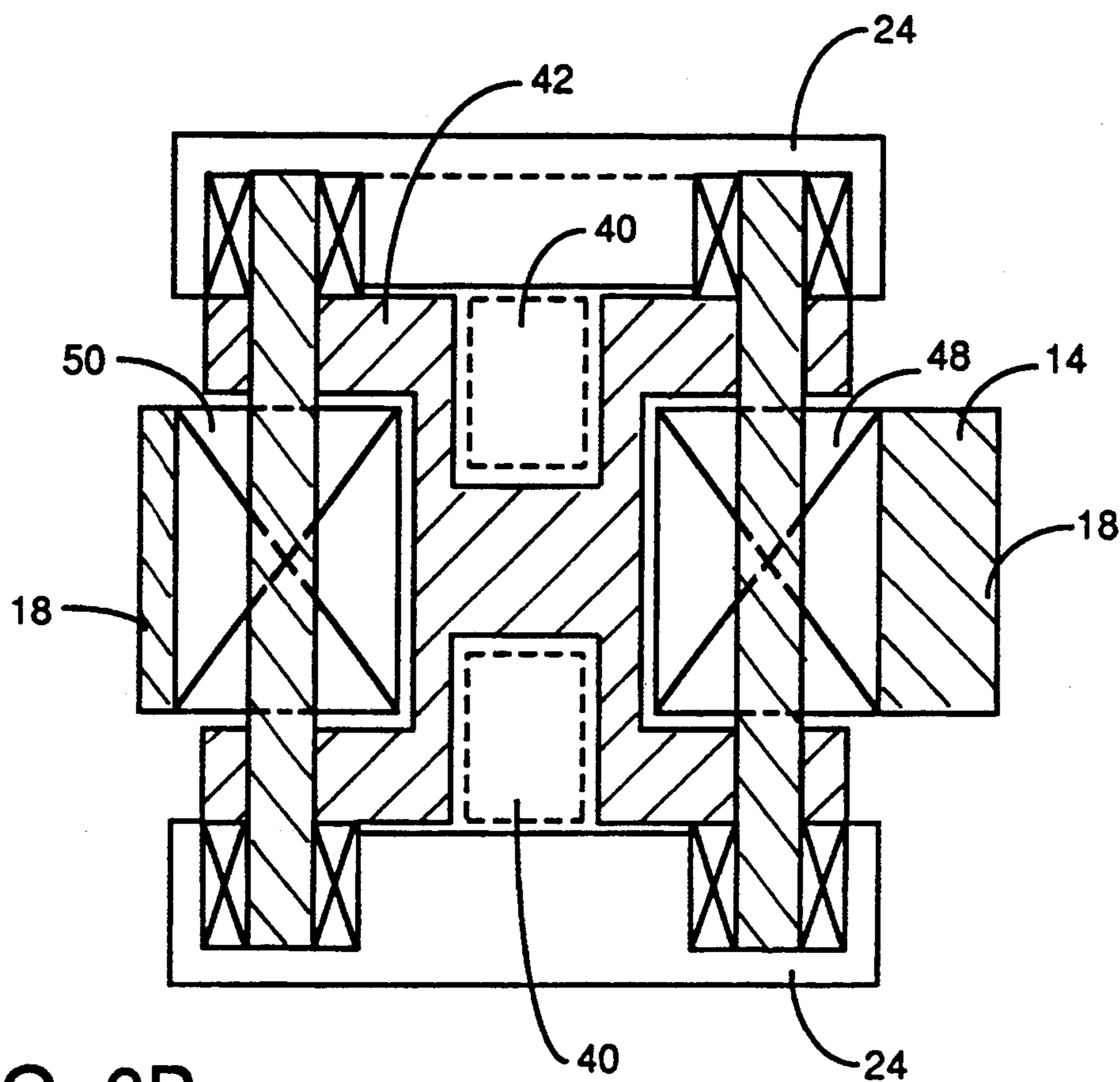
FIG. 6A
