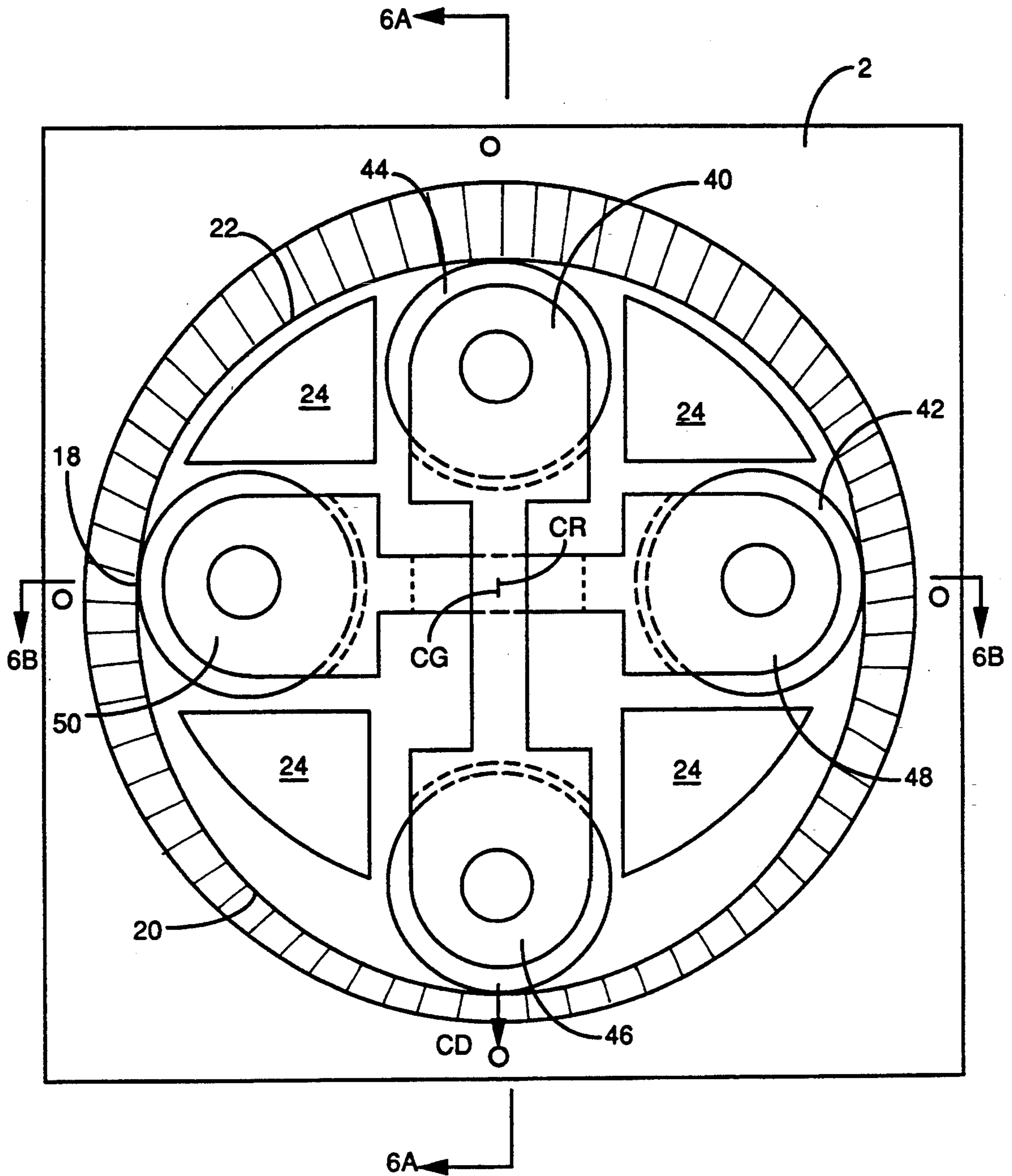
FIG. 5
