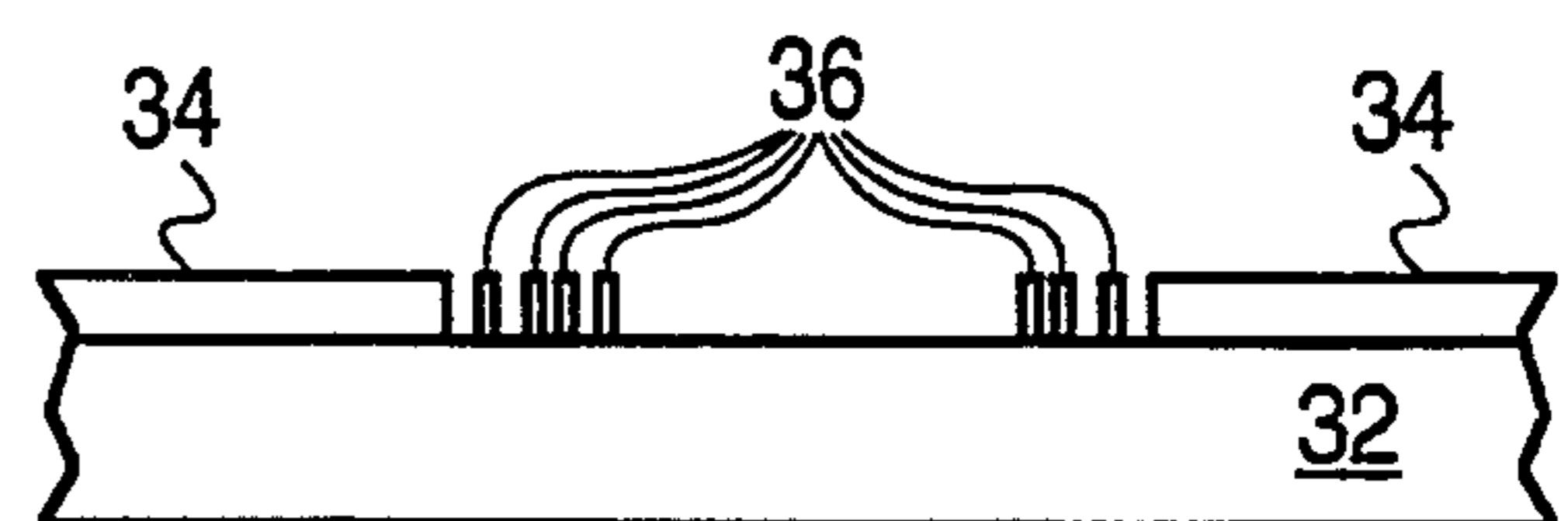
FIG. 3b
