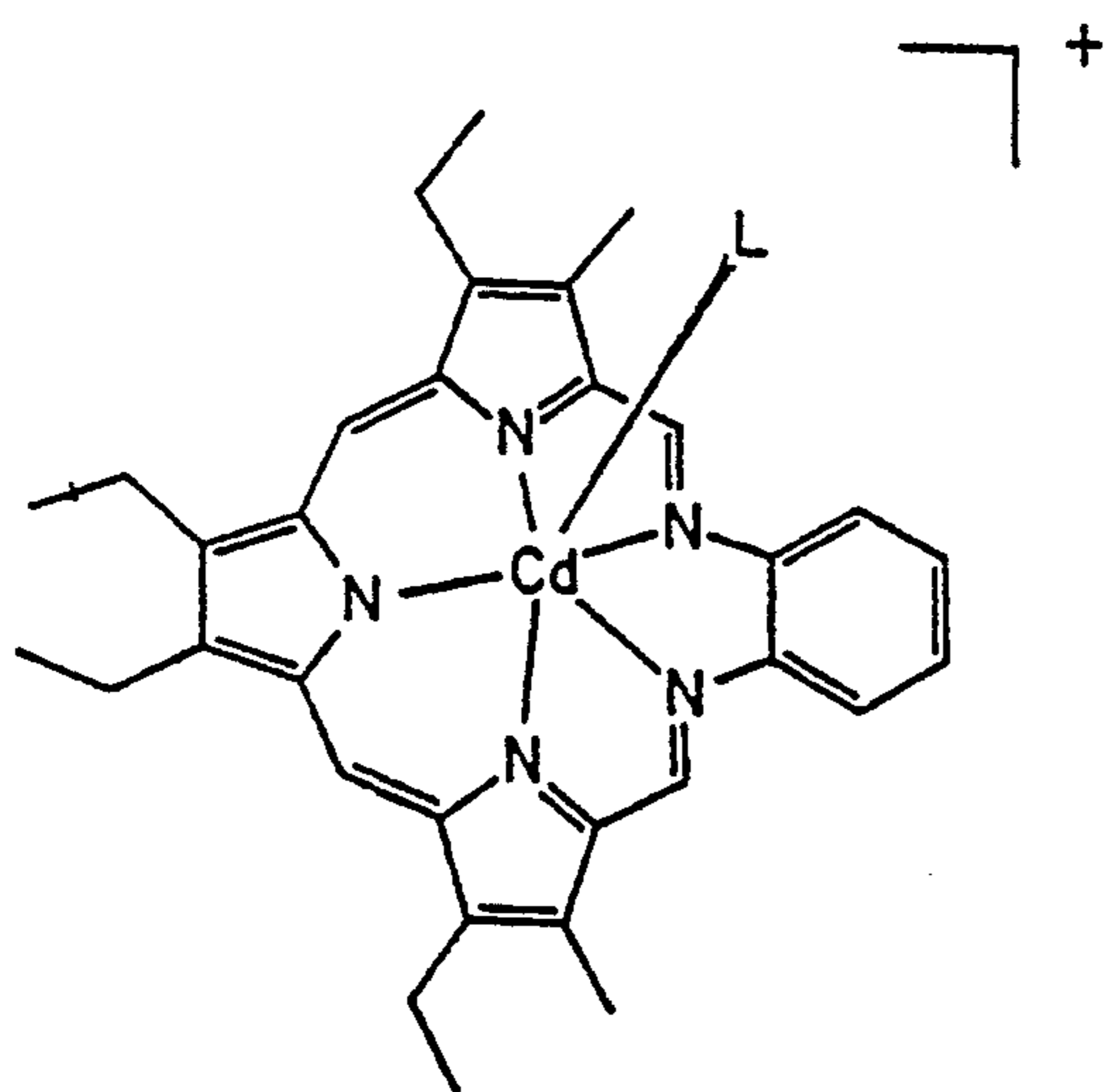
4aA. L = pyr 4bA. L = BzIm
