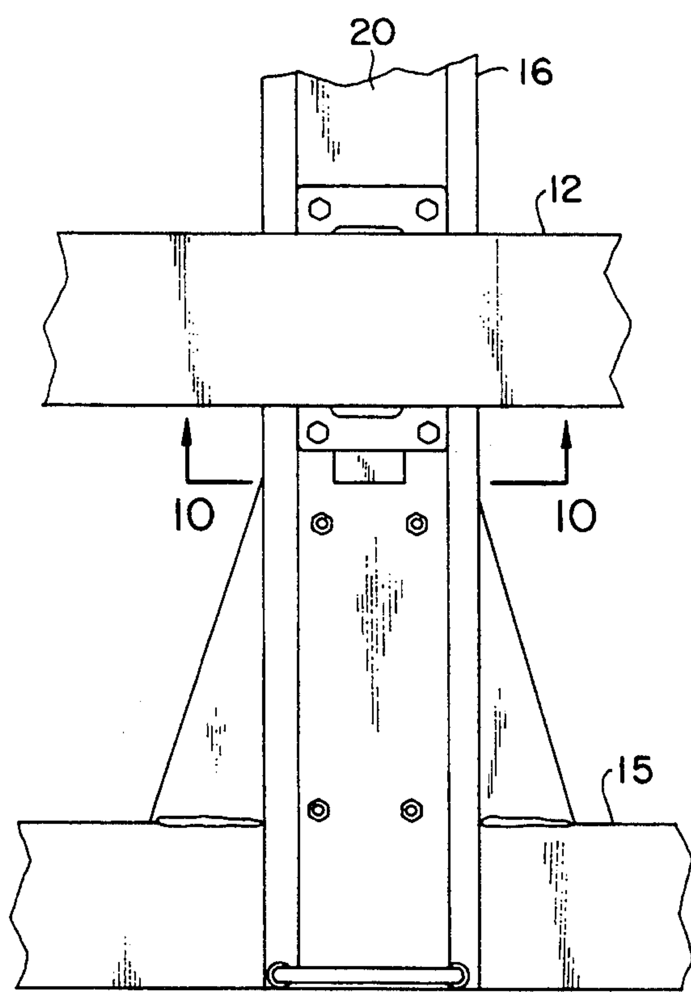
FIG. 9
