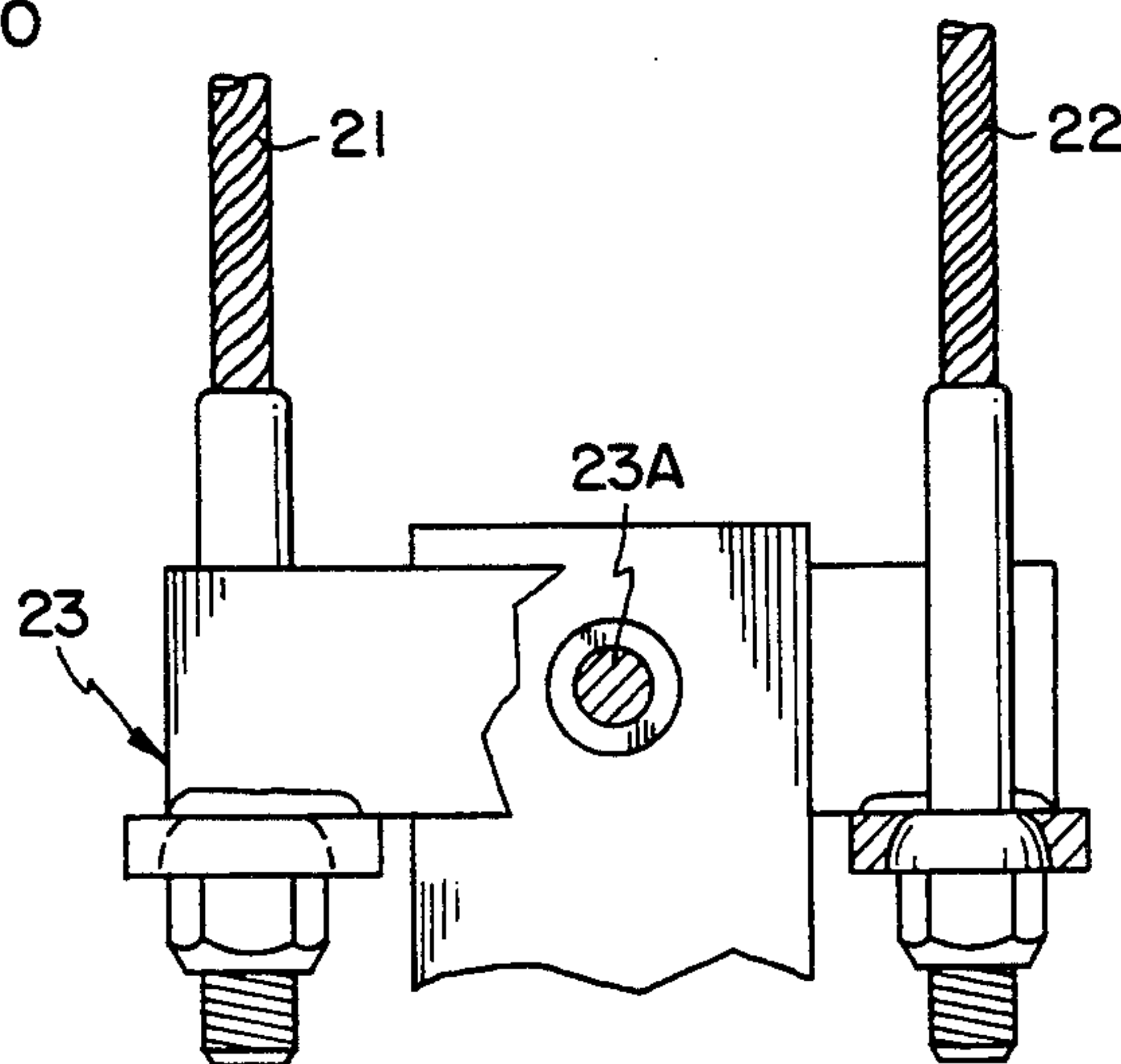
FIG. 8B
