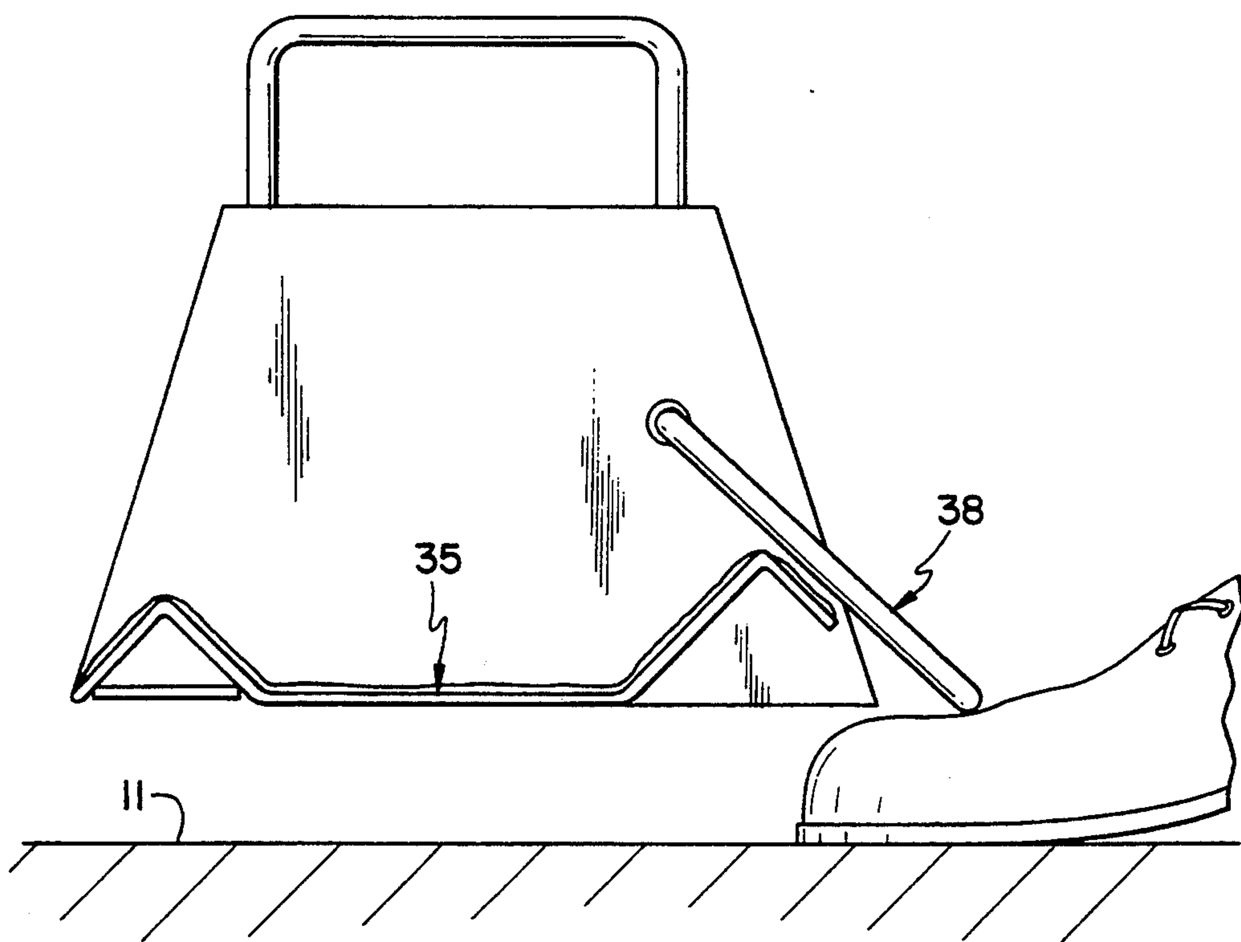
FIG. 26A
