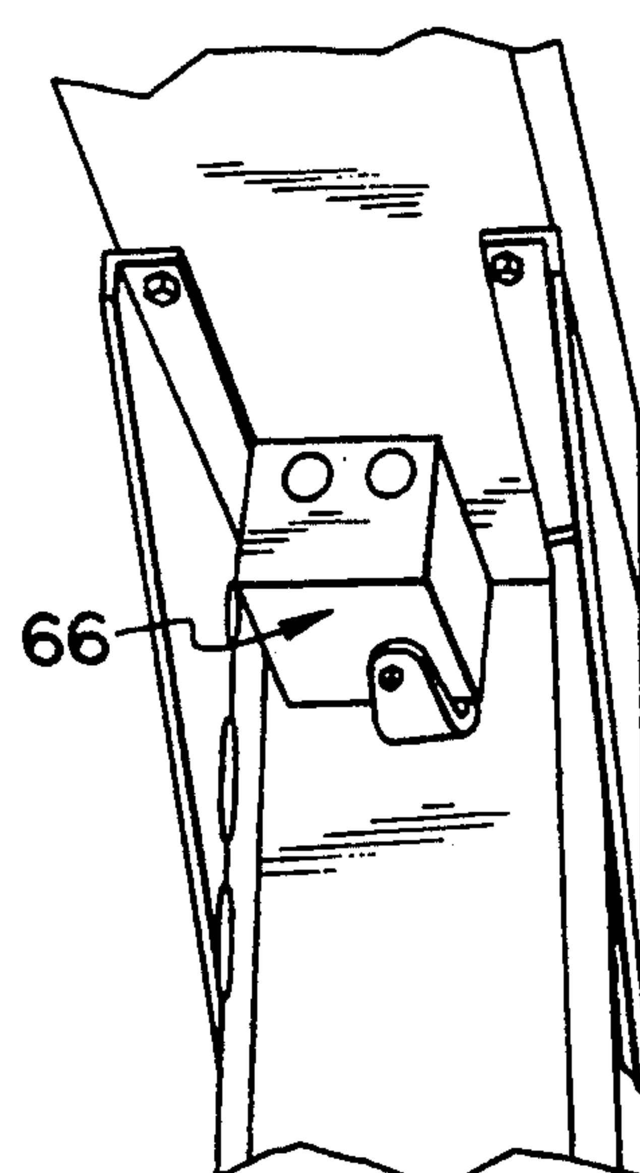
FIG. 21B
