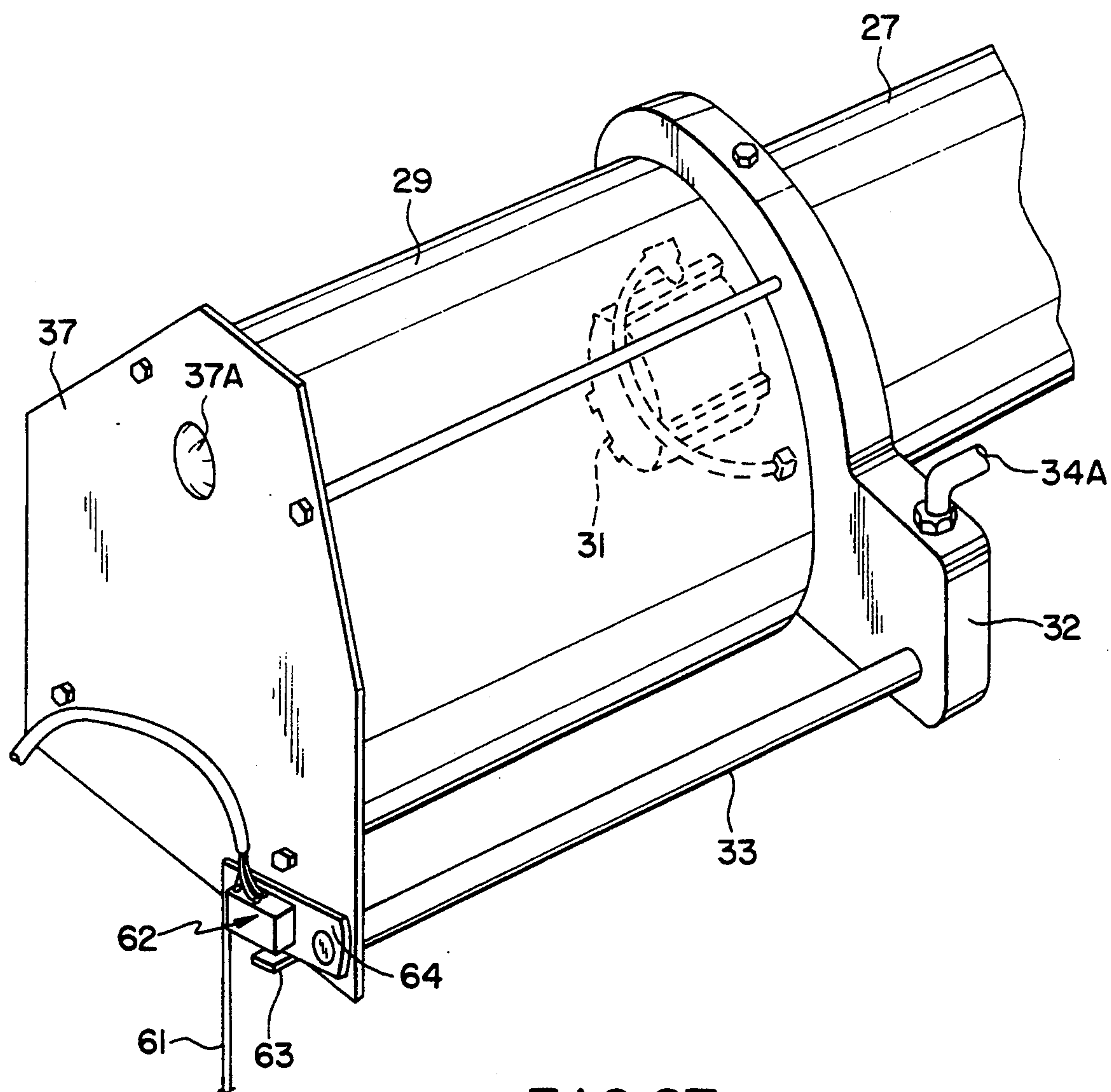
FIG. 27
