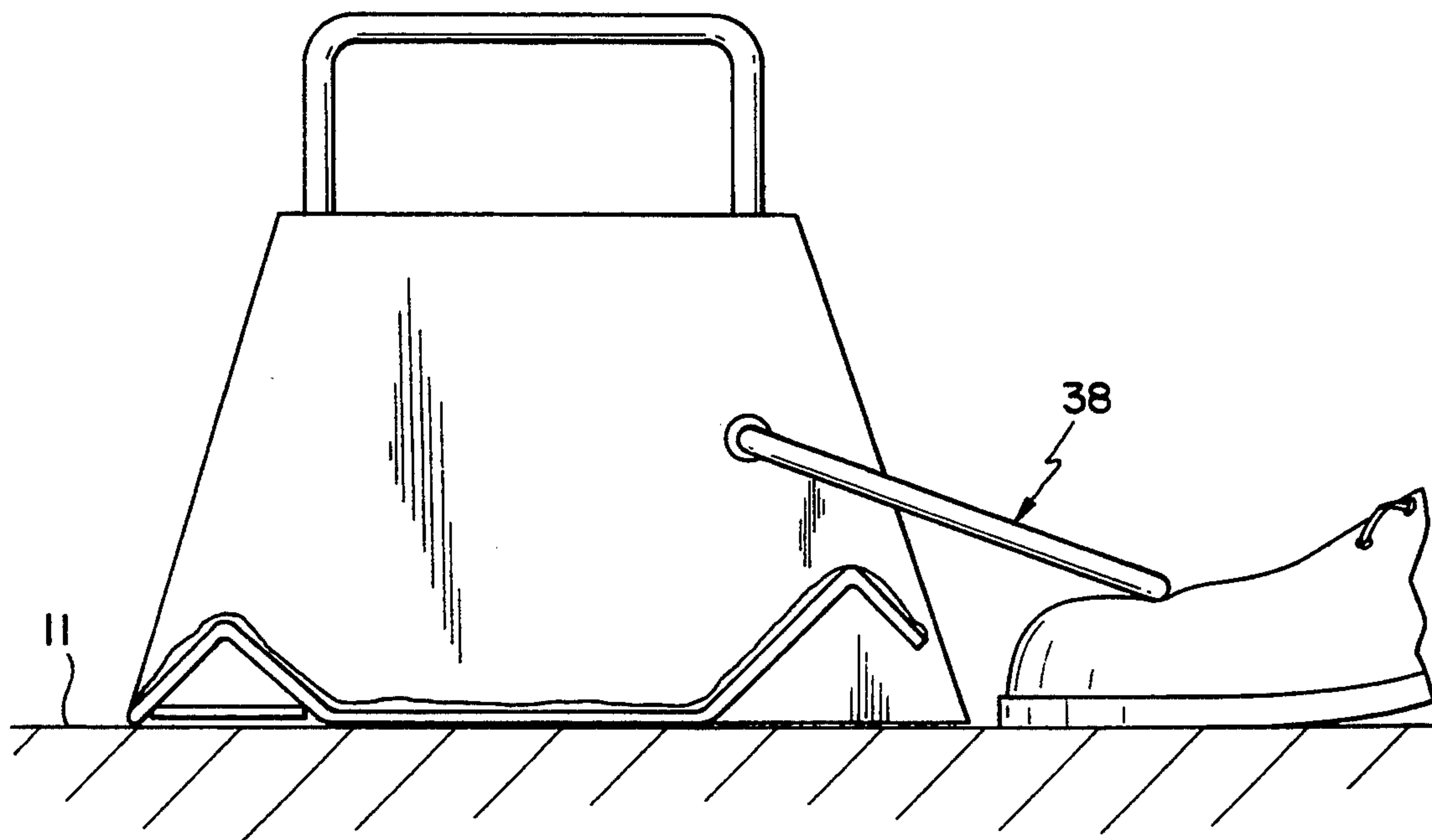
FIG. 26B
