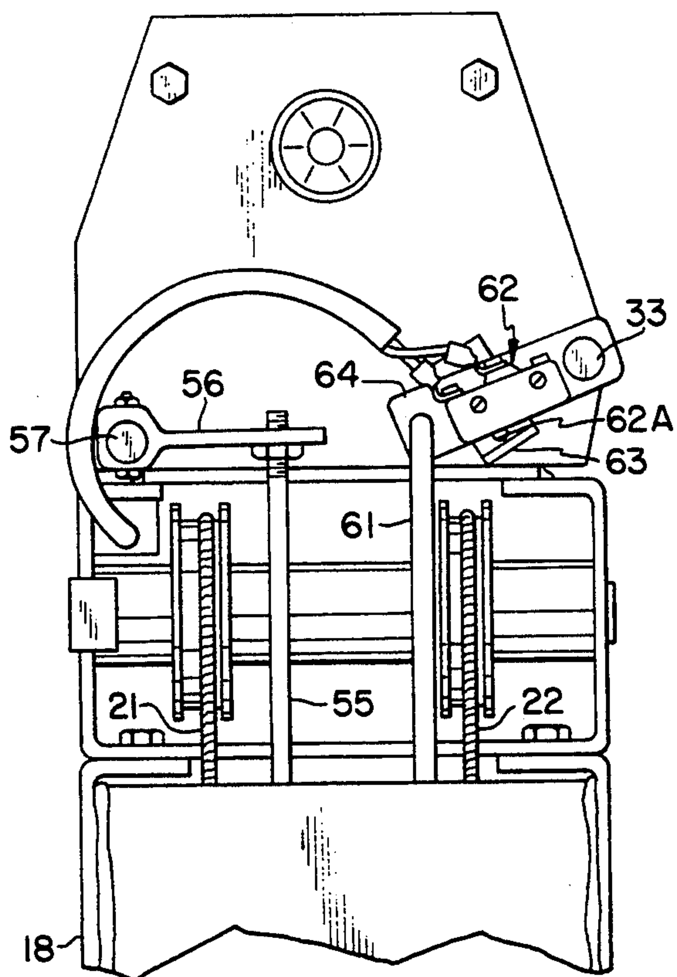
FIG. 17
