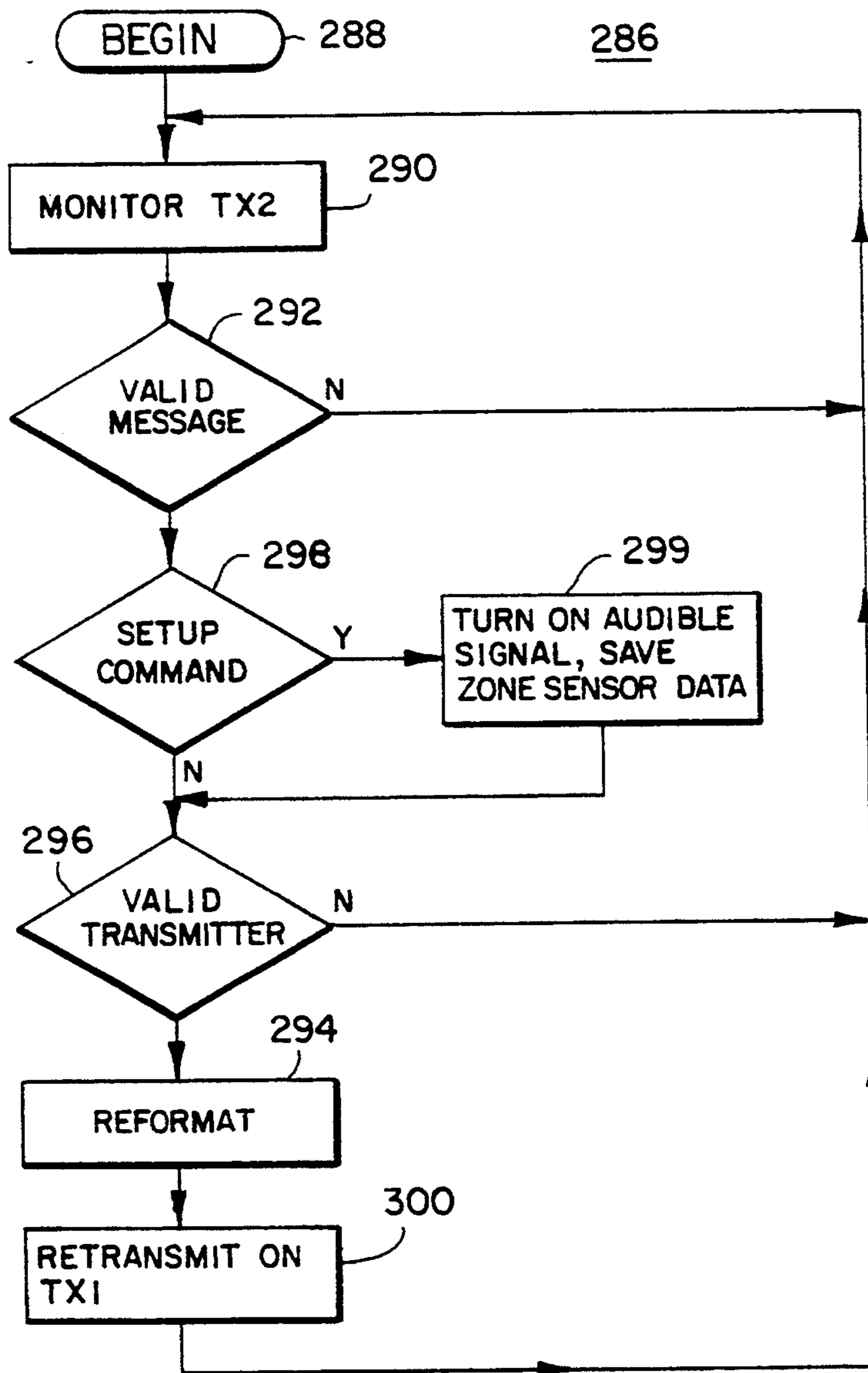
FIG. 16
