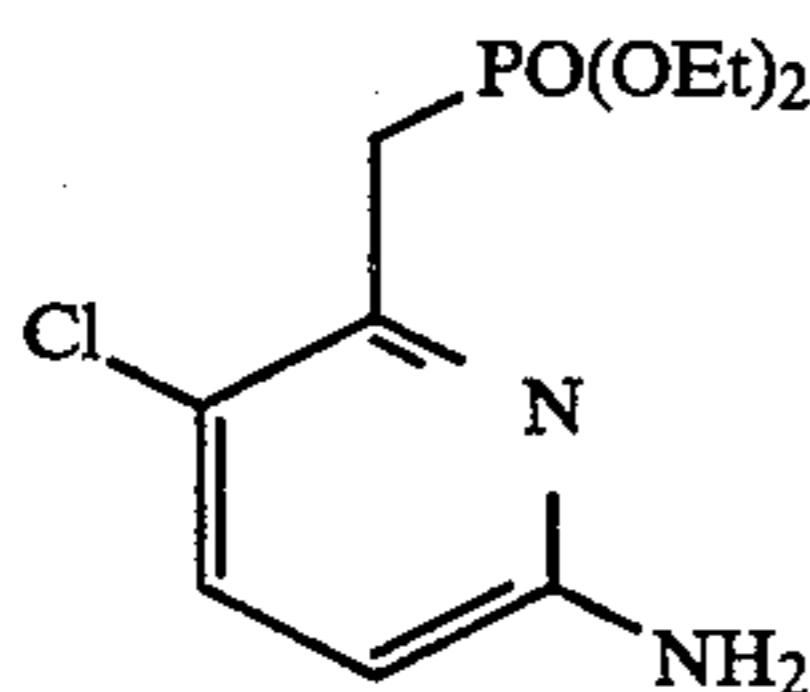
diethyl [(6-amino-3-chloro-2-pyridinyl)methyl]phosphonate
