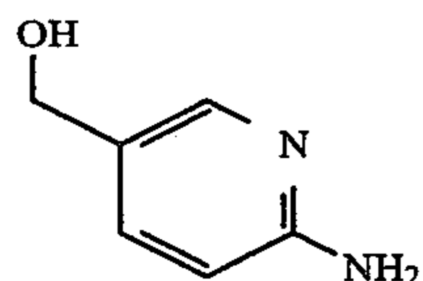
6-amino-3-pyridinemethanol
