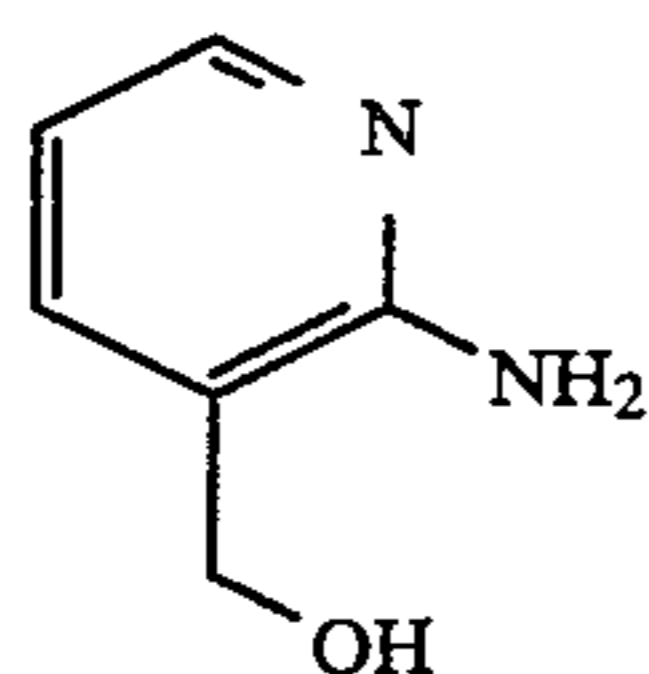
2-amino-3-(hydroxymethyl)pyridine
