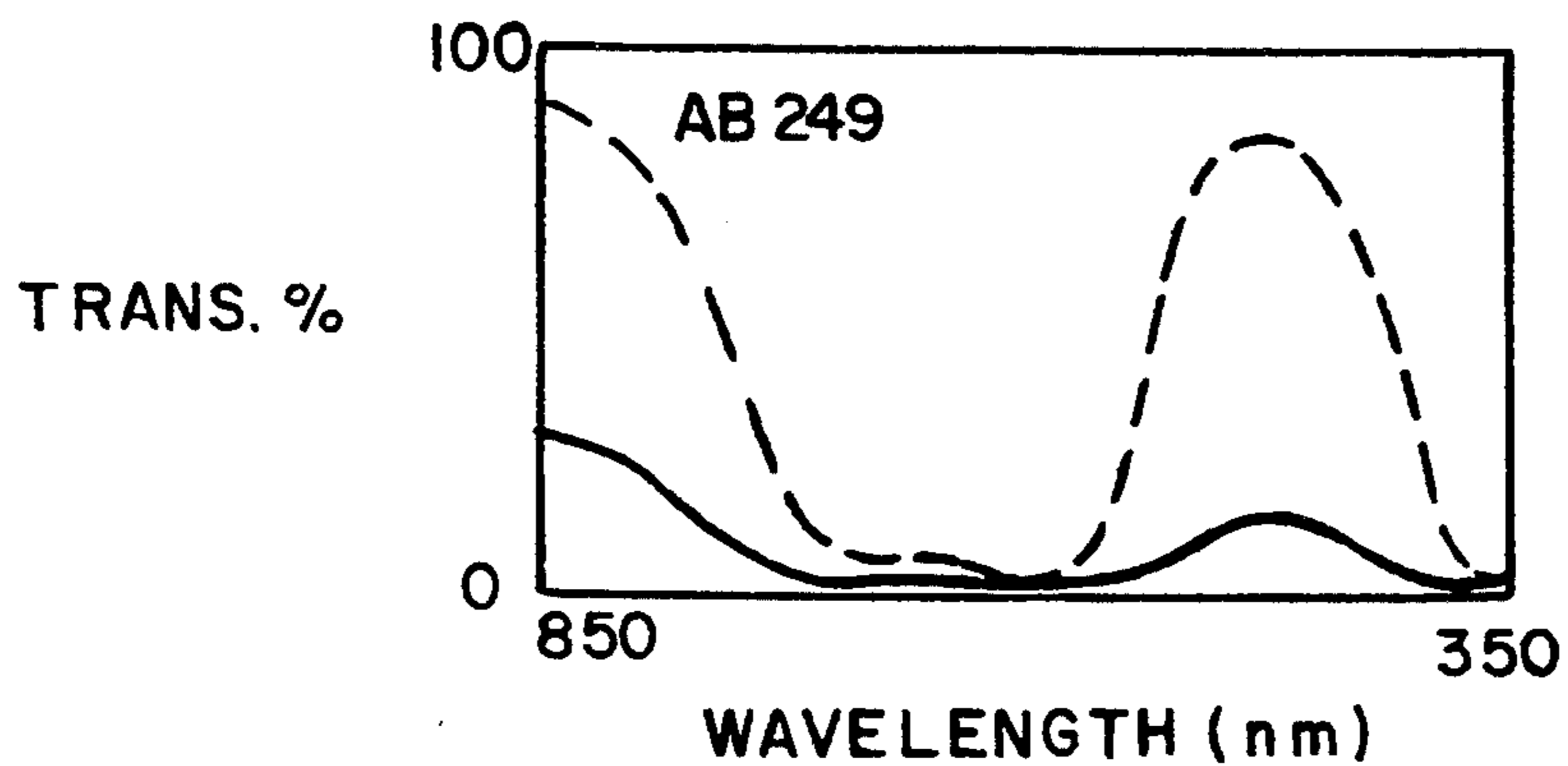
FIG. 10A
