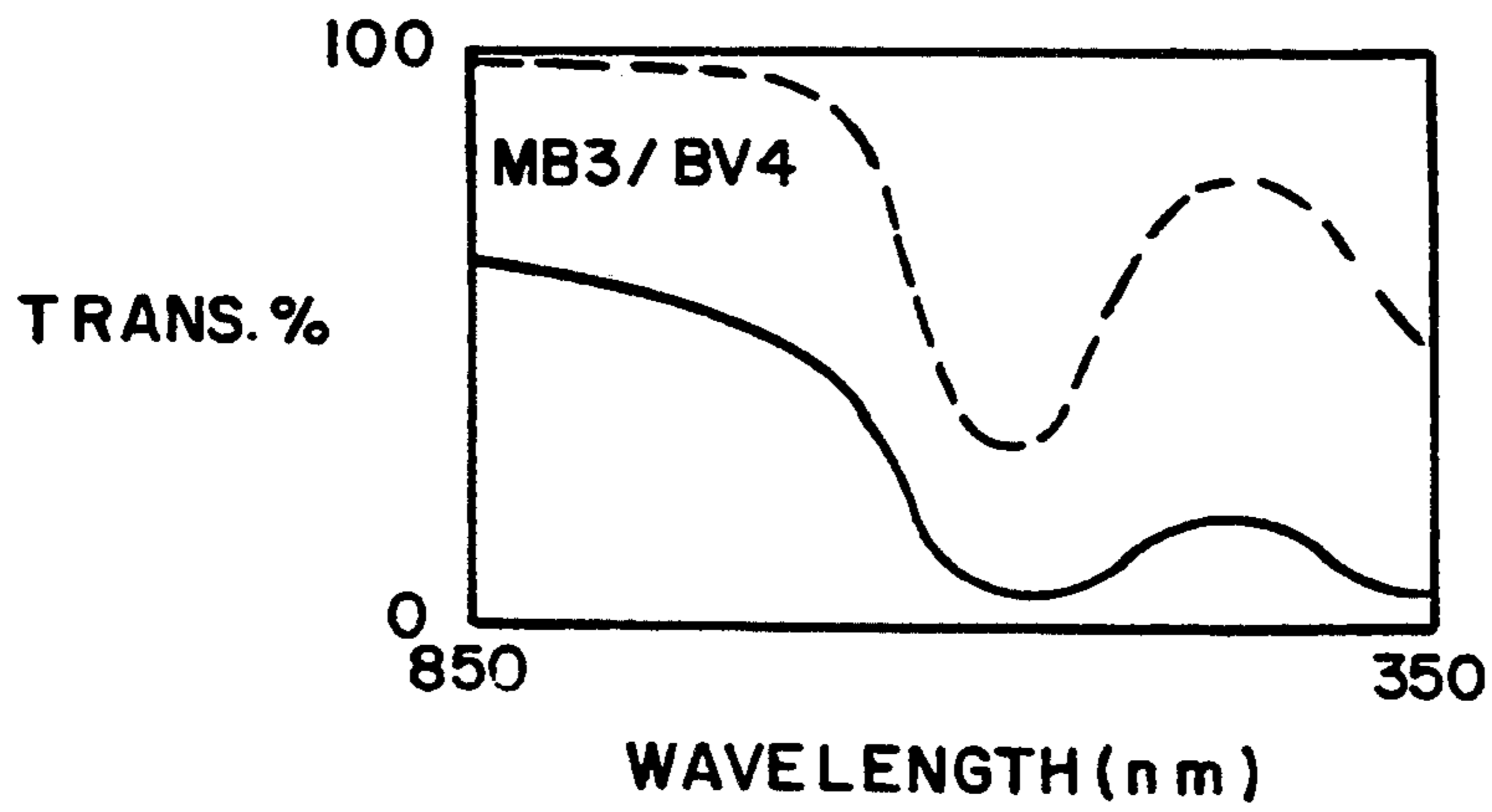
FIG. 10G
