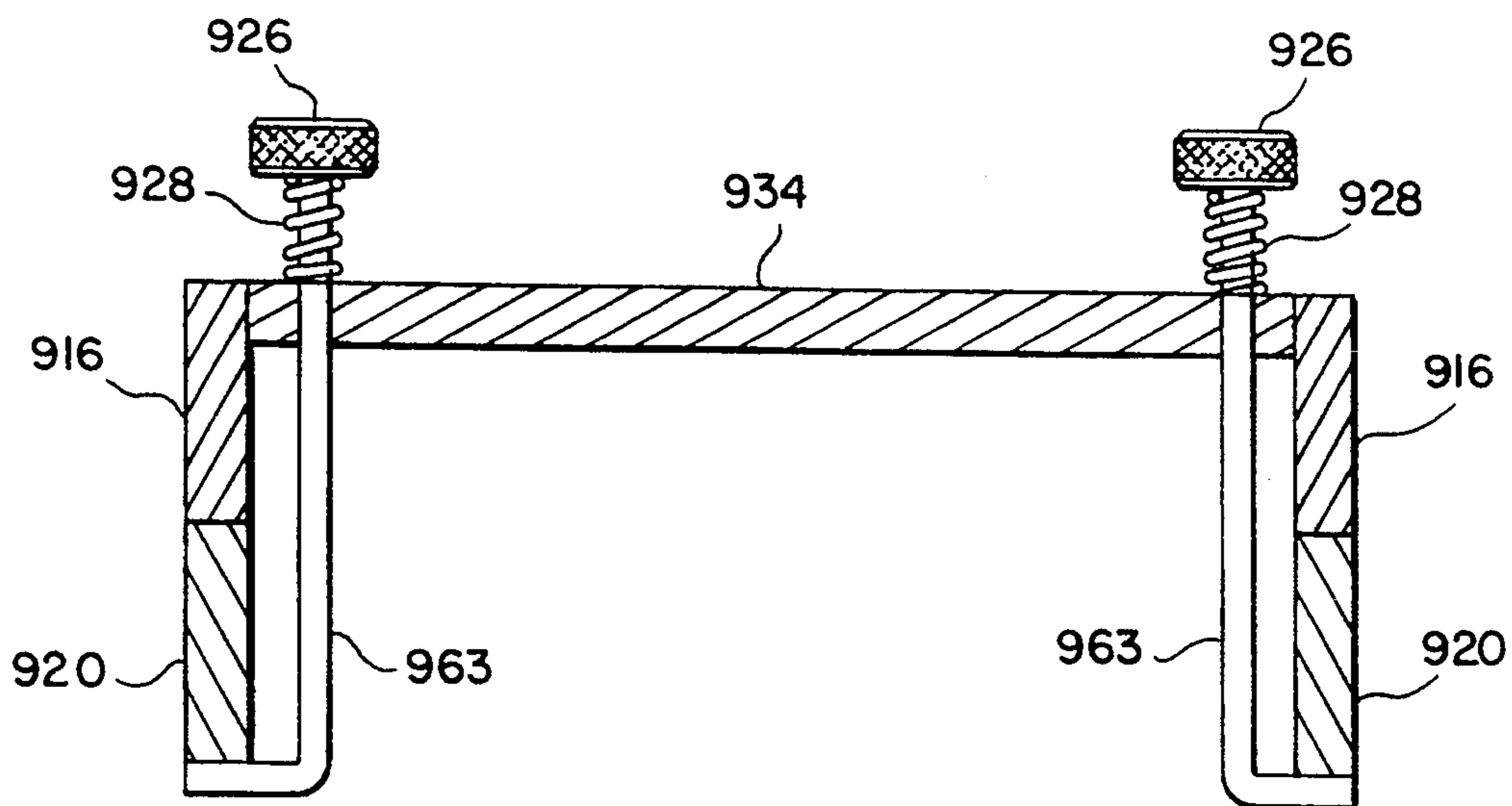
Fig. 7E SECTION "B" - "B"
