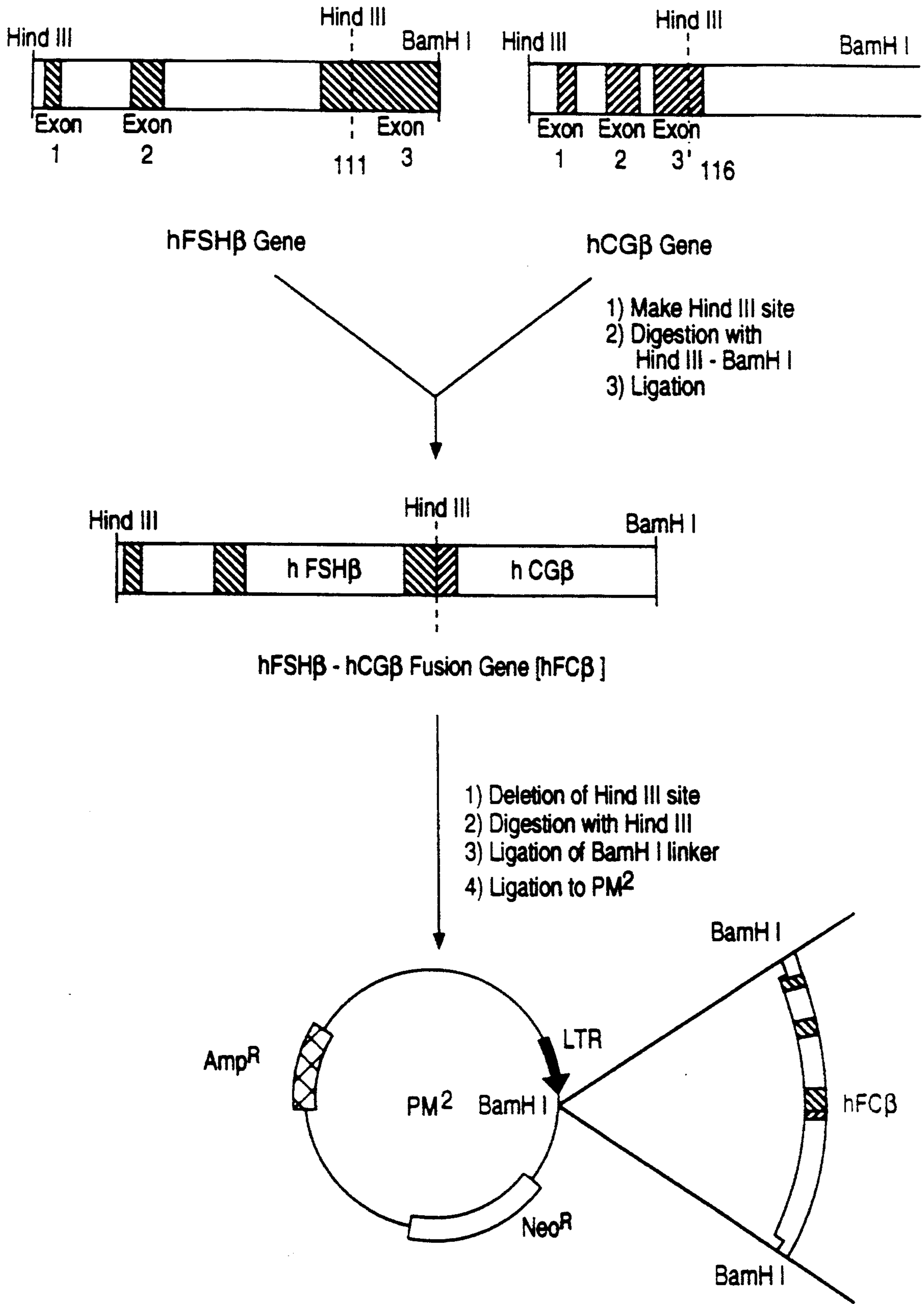
FIG. 4A
